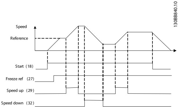
图 6.1 加速/减速
