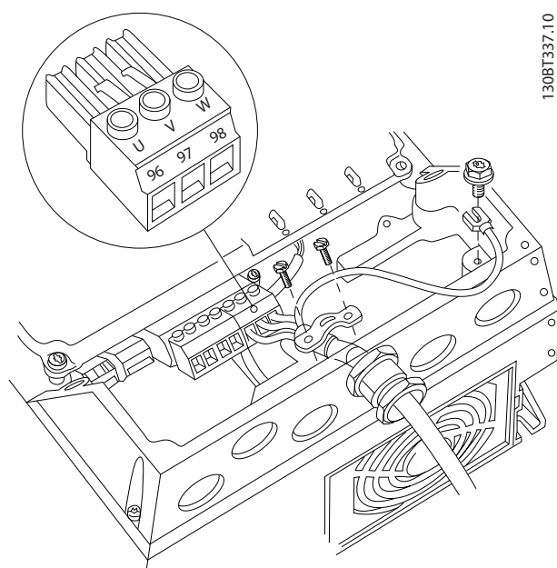
图 4.7 机箱类型 A4/A5 (IP55/66/NEMA 类型 12) 的电动机接线
