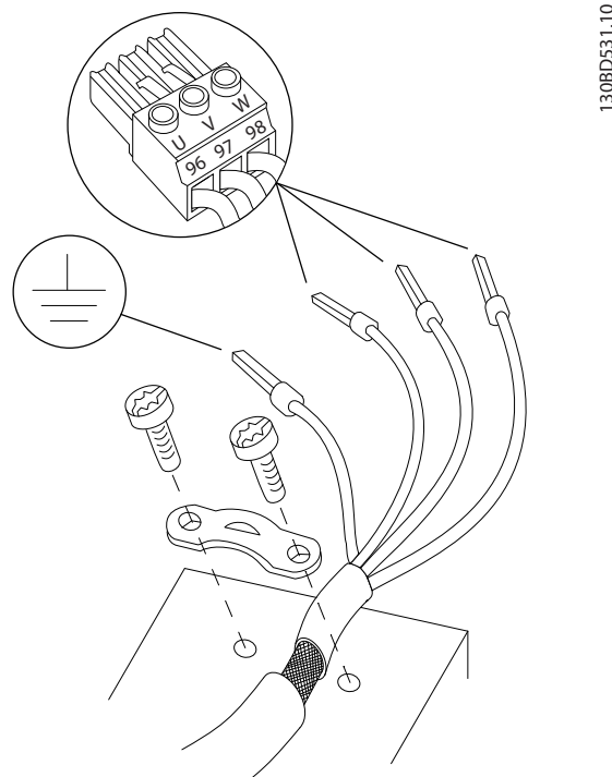
图 4.5 电机连接
