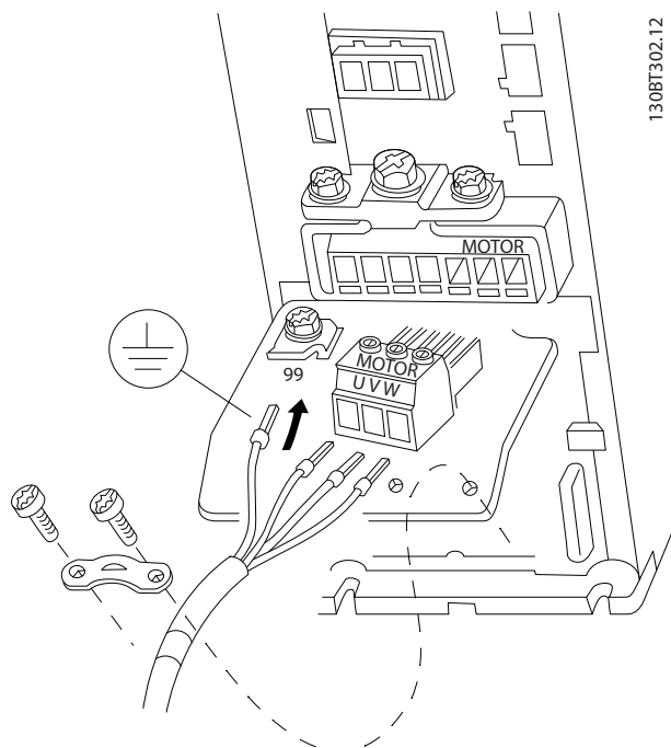
图 4.6 机箱类型 A2 和 A3 的电动机接线
