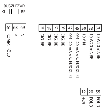
Illusztráció 24: Vezérlőcsatlakozók
