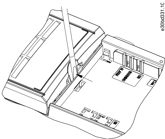
Illusztráció 23: A csatlakozóburkolat eltávolítása
