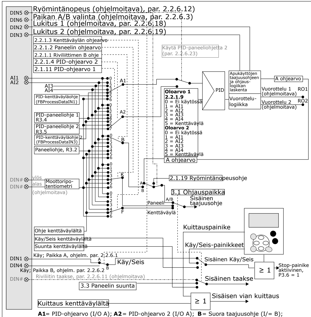
Kuva 23: Pumppu- ja puhallinsovelluksen ohjaussignaalilogiikka
