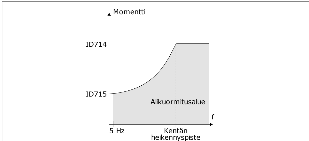
Kuva 76: Minimikuormituksen asetus
