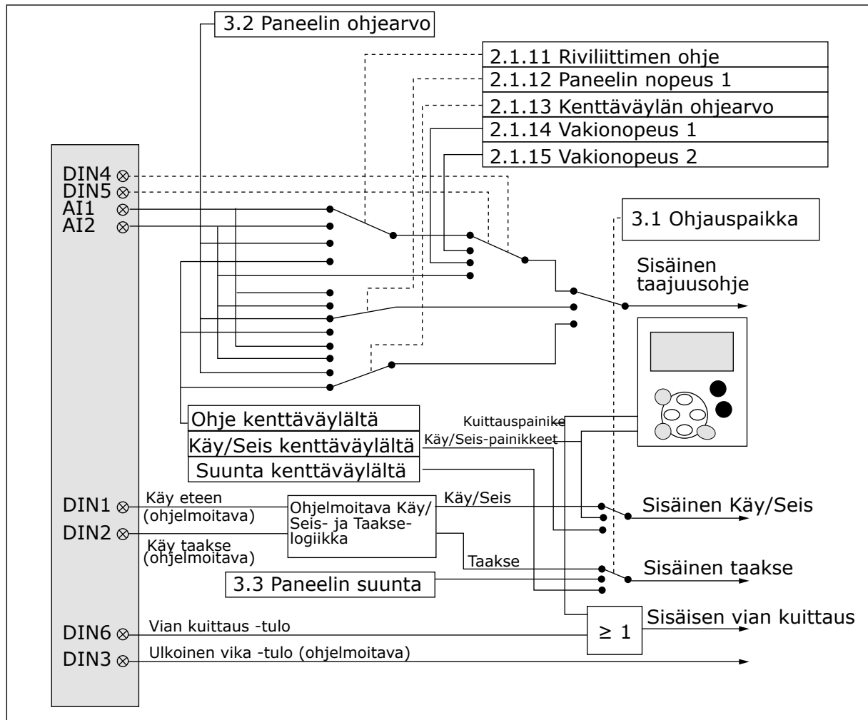
Kuva 6: Vakiosovelluksen ohjaussignaali logiikka
