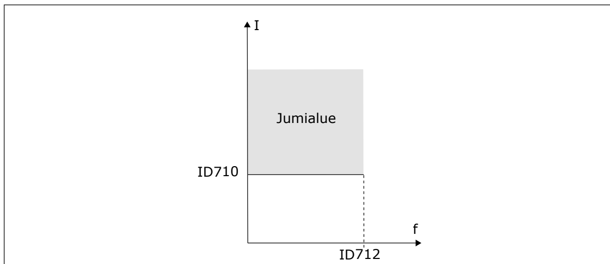
Kuva 74: Jumisuojaus asetukset
