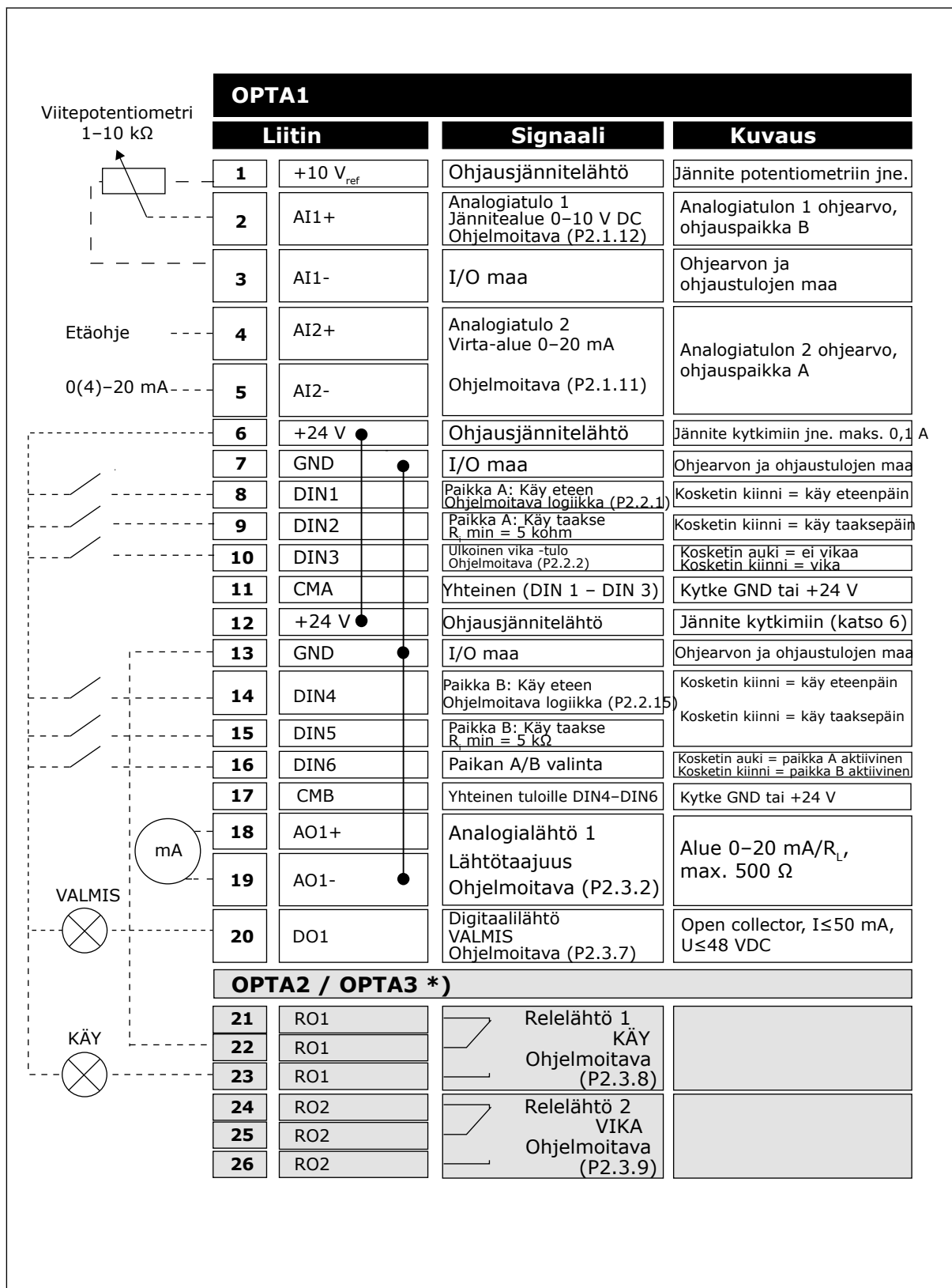
Kuva 7: Paikallis-/etäohjaussovelluksen tulojen ja lähtöjen oletusasetukset
