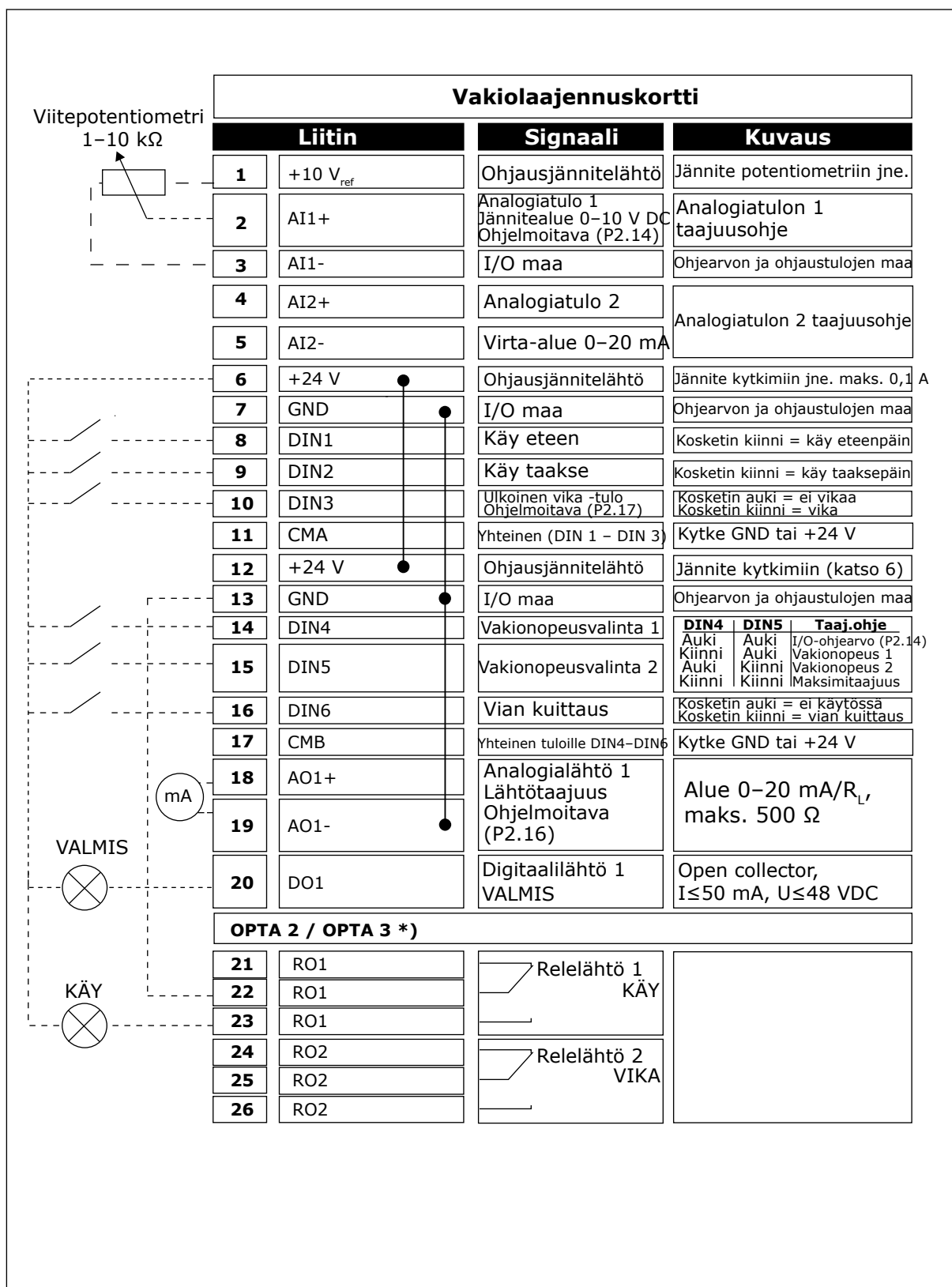
Kuva 1: Perussovelluksen tulojen ja lähtöjen oletusasetukset
