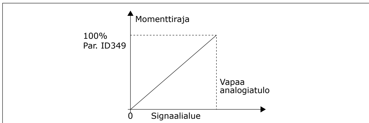
Kuva 53: Momentin valvontarajan alentaminen
