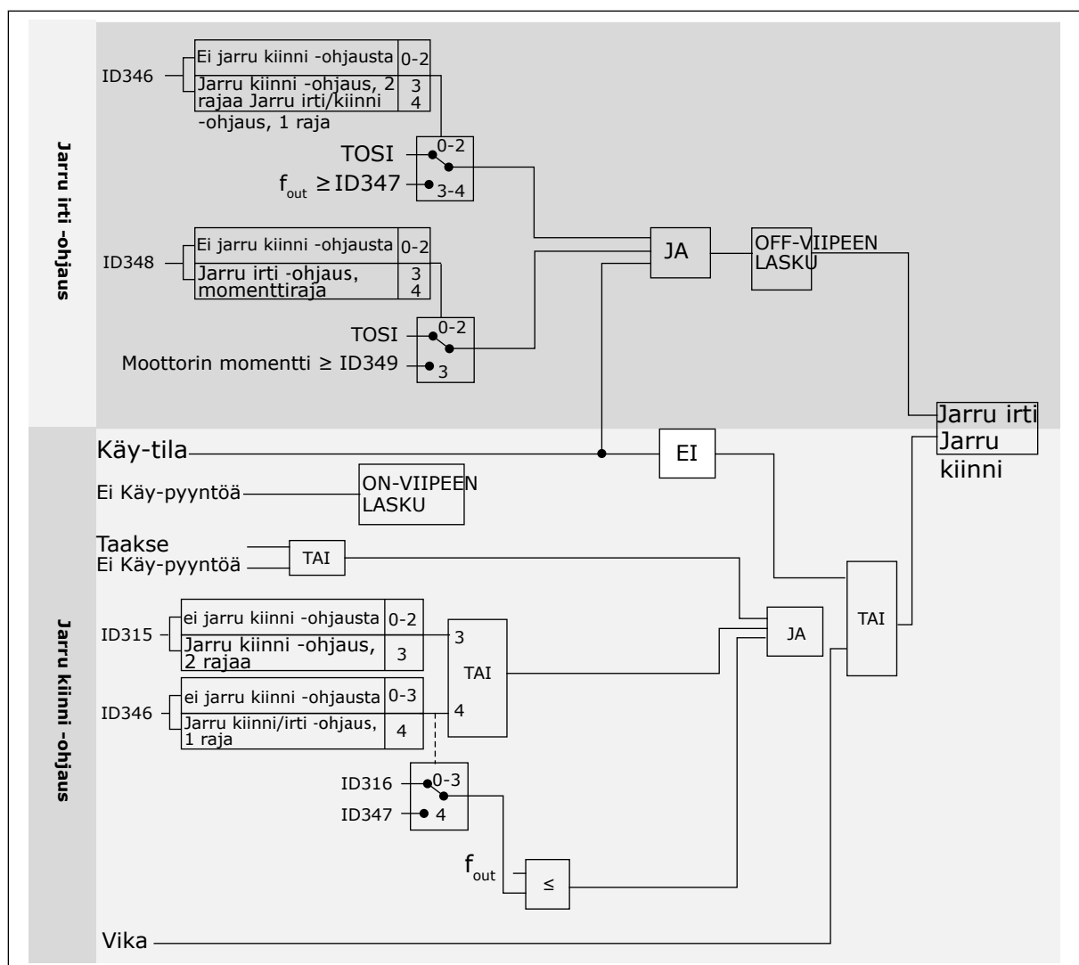
Kuva 93: Jarrun ohjauslogiikka
