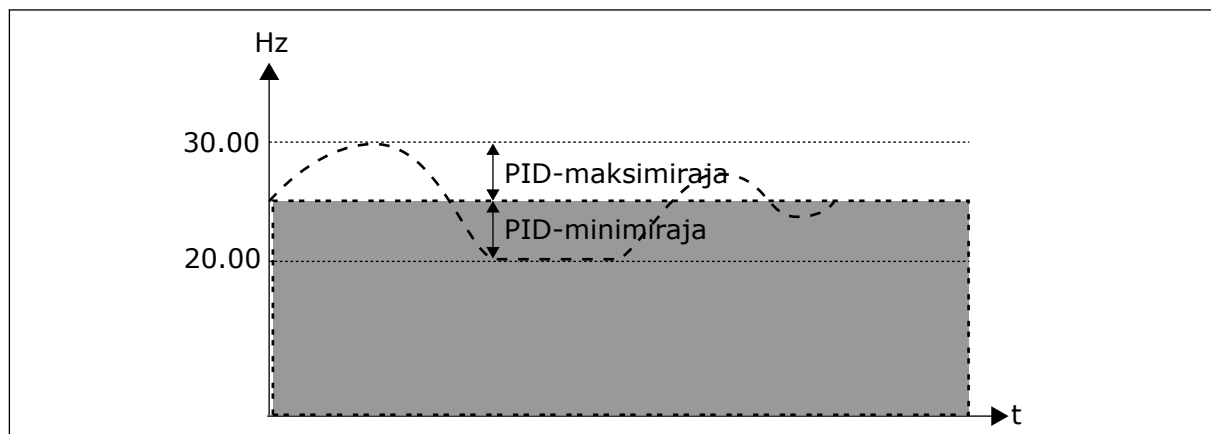
Kuva 57: PID-summapisteen ohjearvo
