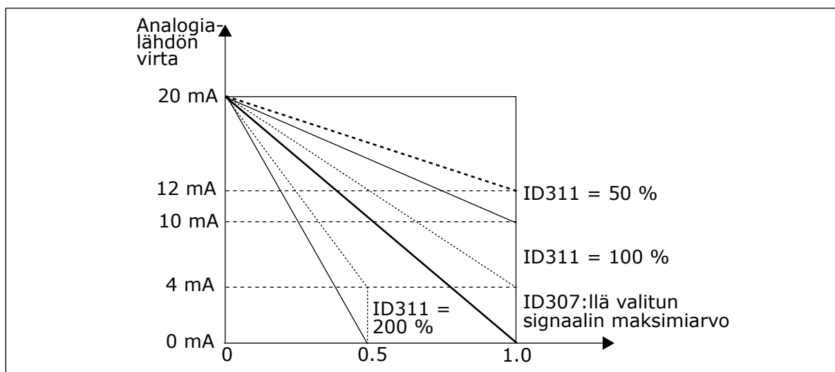
Kuva 38: Analogialähdön kääntö
