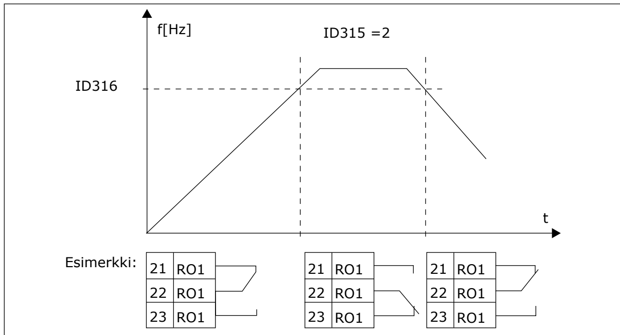
Kuva 40: Lähtötaajuuden valvonta
