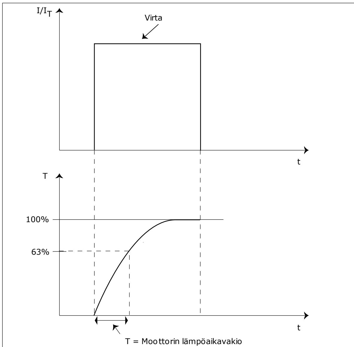
Kuva 73: Moottorin lämpöaikavakio
