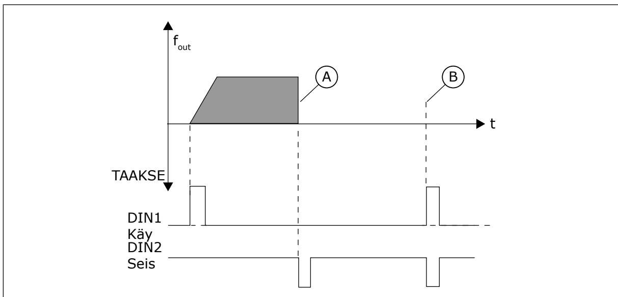
Kuva 32: Käy-pulssi/Seis-pulssi
