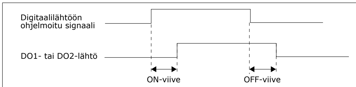
Kuva 65: Digitaallähtöjen 1 ja 2 ON- ja OFF-viiveet
