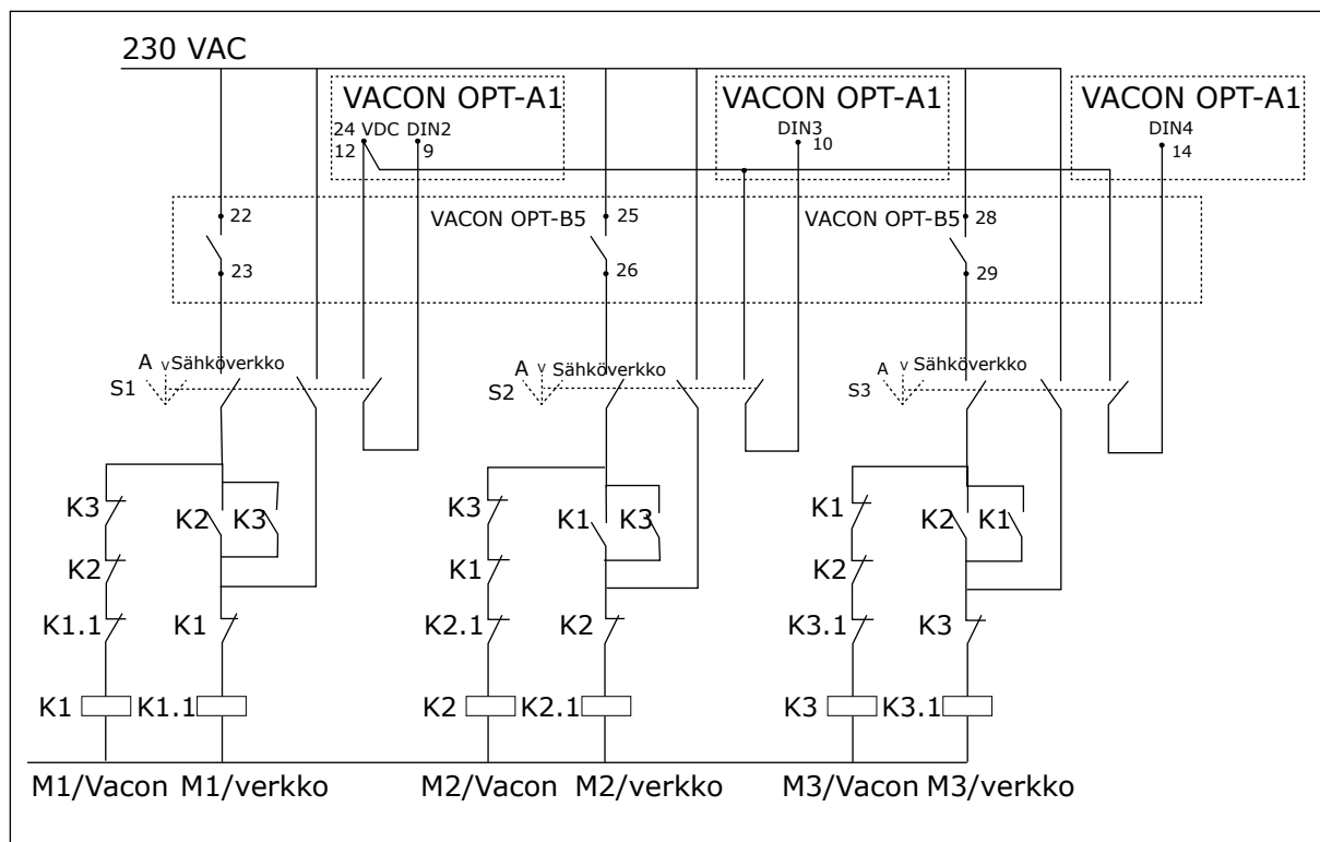
Kuva 22: Pumppujen vuorottelujärjestelmä, ensisijainen ohjauskaavio
