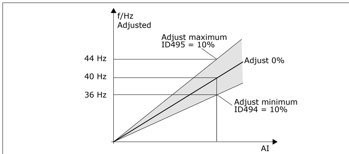
Kuva 66: Esimerkki säätötulosta
