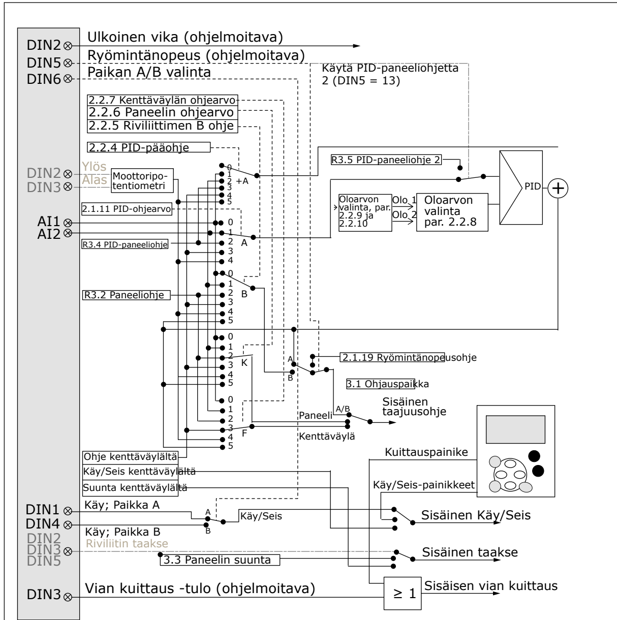
Kuva 15: PID-säätösovelluksen ohjaussignaaliologiikka
