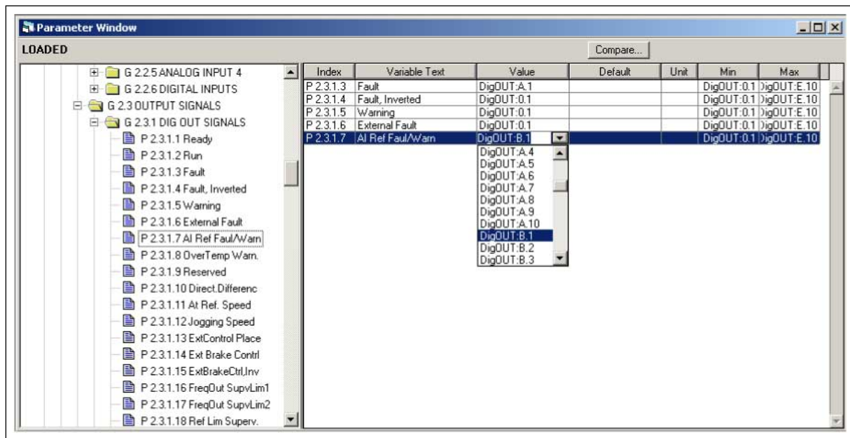
Kuva 95: NCDrive-ohjelmointityökalun näyttökuva; osoitekoodin syöttäminen
