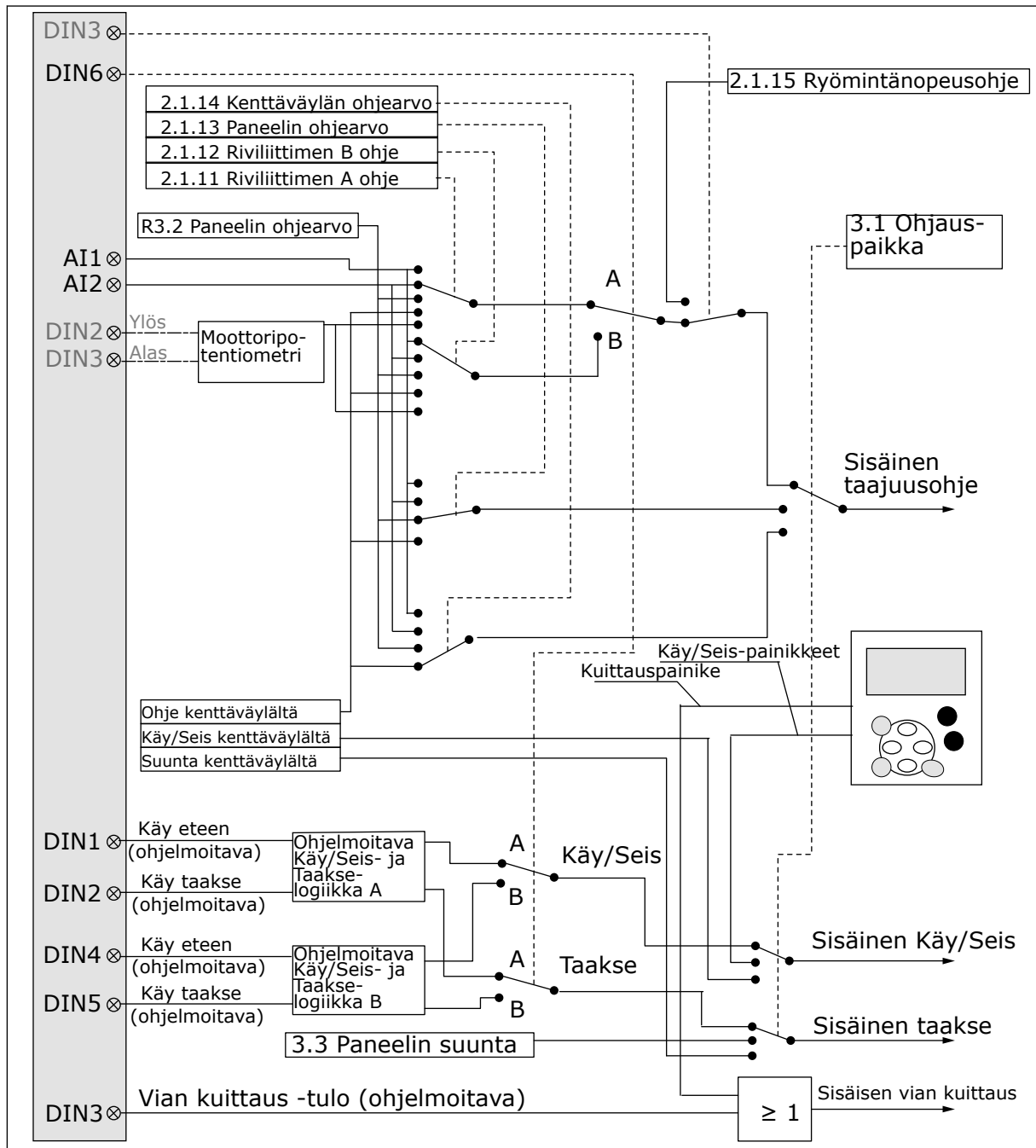
Kuva 9: Paikallis-/etäohjaussovelluksen ohjaussignaaliologia
