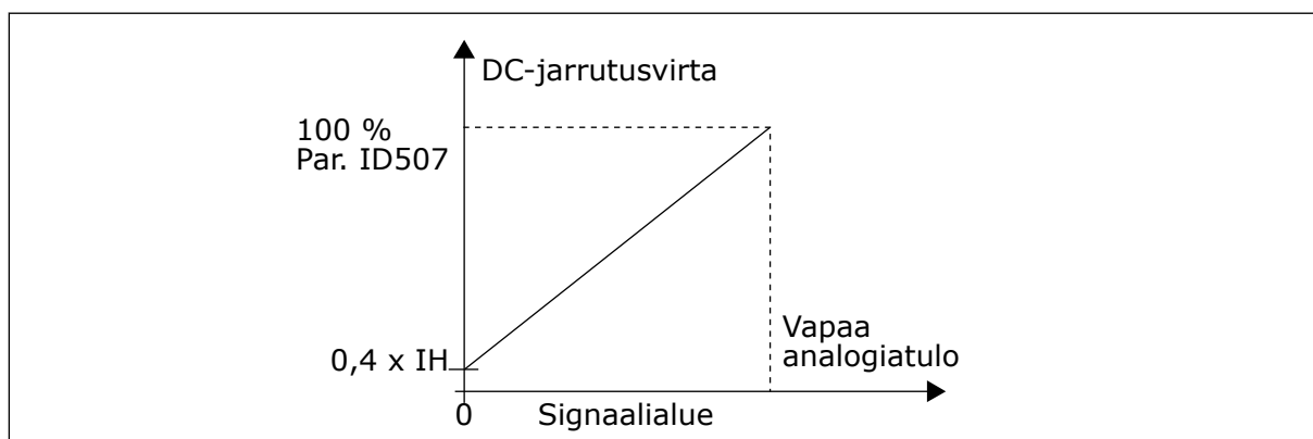
Kuva 51: DC-jarrutusvirran pienentäminen
