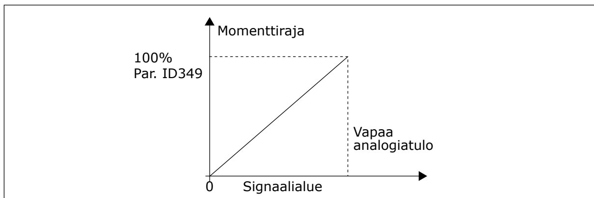
Kuva 64: Moottorin momenttirajan skaalaus
