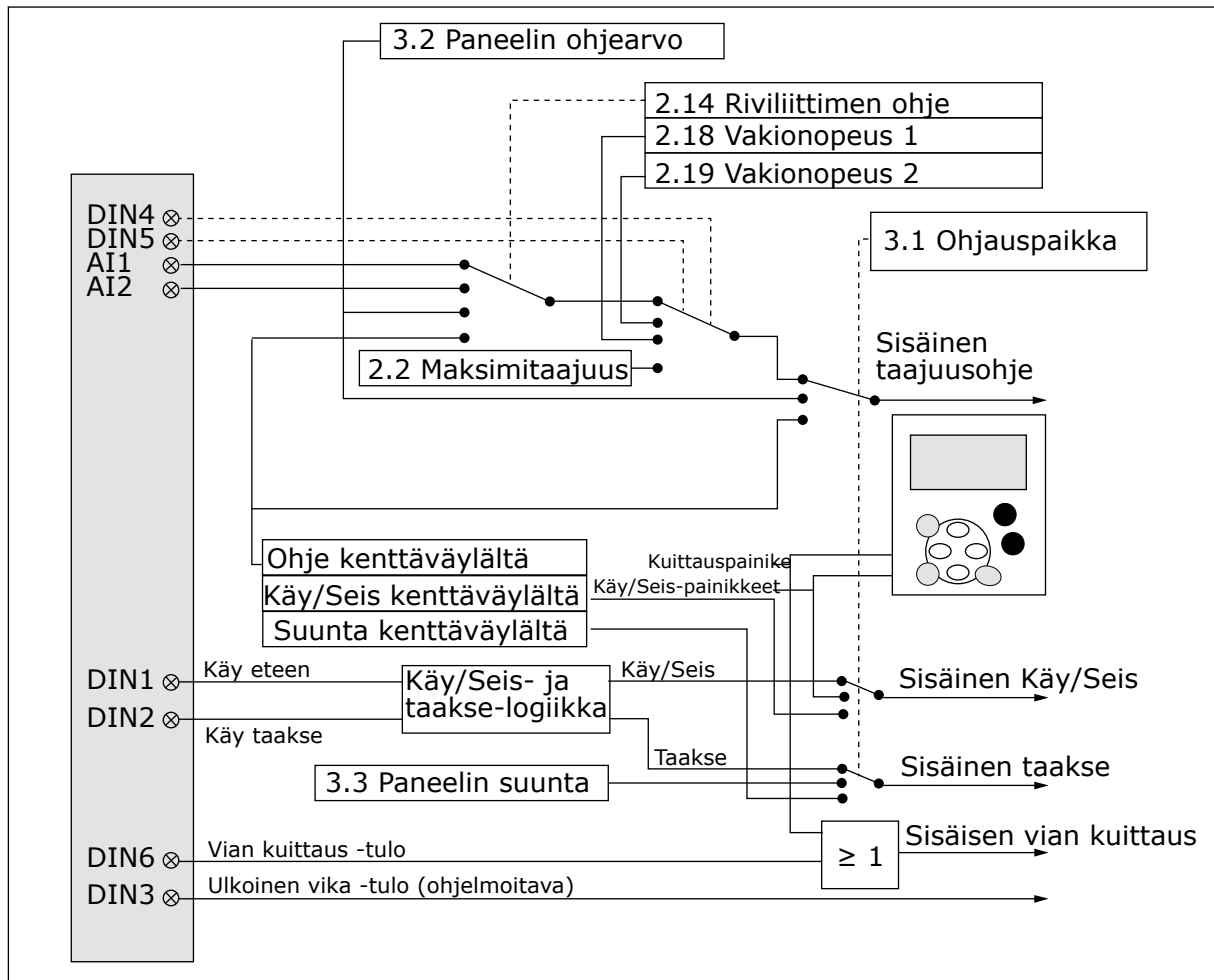
Kuva 3: Perussovelluksen ohjaussignaaliologiikka
