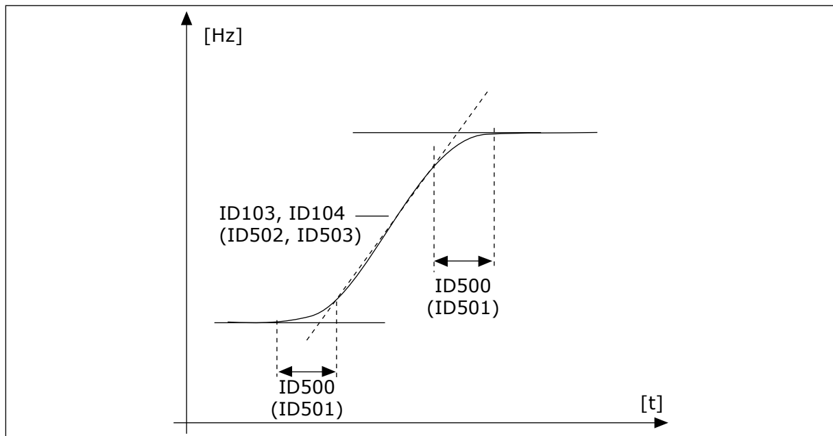
Kuva 67: Kiihtyvyyden-/hidastuvuuskäyrä (S-muoto)
