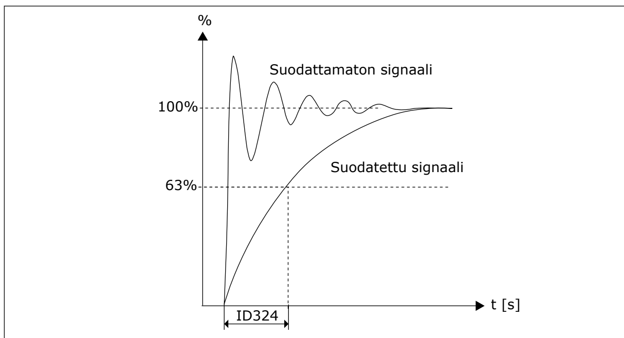
Kuva 44: AI1-signaalin suodatus.
