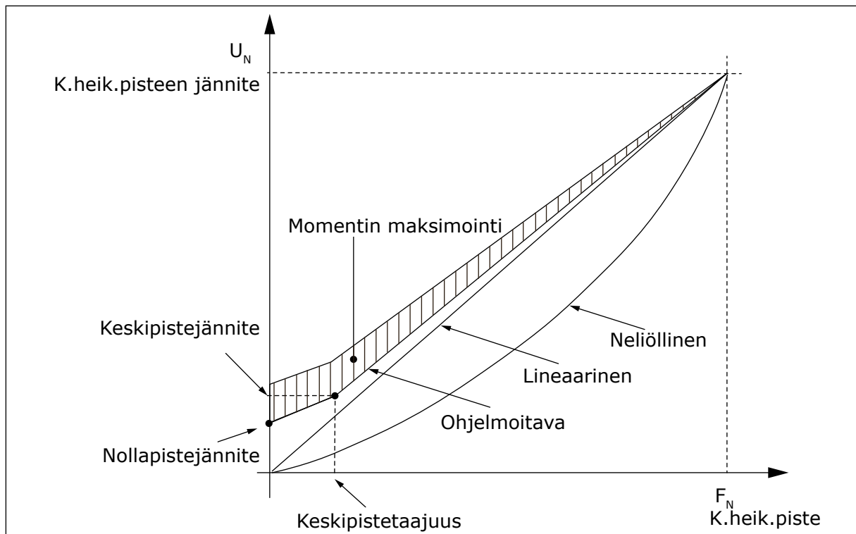
Kuva 26: U/f-optimointi
