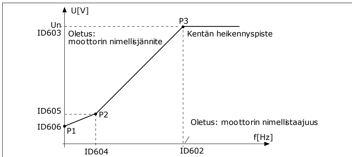
Kuva 25: Ohjelmoitava U/f-käyrä
