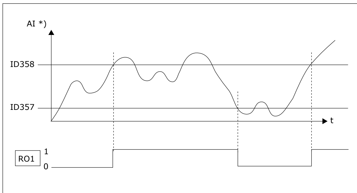
Kuva 49: Esimerkki päälle/pois-ohjauksesta
