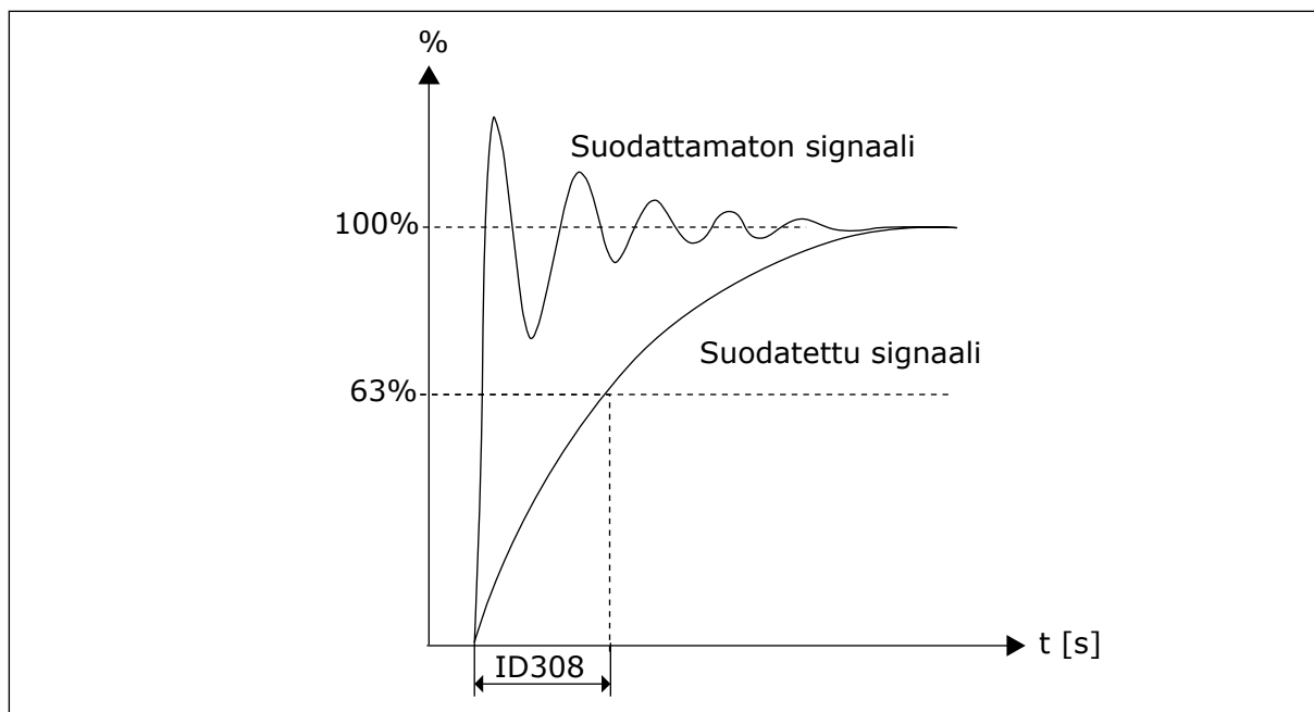
Kuva 37: Analogialähdön suodatus
