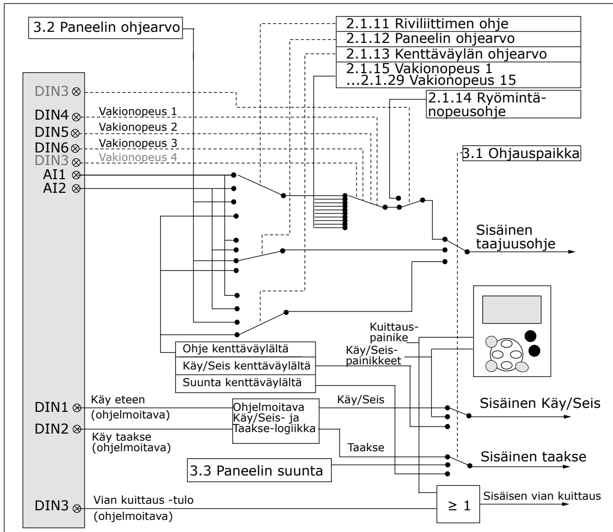
Kuva 12: Multi-Step-nopeussovelluksen ohjaussignaalilogiikka
