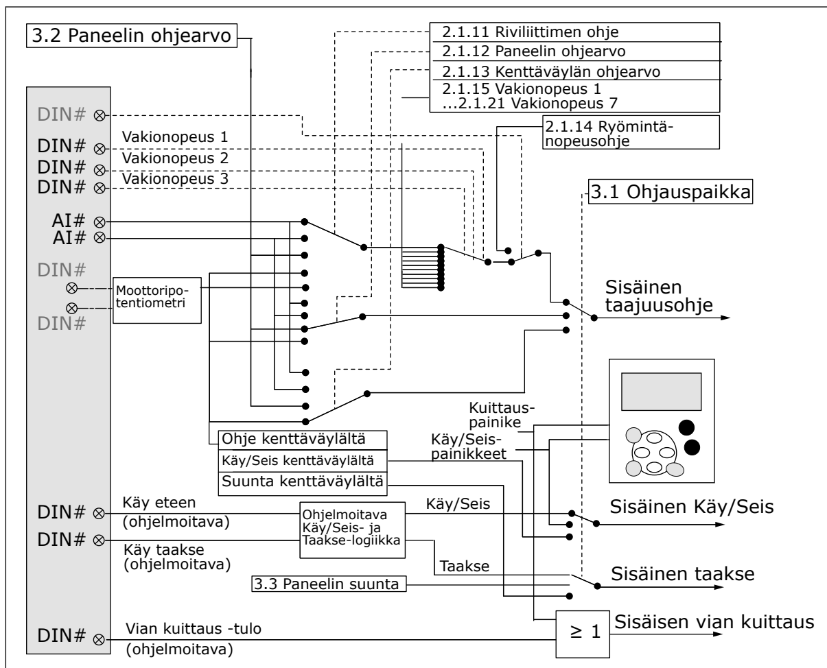
Kuva 18: Erikoiskäyttösovelluksen ohjaussignaaliologiikka
