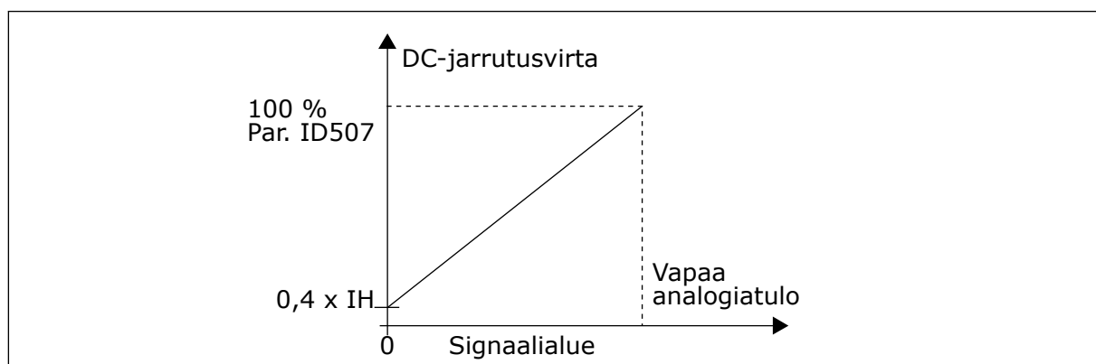
Kuva 61: DC-jarrutusvirran skaalaus
