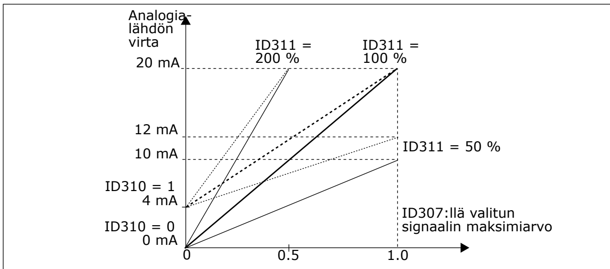
Kuva 39: Analogilähdön skaalaus
