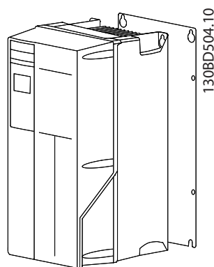
圖 3.3 使用背板的正確安裝
