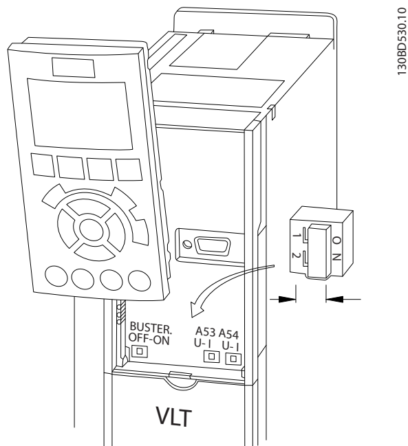
圖 4.13 端子 53 和 54 開關的位置
