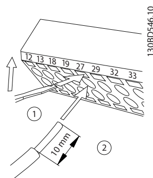
圖 4.12 連接控制線路
