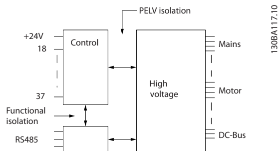
圖 8.1 PELV 絕緣
