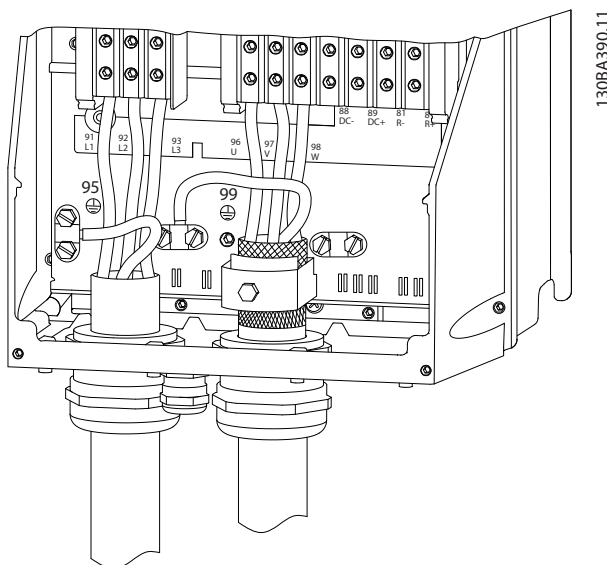
圖 4.8 使用遮罩電纜線外殼類型 B 和 C 的馬達、主電源與接地配線
