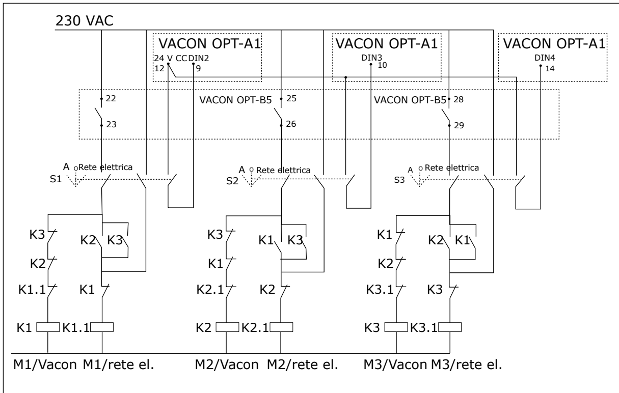
Fig. 22: Sistema di rotazione ausiliari pompa, schema dei collegamenti
