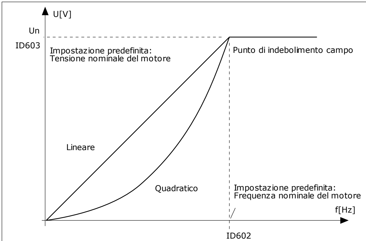
Fig. 24: variazione lineare e quadratica della tensione del motore
