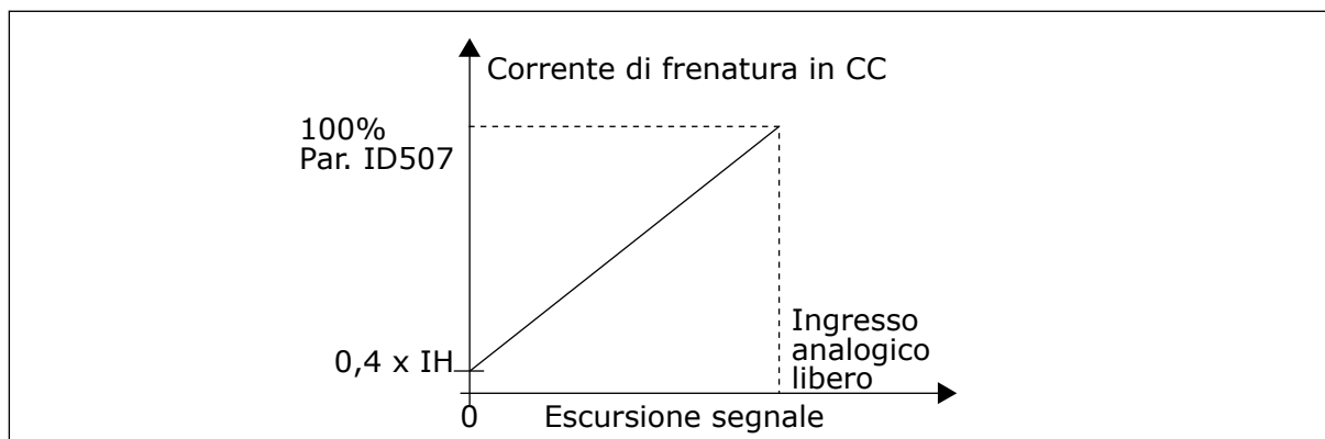
Fig. 61: Scalatura corrente di frenatura in CC
