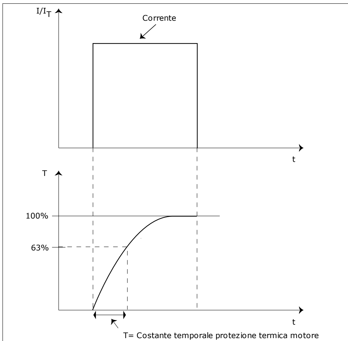
Fig. 73: la costante temporale per la protezione termica del motore
