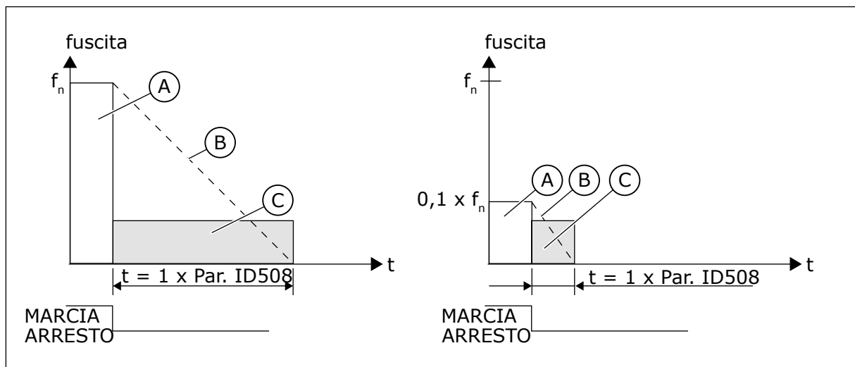
Fig. 68: Tempo di frenatura in CC nella funzione Arresto = Arresto per inerzia
