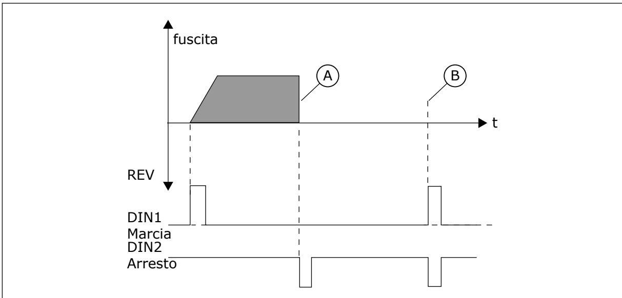
Fig. 32: Impulso di marcia/Impulso di arresto
