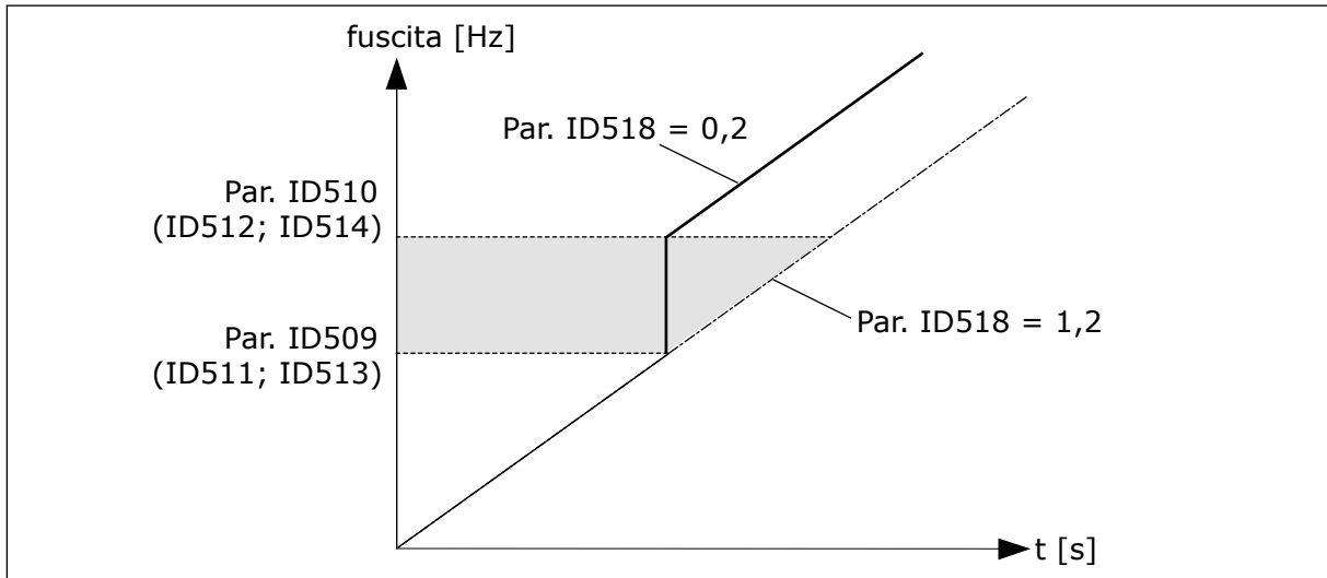
Fig. 71: Multiplicazione del tempo di rampa tra le frequenze proibite
