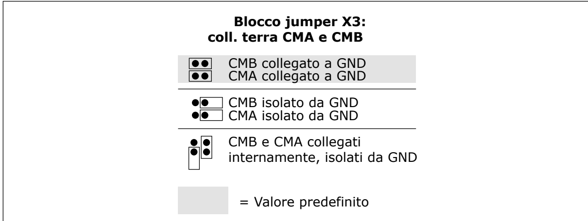
Fig. 2: Selezioni jumper
