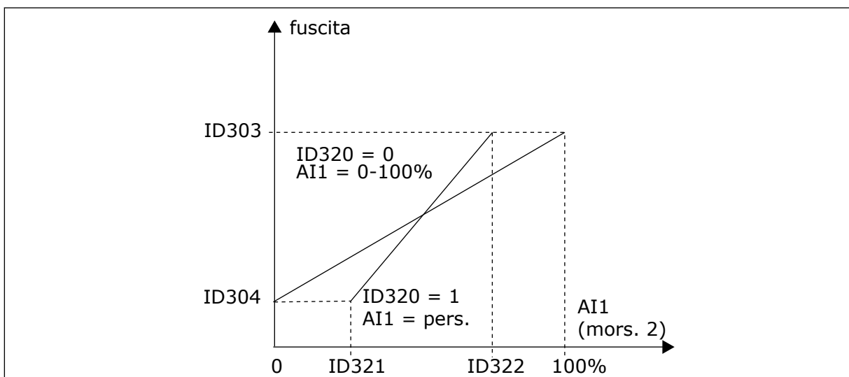
Fig. 42: Nessuna inversione del segnale AI1
