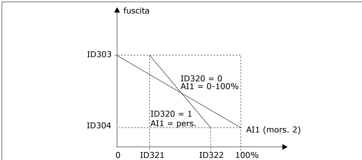
Fig. 43: Inversione segnale AI1
