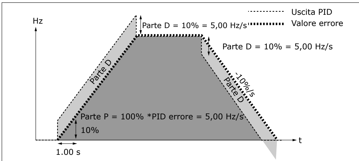
Fig. 29: Uscita PID con i valori dell'esempio 3
