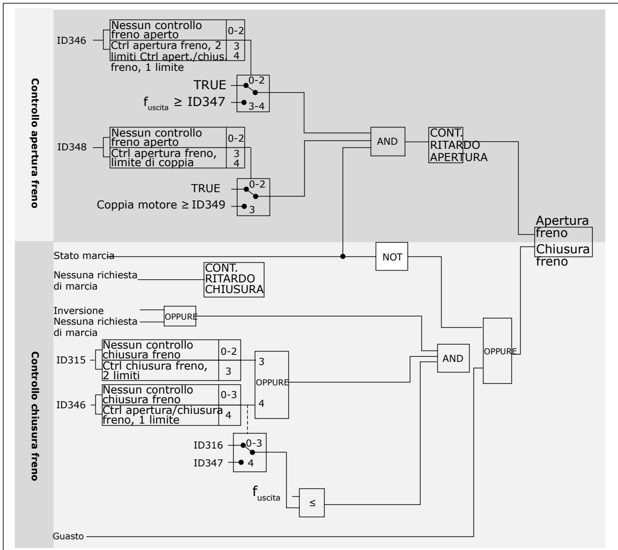
Fig. 93: Logica di controllo del freno
