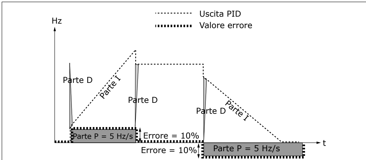
Fig. 28: Curva uscita PID con i valori dell'esempio 2
