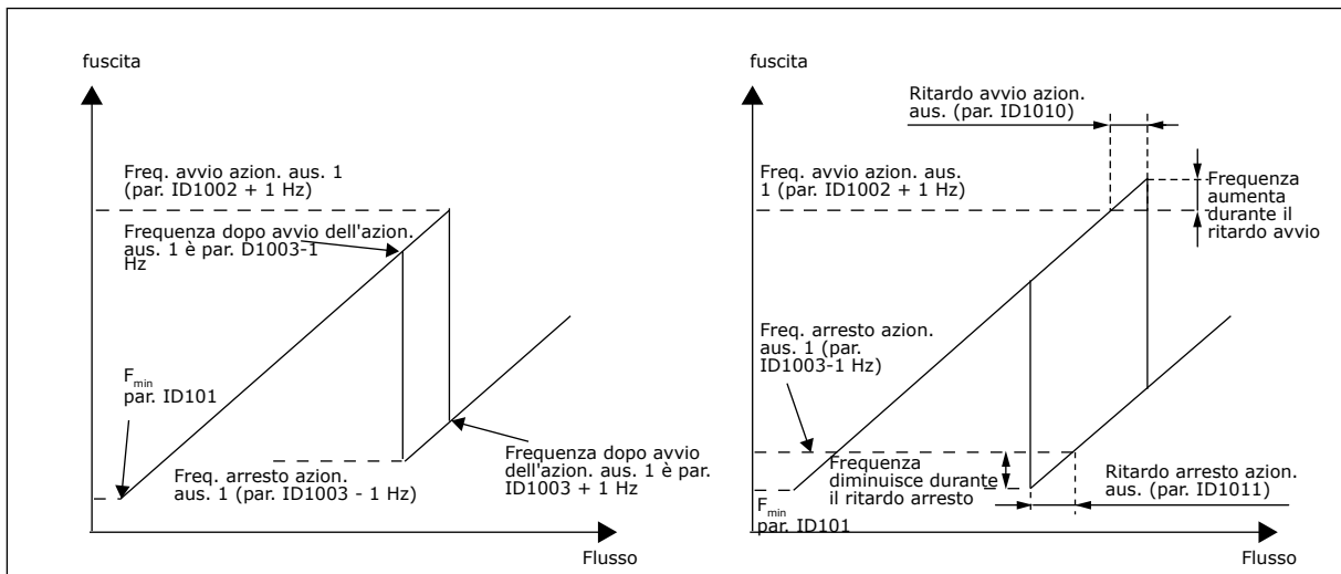
Fig. 79: Esempio di impostazione dei parametri; azionamento a velocità variabile e un azionamento ausiliario
