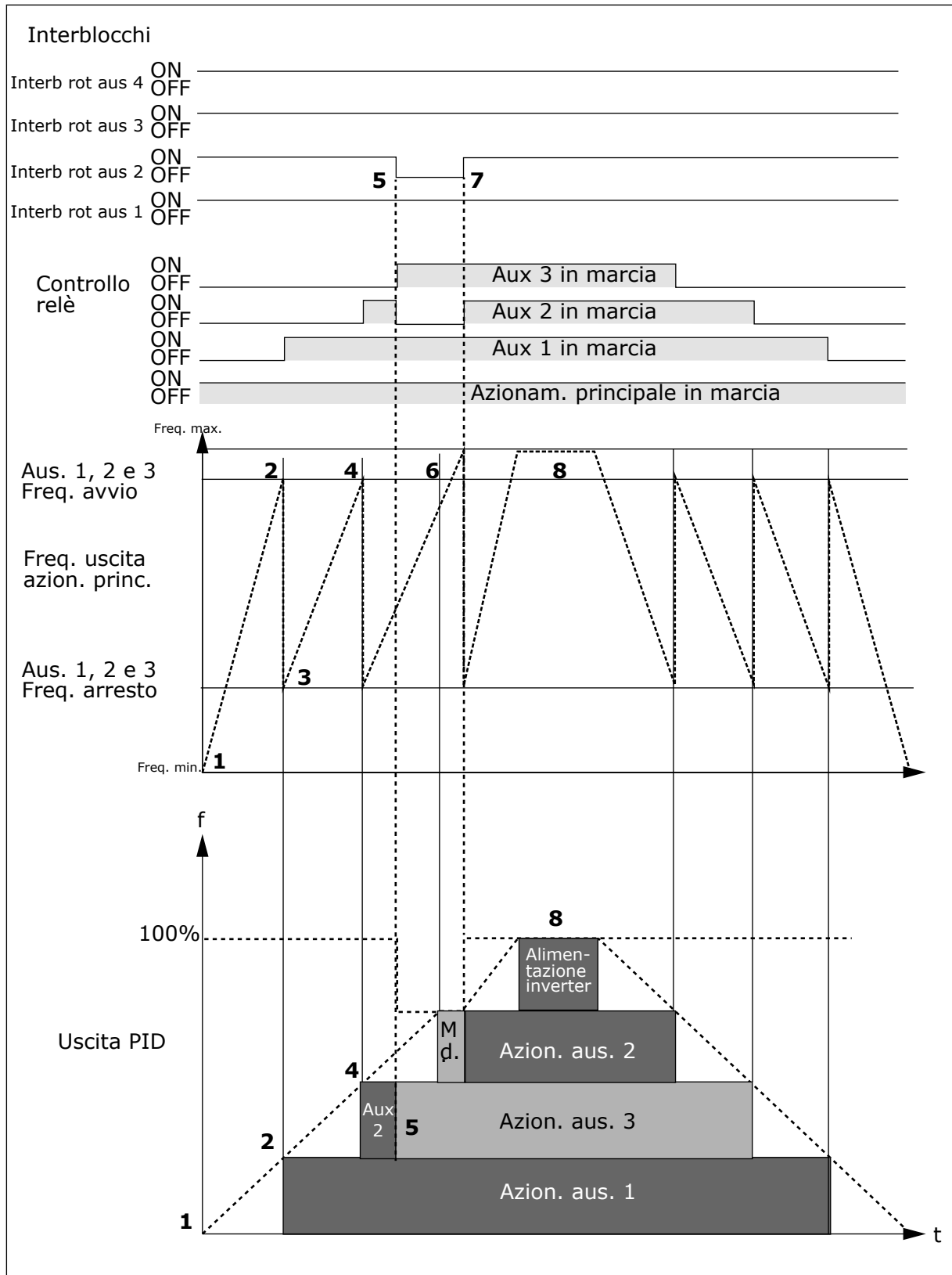
Fig. 97: Esempio della funzione dell'Applicazione per Controllo Pompe e Ventole con tre azionamenti ausiliari
