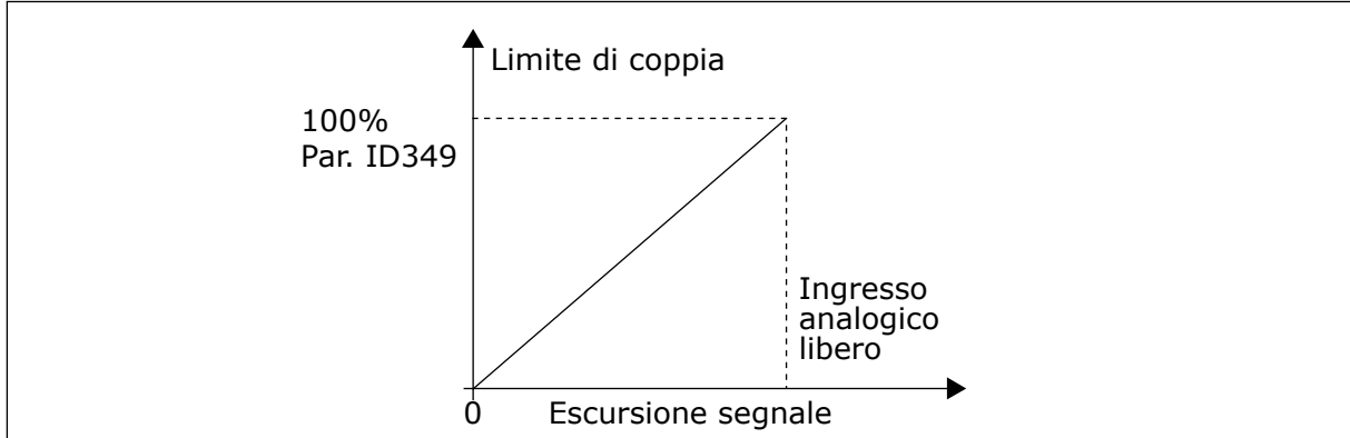
Fig. 63: Riduzione del limite di supervisione della coppia
