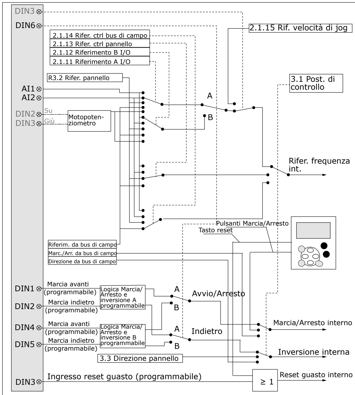
Fig. 9: Logica del segnale di controllo dell'Applicazione di Controllo Locale/Remoto
