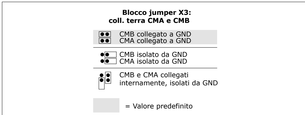
Fig. 11: Selezioni jumper
