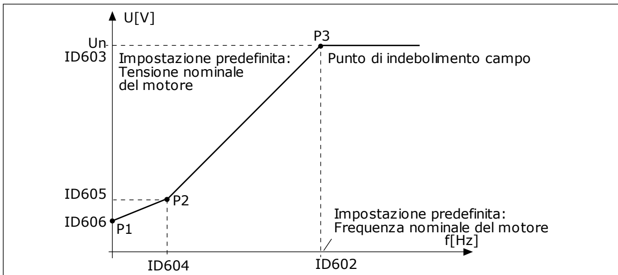
Fig. 25: la curva V/f programmabile
