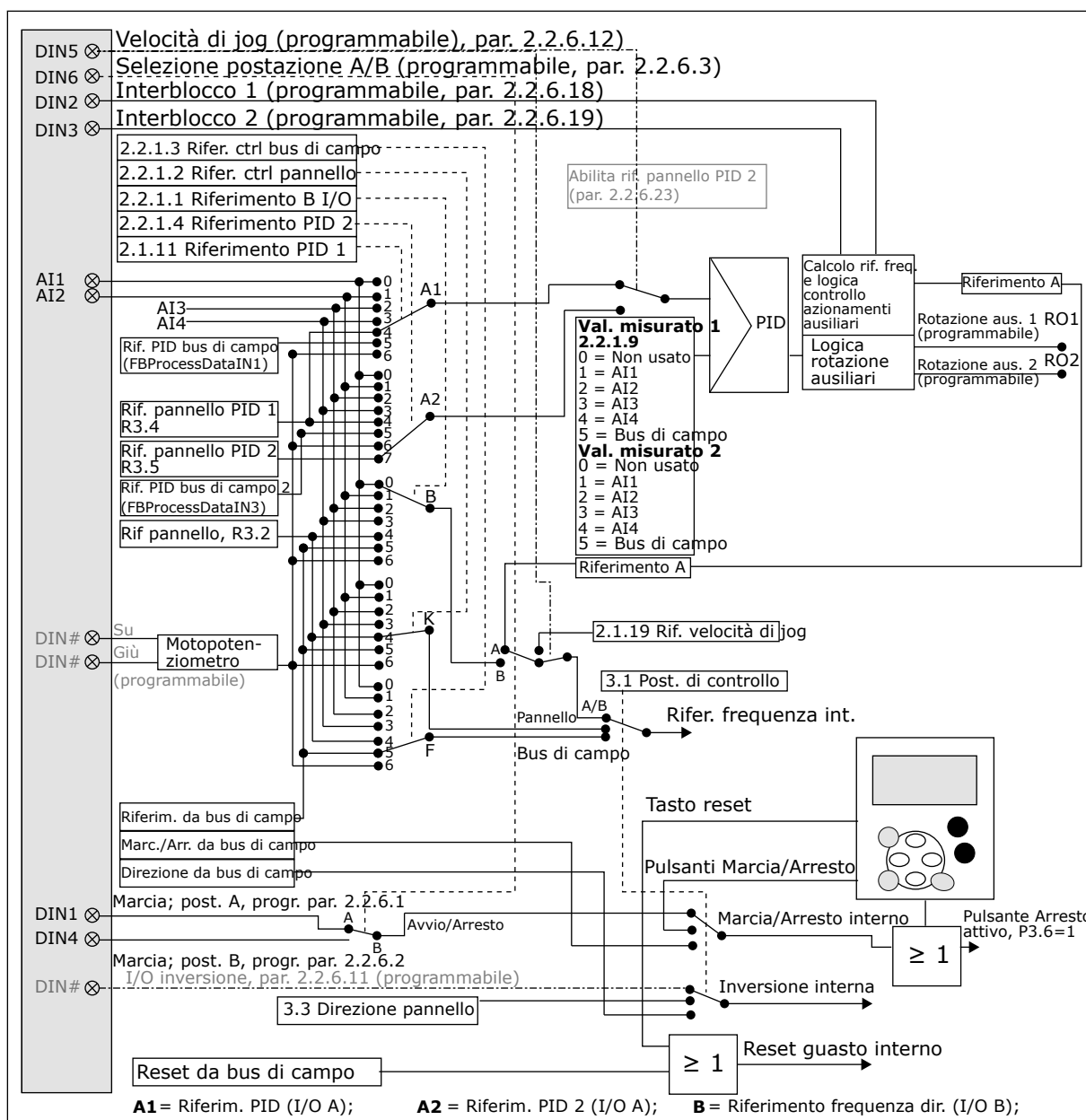
Fig. 23: Logica del segnale di controllo dell'Applicazione per Controllo Pompe e Ventole
