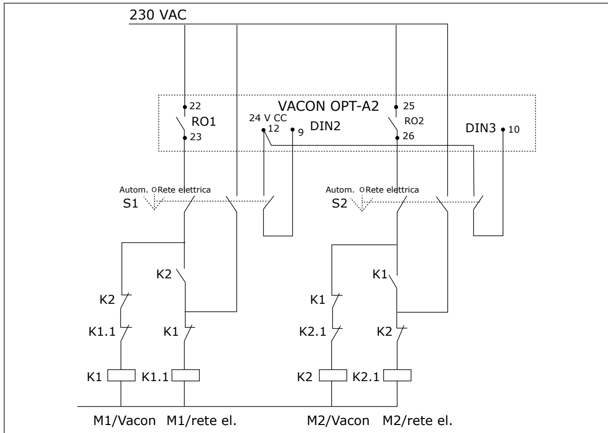
Fig. 21: Sistema di rotazione ausiliari pompa, schema dei collegamenti
