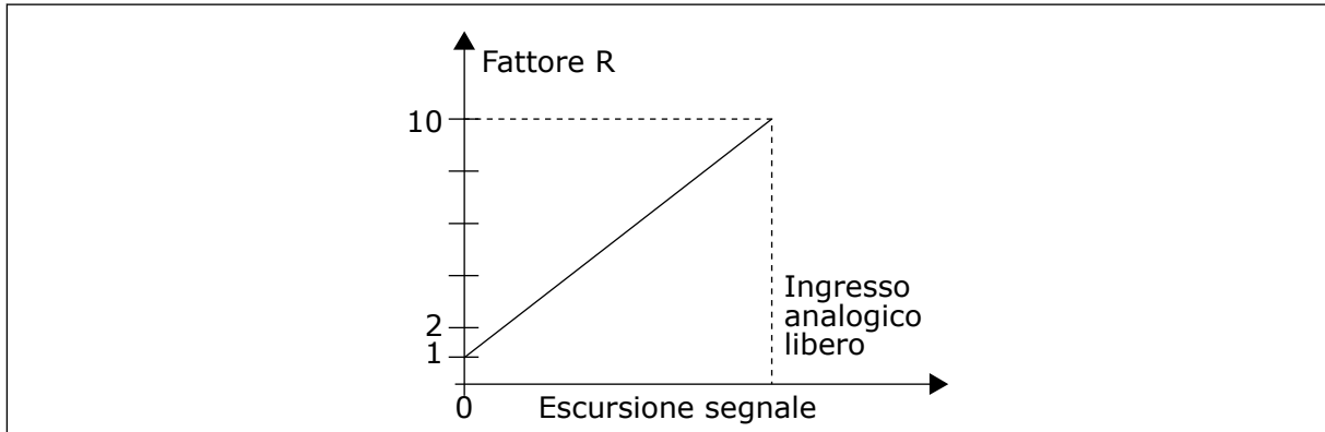
Fig. 62: Riduzione dei tempi di accelerazione e decelerazione
