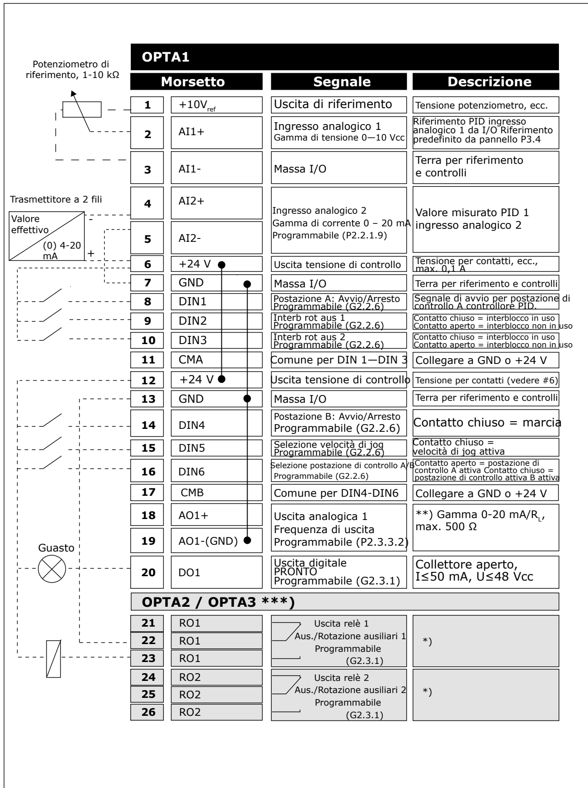
Fig. 19: Configurazione I/O predefinita Applicazione per Controllo Pompe e Ventole ed esempio di connessione (con trasmettitore a 2 fili)
