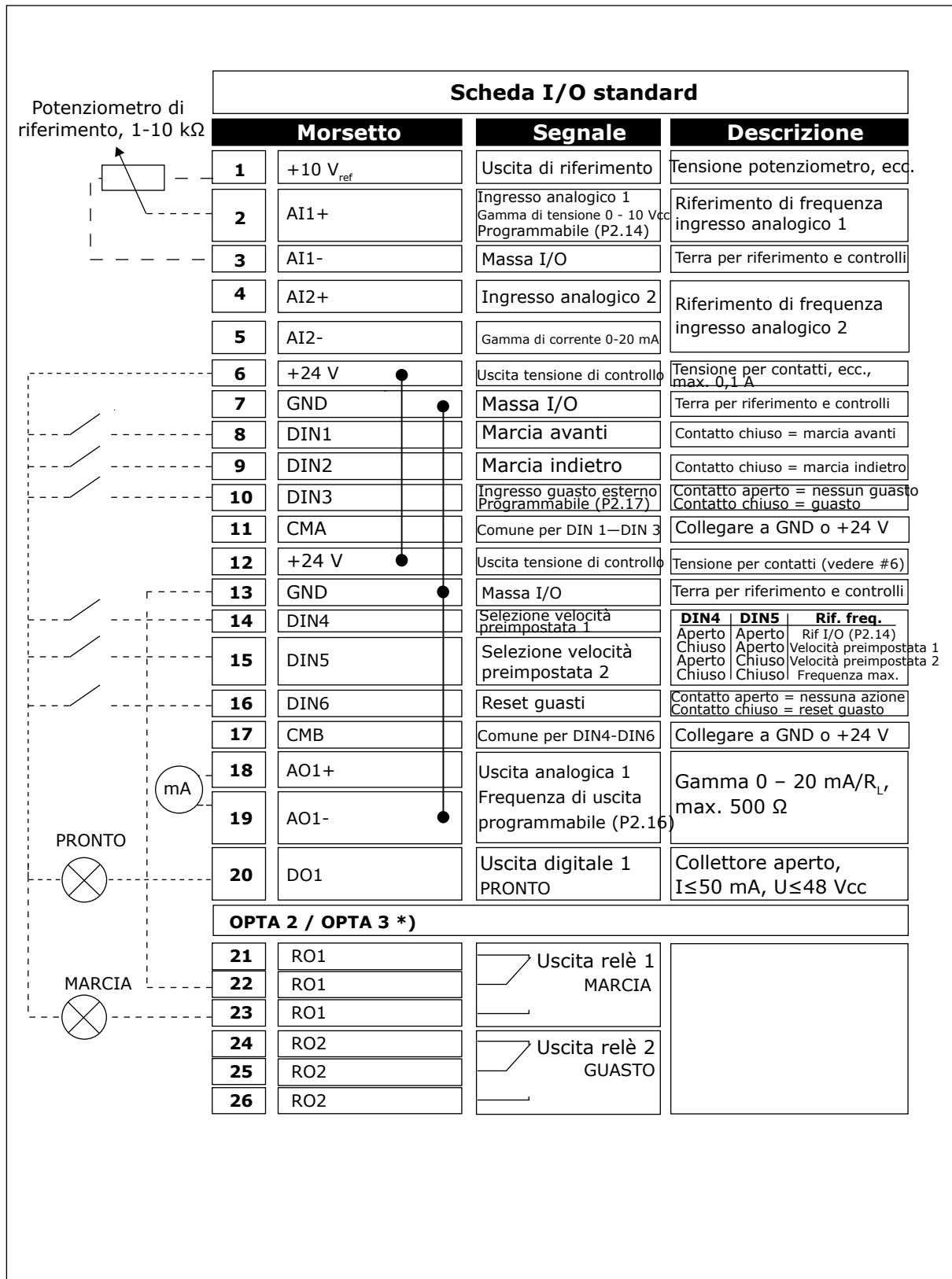
Fig. 1: Configurazione I/O predefinita dell'Applicazione Base
