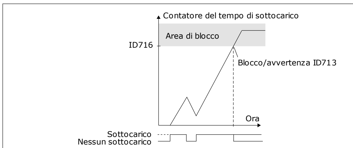
Fig. 77: la funzione contatore tempo di sottocarico
