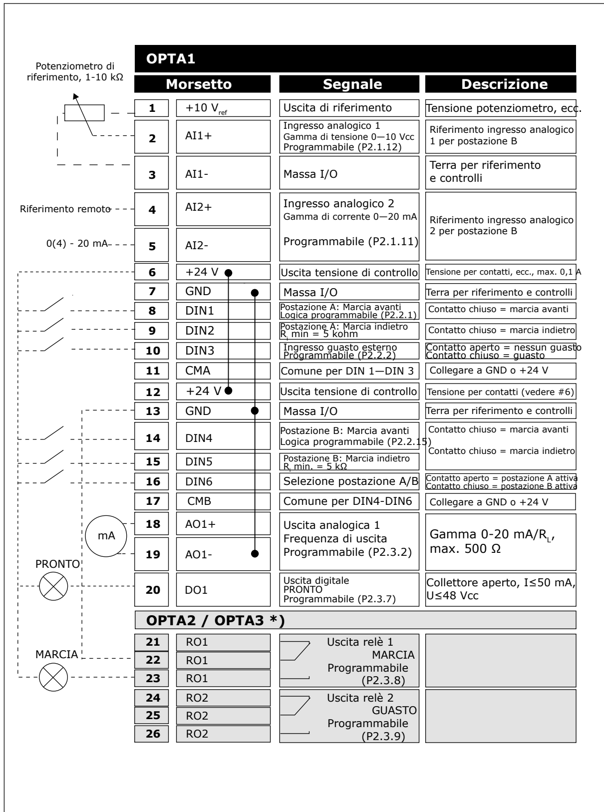
Fig. 7: Configurazione I/O predefinita per l'Applicazione di Controllo Locale/Remoto
