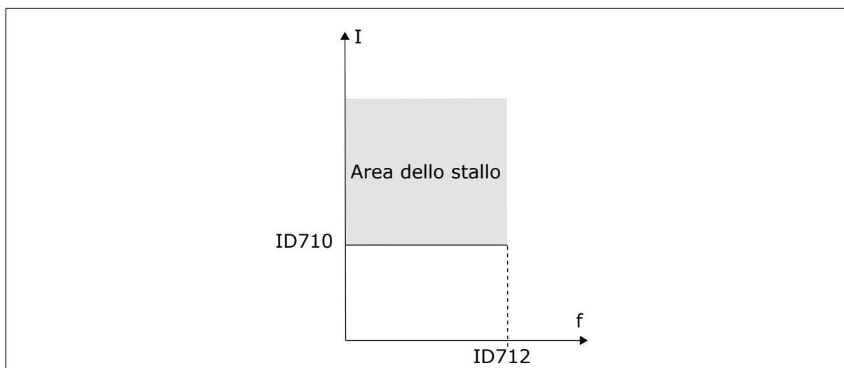
Fig. 74: le impostazioni relative alle caratteristiche dello stallo
