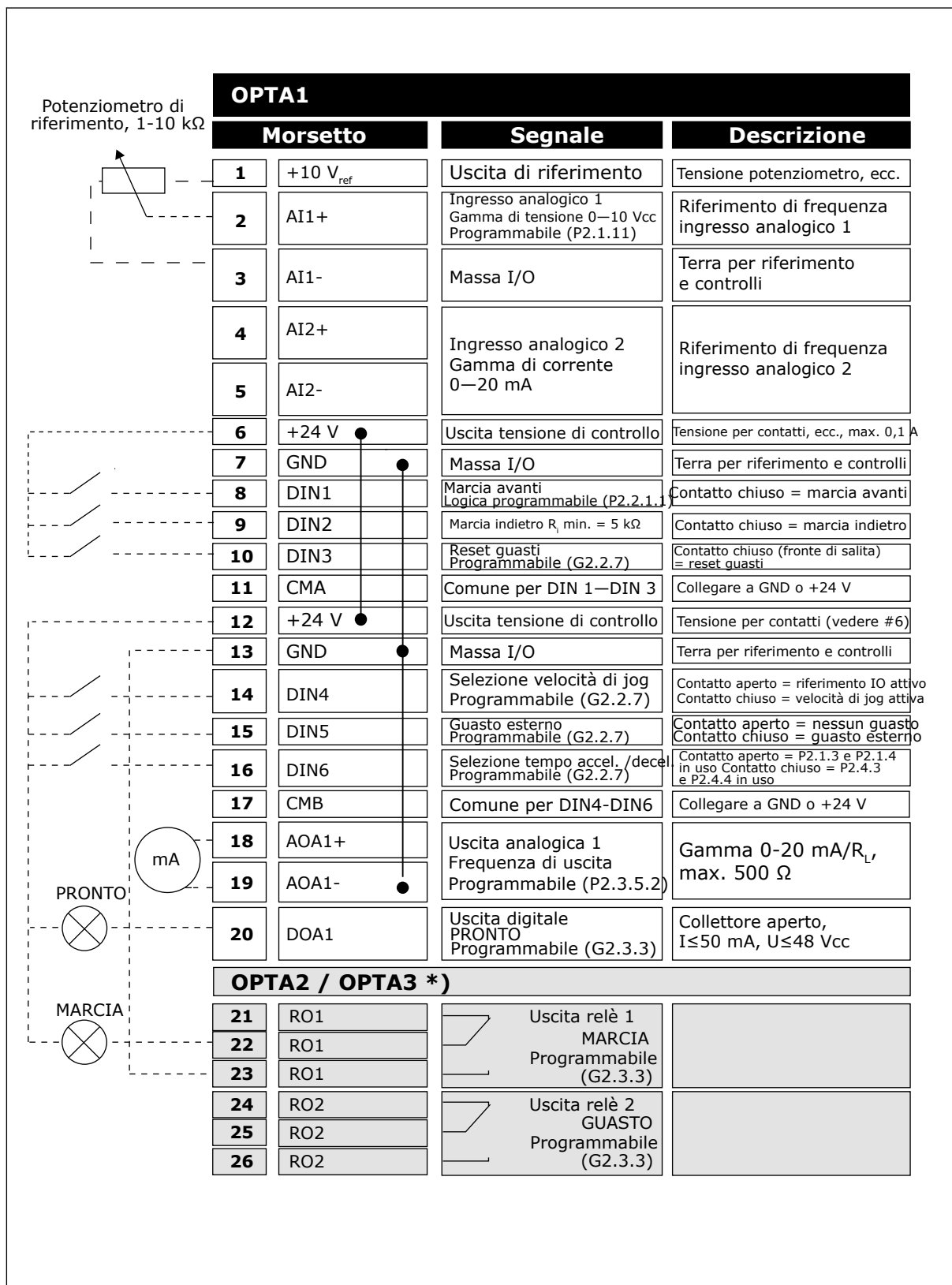
Fig. 16: Configurazione I/O predefinita Applicazione di Controllo Multifunzione ed esempio di connessione
