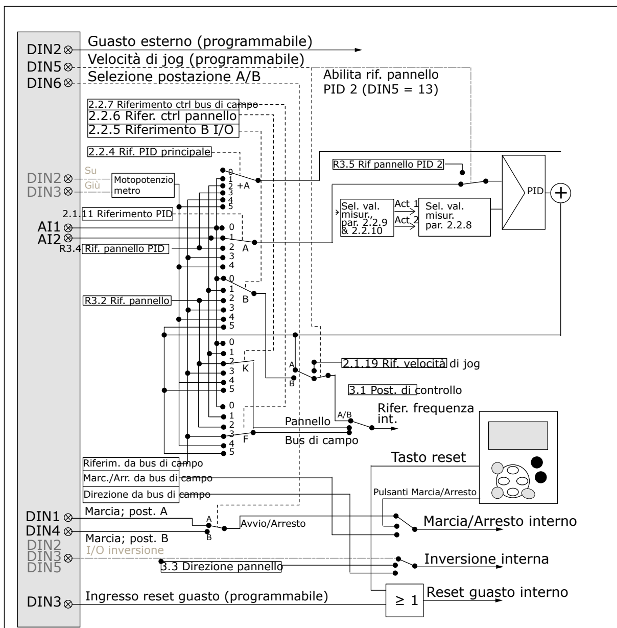
Fig. 15: Logica del segnale di controllo dell'Applicazione di Controllo PID
