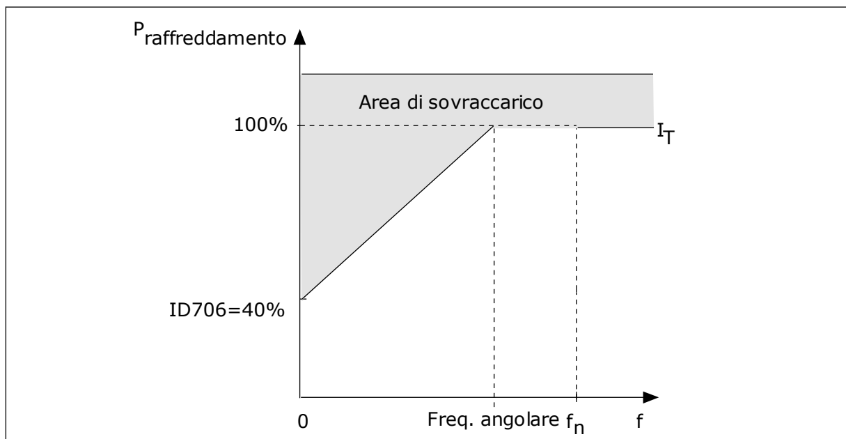
Fig. 72: Curva I_T della corrente di protezione termica del motore
