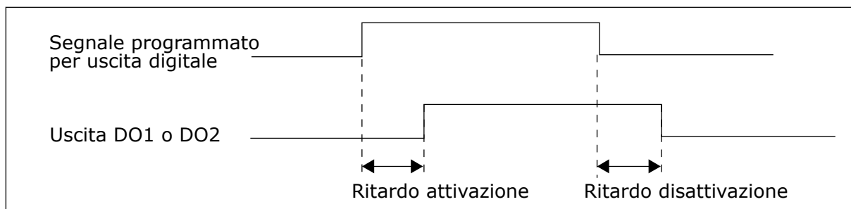
Fig. 65: Uscite digitali 1 e 2, ritardi di attivazione e disattivazione
