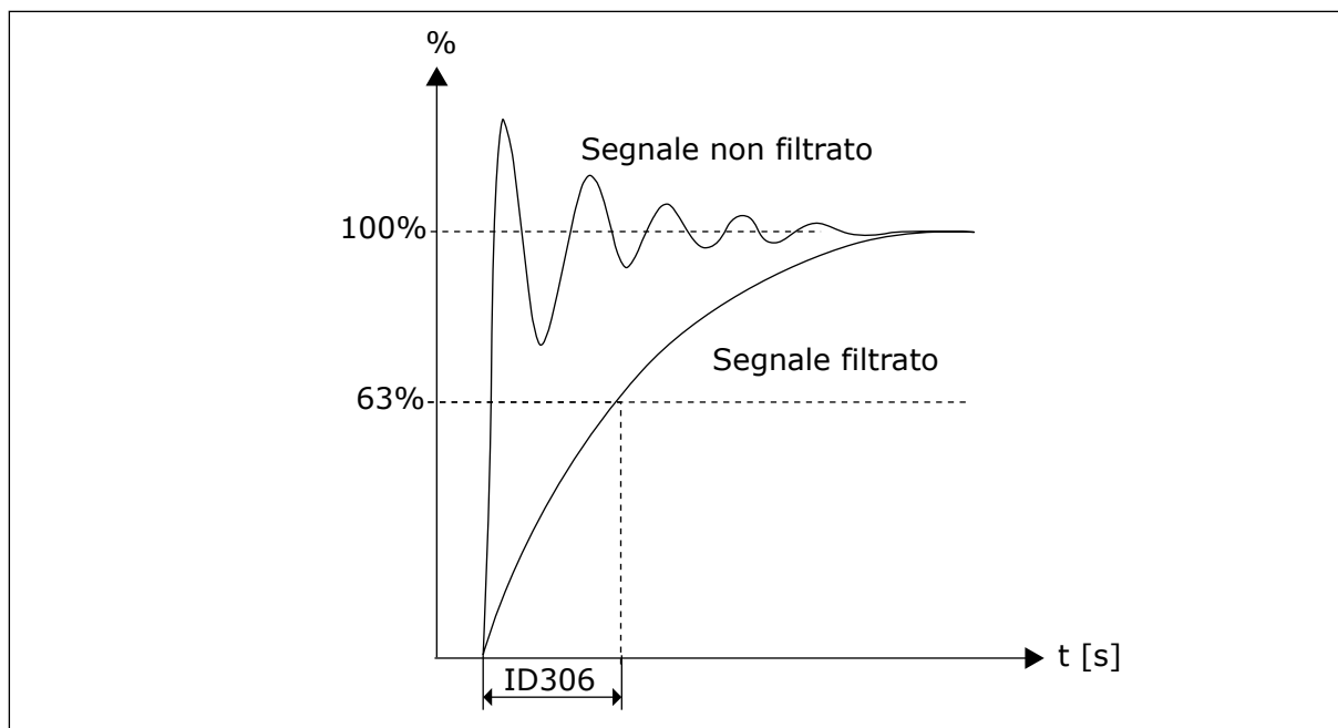
Fig. 36: Filtraggio di riferimento
