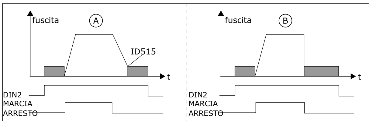
Fig. 41: Comando frenatura in CC (selezione 12) selezionato per DIN2
