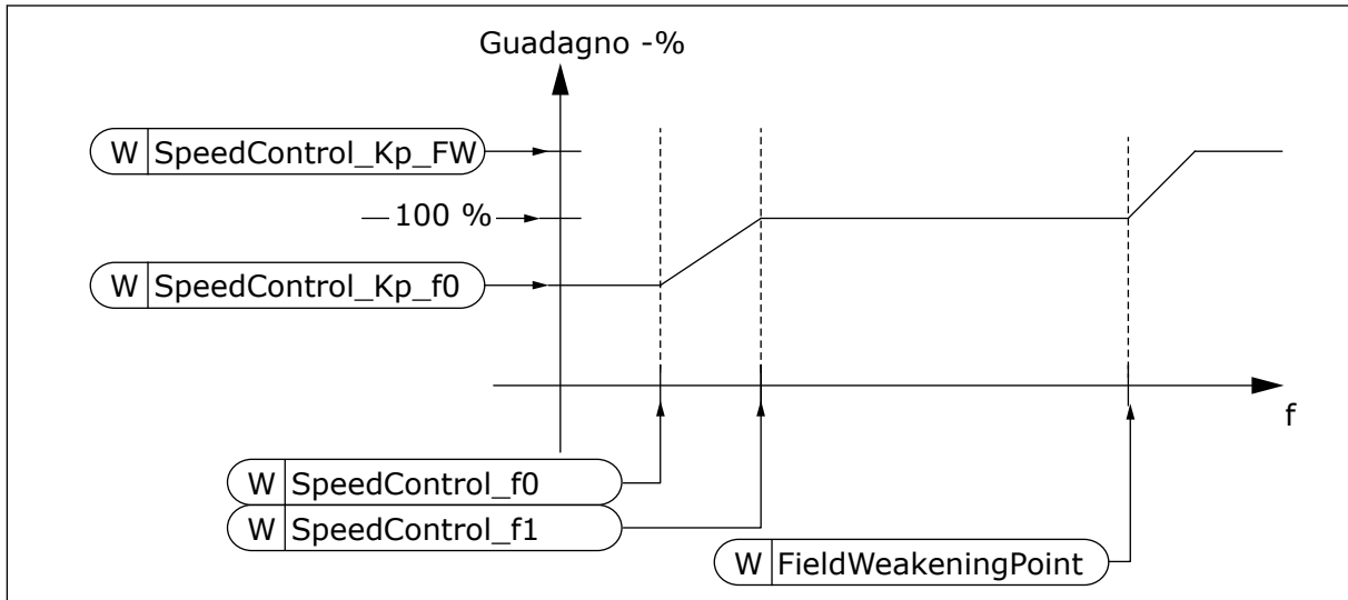
Fig. 96: Guadagno del regolatore di velocità adattativo
