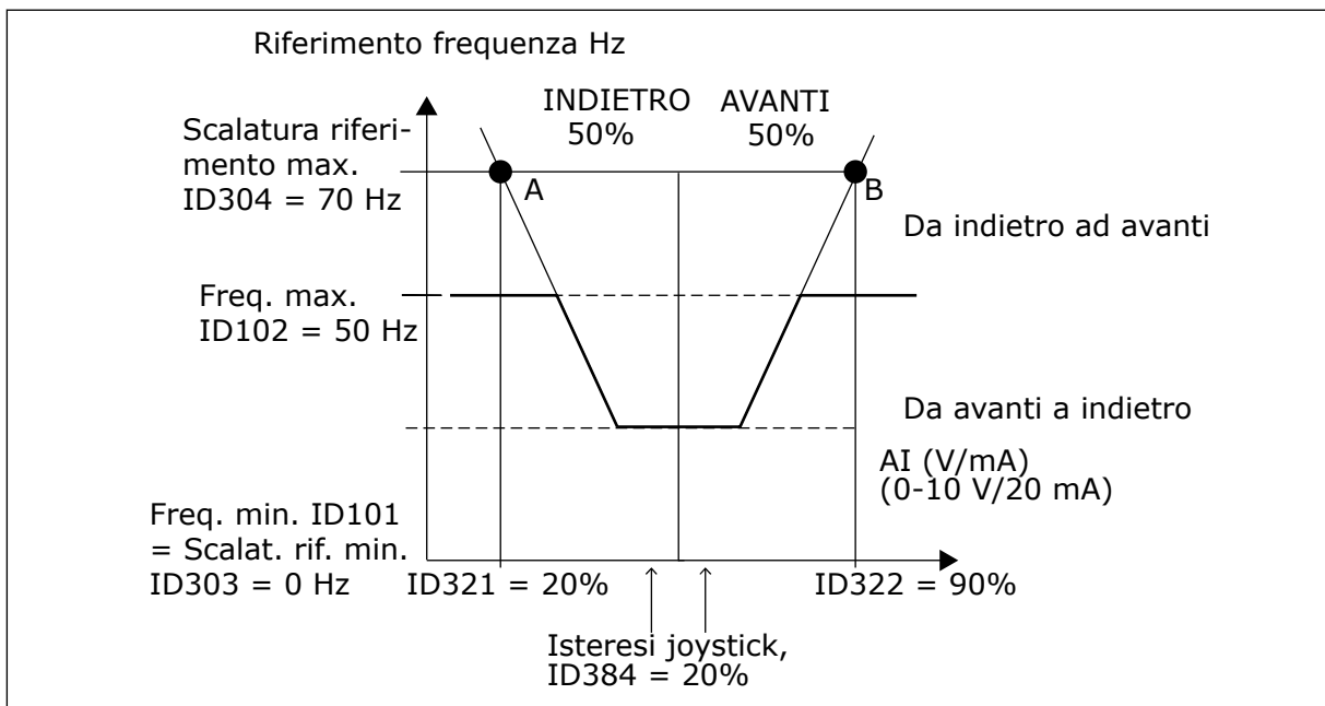
Fig. 60: Isteresi del joystick con frequenza minima a 35 Hz
