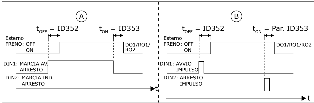
Fig. 48: Controllo freno esterno
