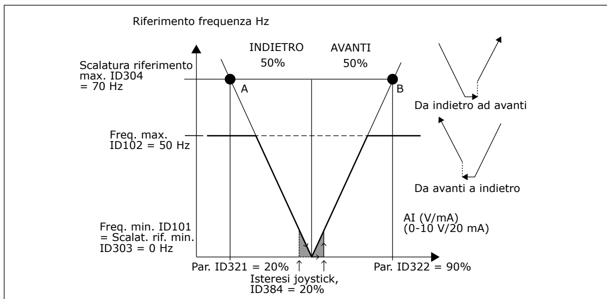
Fig. 58: Esempio di isteresi del joystick. In questo esempio il valore del parametro ID385 (limite standby) = 0
