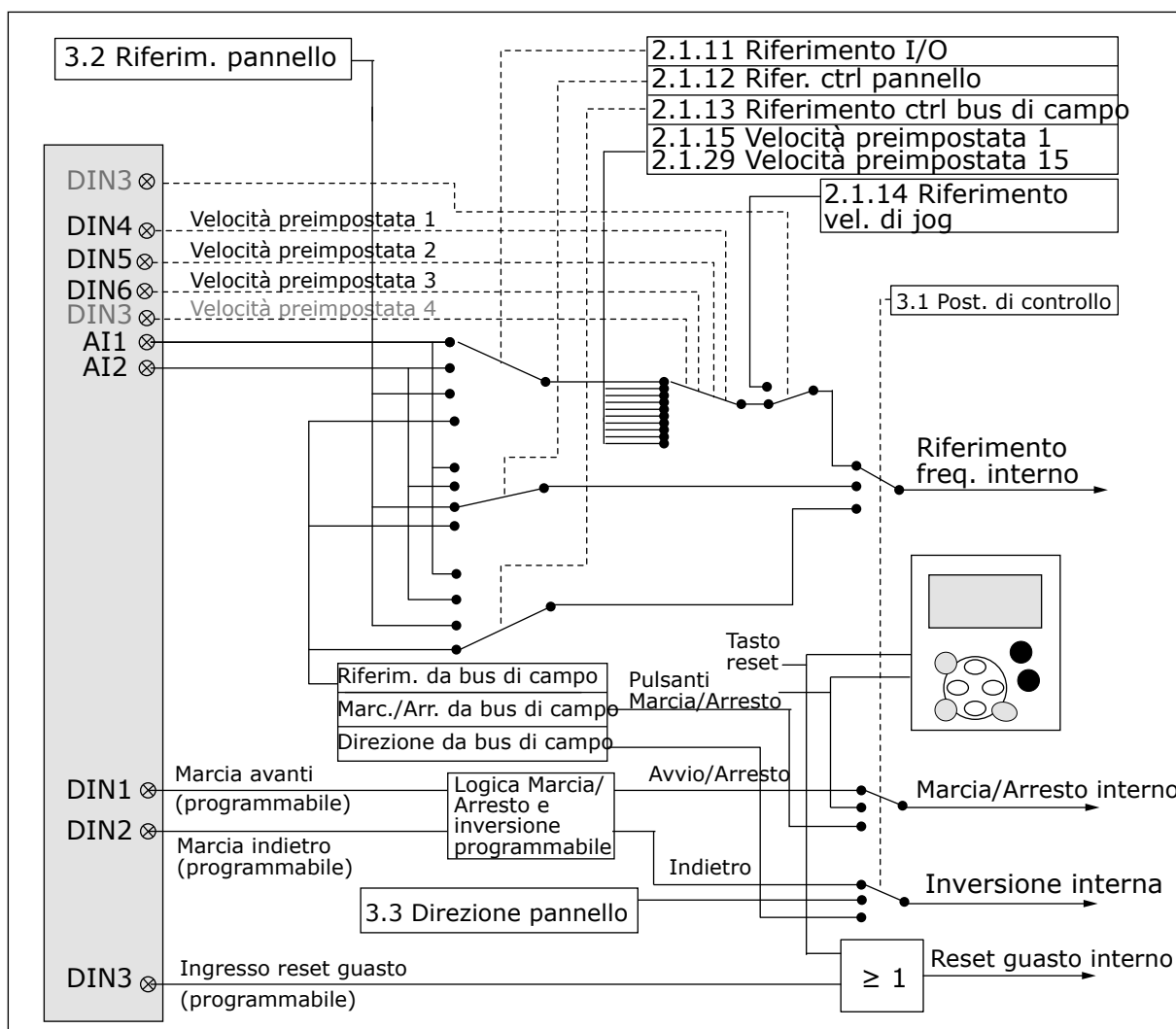
Fig. 12: Logica del segnale di controllo dell'Applicazione di Controllo della Velocità Multistep
