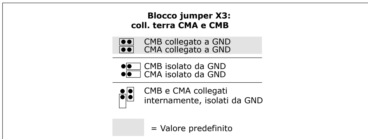
Fig. 5: Selezioni jumper
