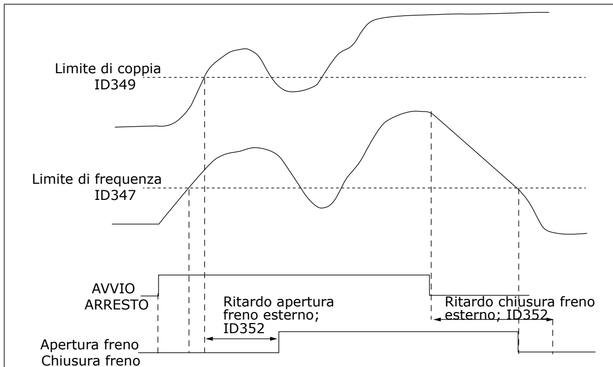
Fig. 92: Controllo freno con limiti aggiuntivi
