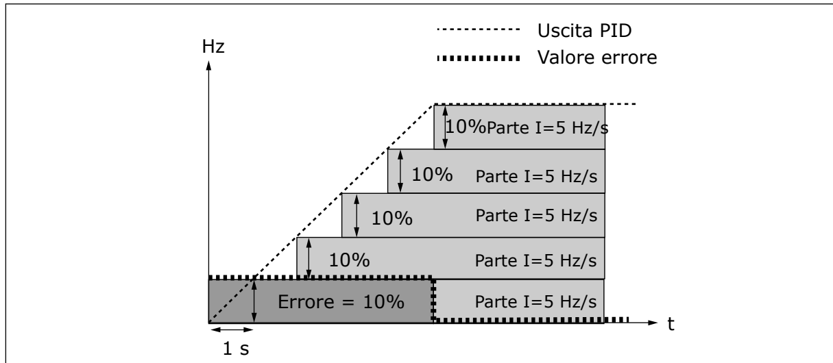
Fig. 27: Funzione del controllore PID come regolatore I
