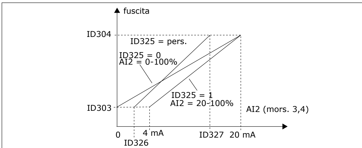
Fig. 45: Scalatura ingresso analogico AI2
