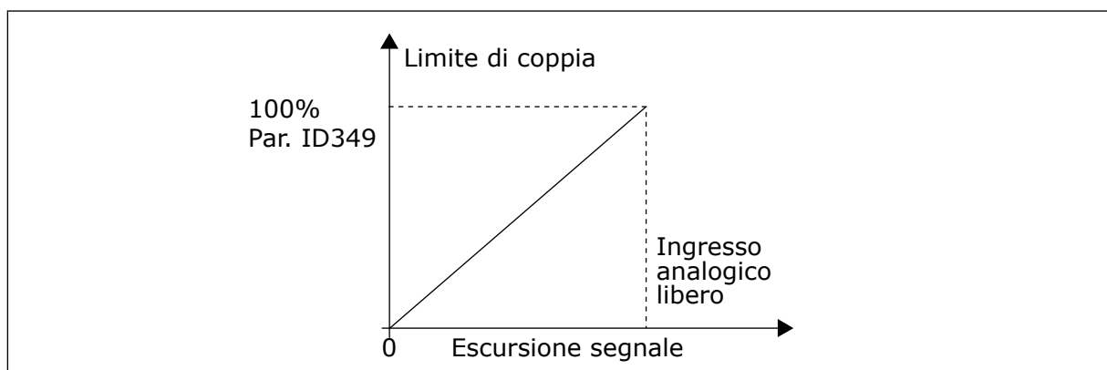
Fig. 64: Scalatura del limite di coppia del motore
