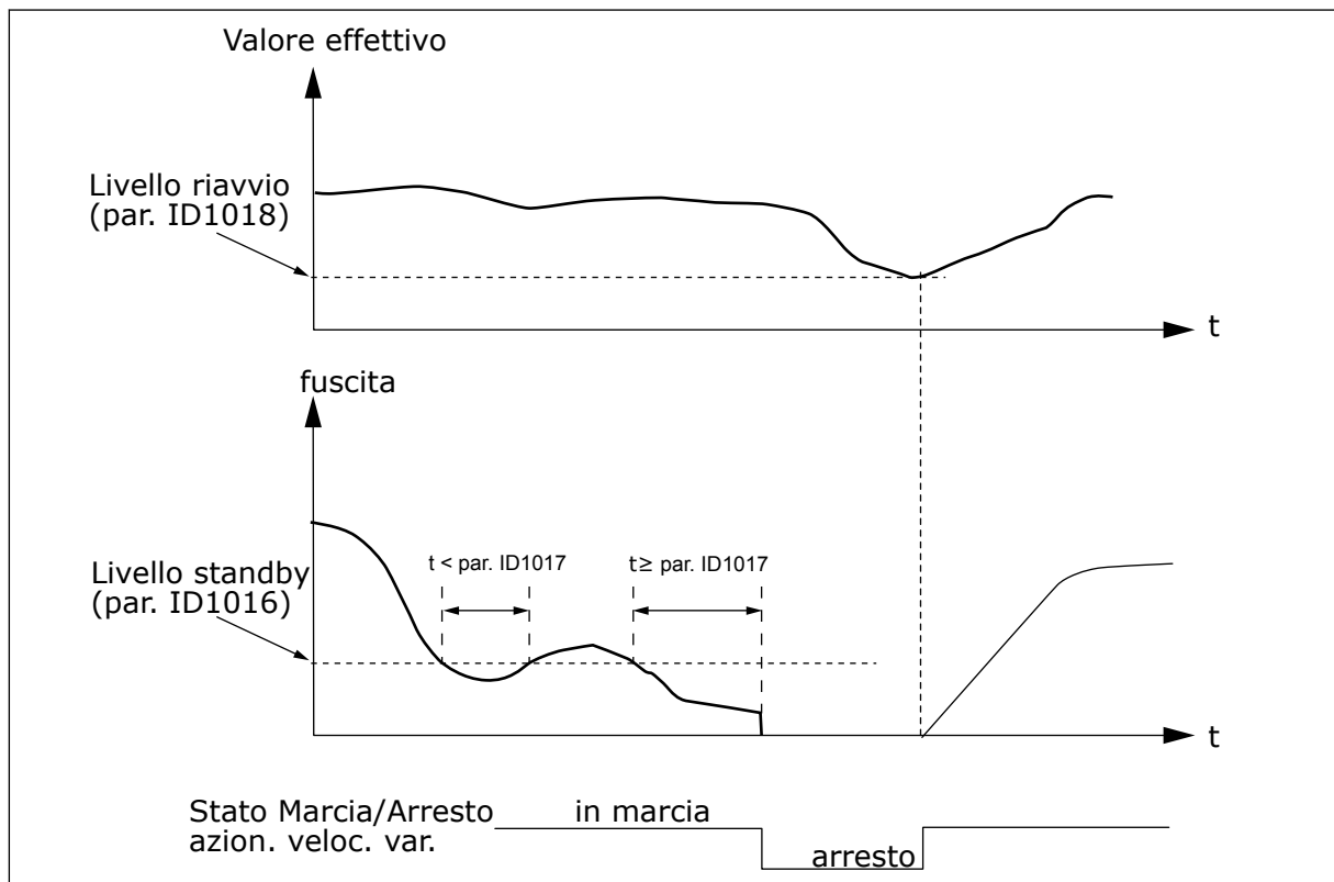
Fig. 81: Funzione standby dell'inverter
