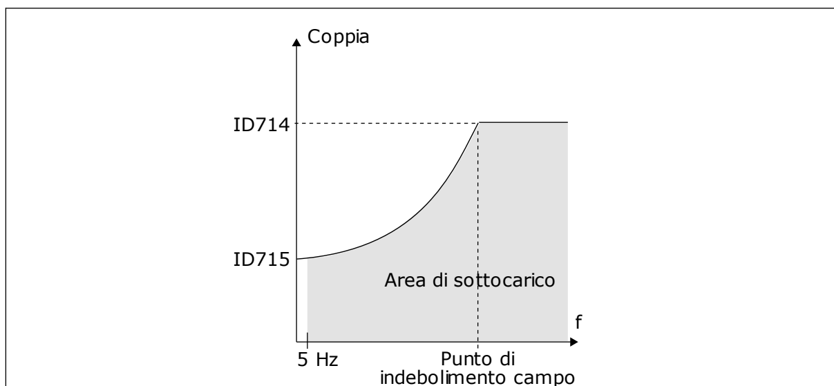
Fig. 76: impostazione del carico minimo
