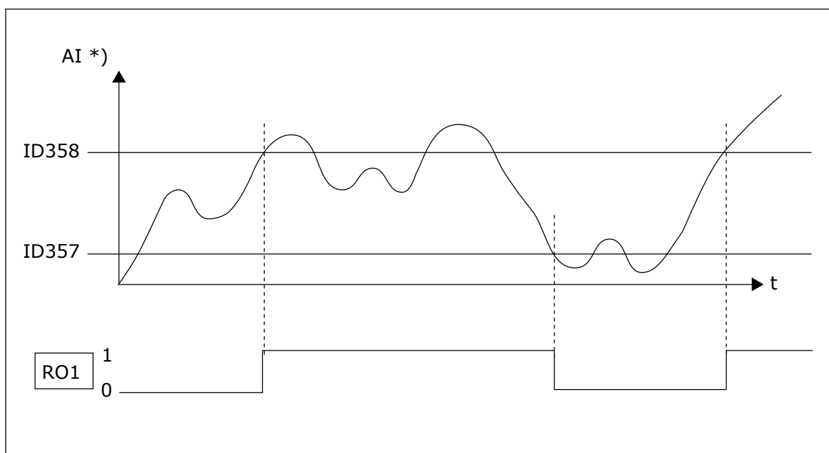
Fig. 49: Esempio del controllo On/Off
