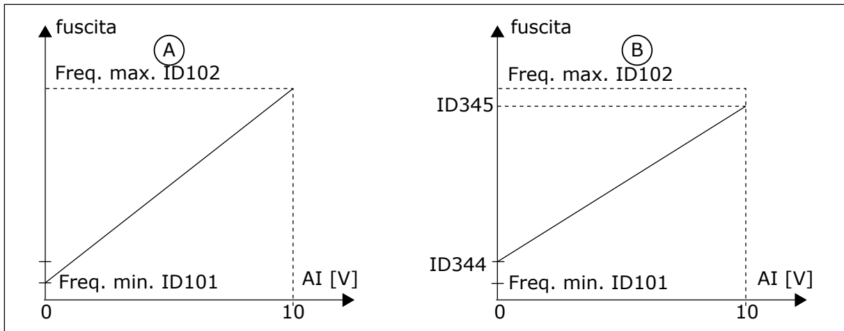
Fig. 47: Scalatura di riferimento, valore massimo
