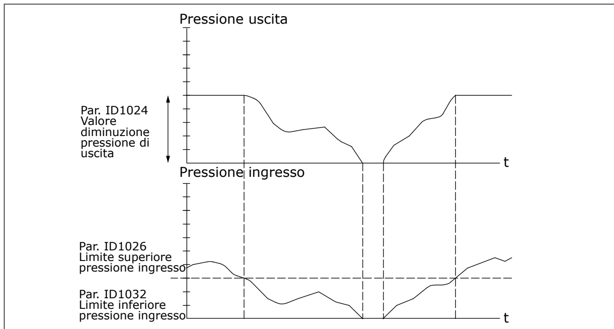
Fig. 84: Comportamento della pressione d'uscita in base alla pressione d'ingresso e alle impostazioni dei parametri
