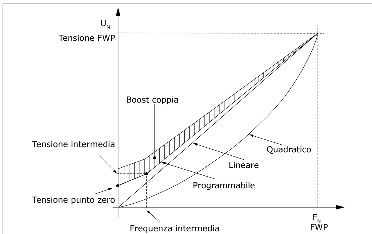
Fig. 26: Ottimizzazione V/f
