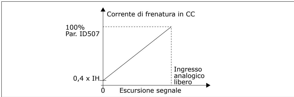
Fig. 51: Riduzione della corrente di frenatura in CC
