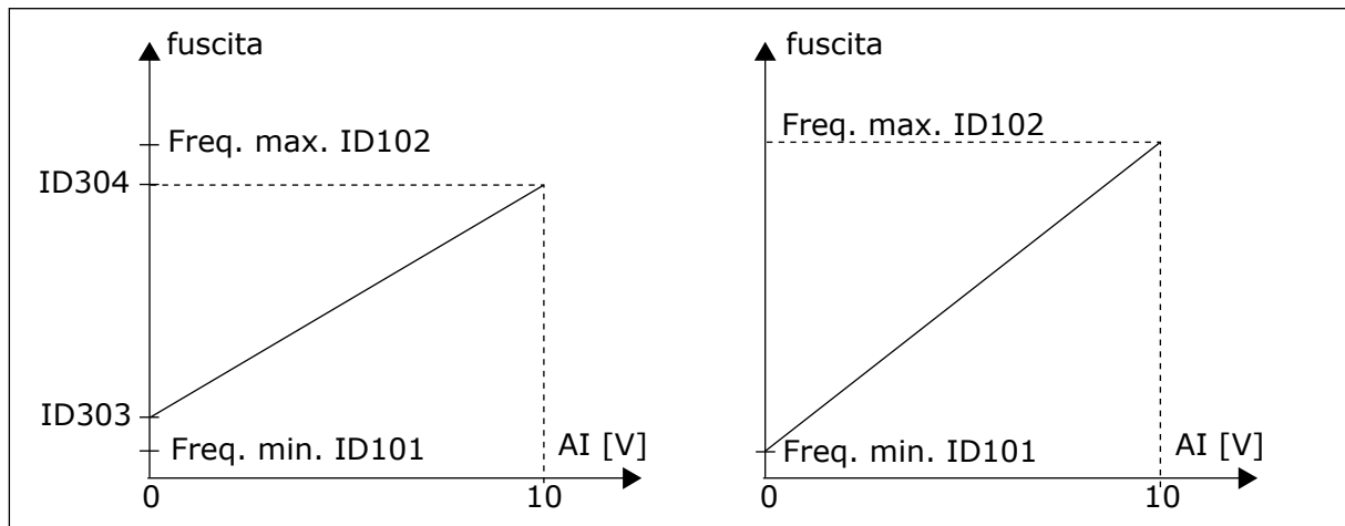
Fig. 34: A sinistra: scalatura di riferimento. A destra: nessuna scalatura in uso (parametro ID303 = 0)
