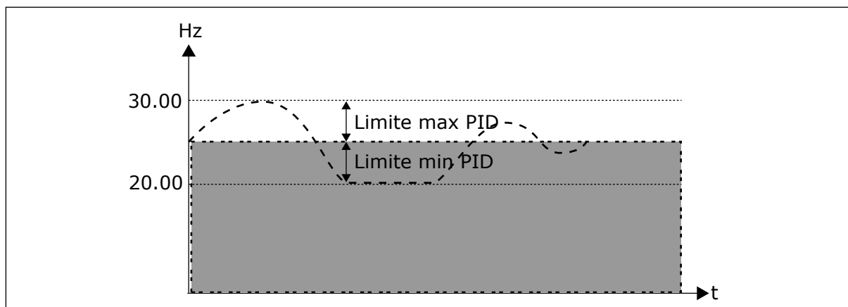
Fig. 57: Riferimento somma PID
