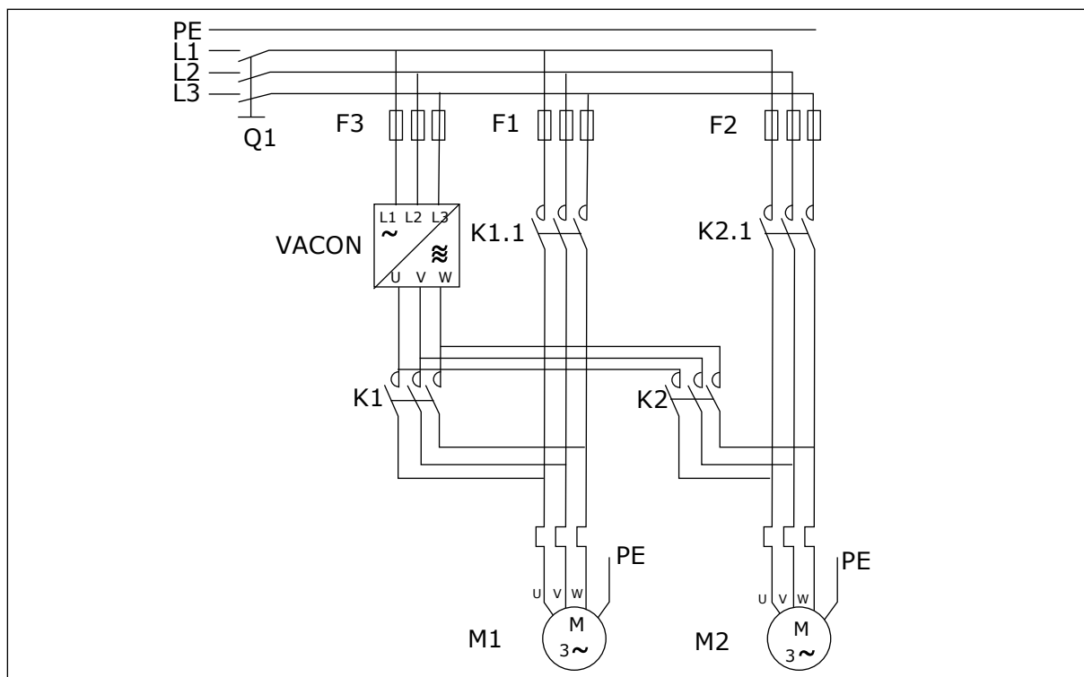
Fig. 98: Esempio di rotazione ausiliari con 2 pompe, schema principale
