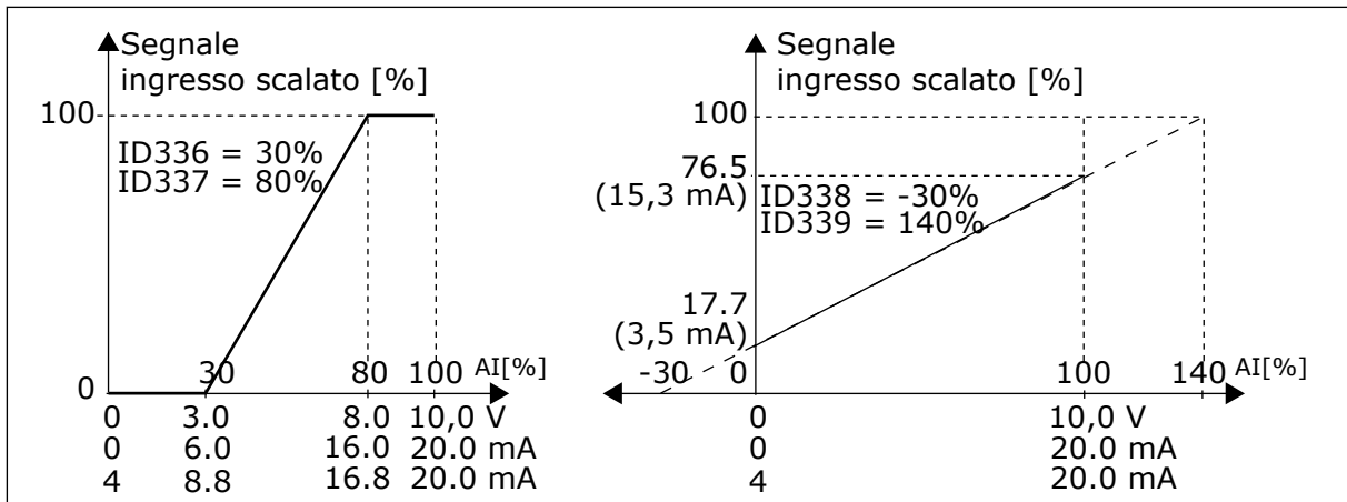
Fig. 46: Esempi di scalatura del segnale del valore misurato
