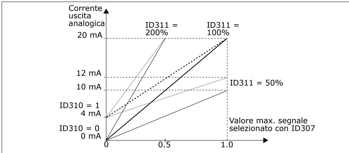
Fig. 39: Scalatura uscita analogica
