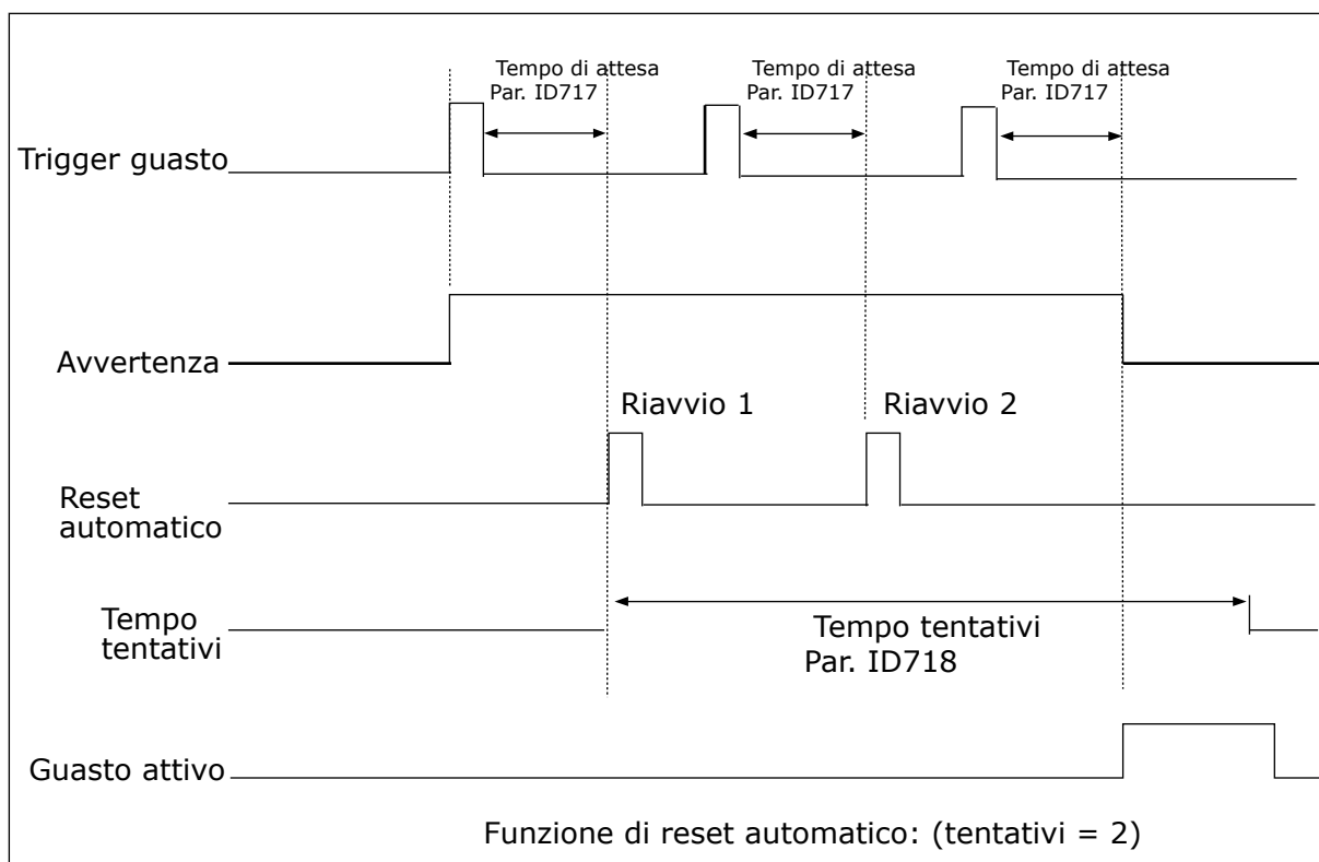
Fig. 78: Esempio di riavviamento automatico con due riavviamenti
