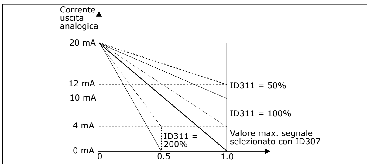
Fig. 38: Inversione uscita analogica
