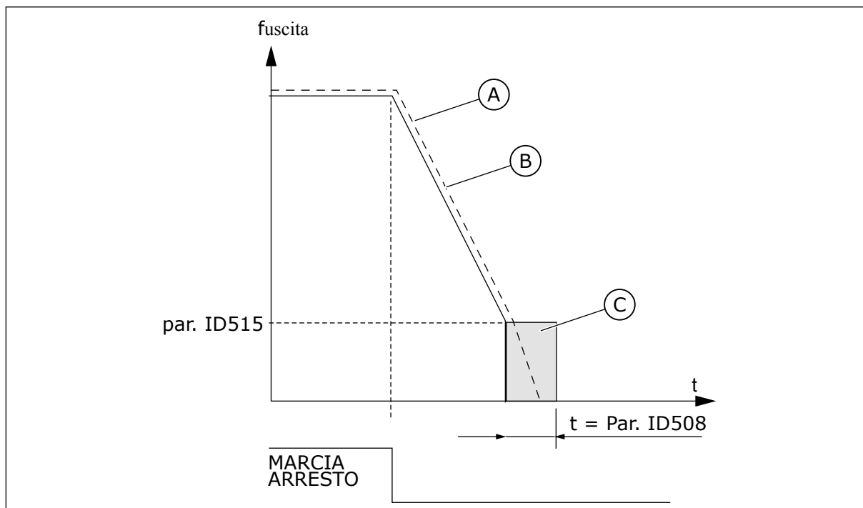
Fig. 69: Tempo di frenatura in CC nella Funzione Arresto = Rampa
