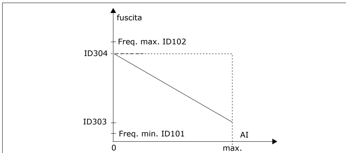
Fig. 35: Inversione riferimento
