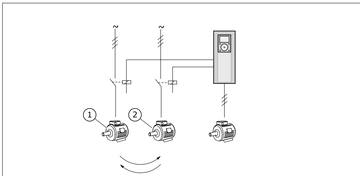
Fig. 86: Rotazione ausiliari applicata solo agli azionamenti ausiliari
