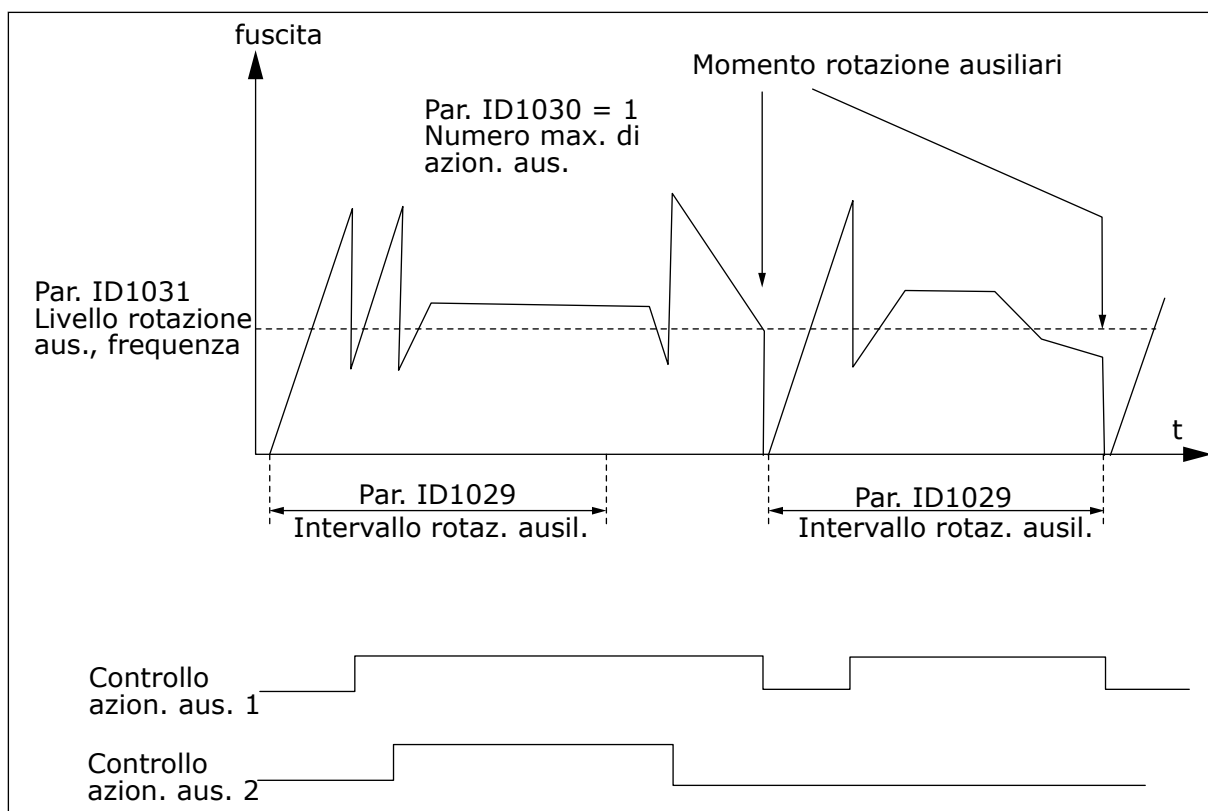
Fig. 88: Intervallo e limiti della rotazione ausiliari
