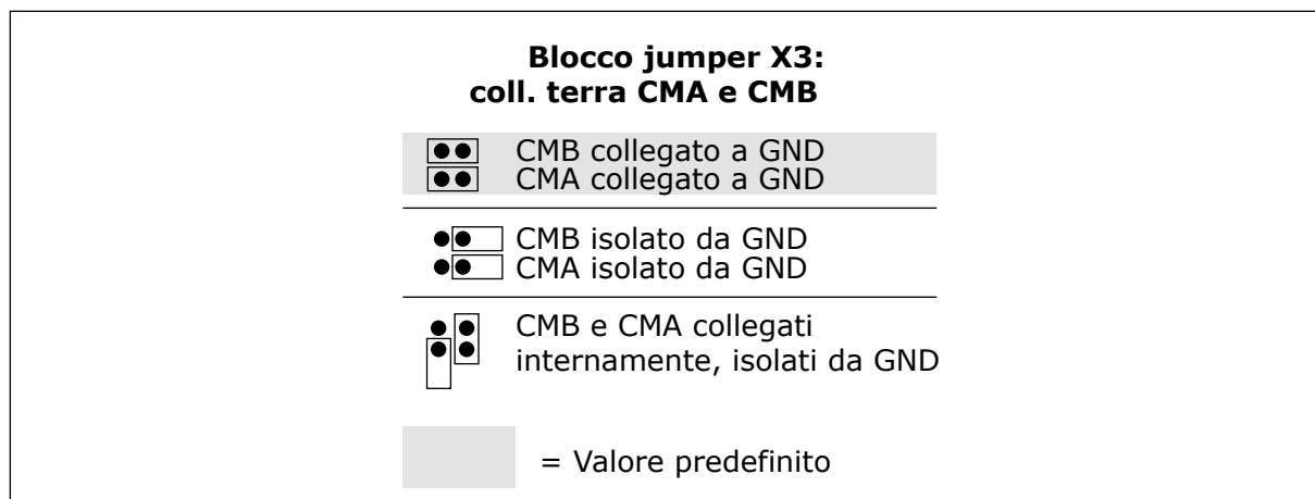
Fig. 20: Selezioni jumper
