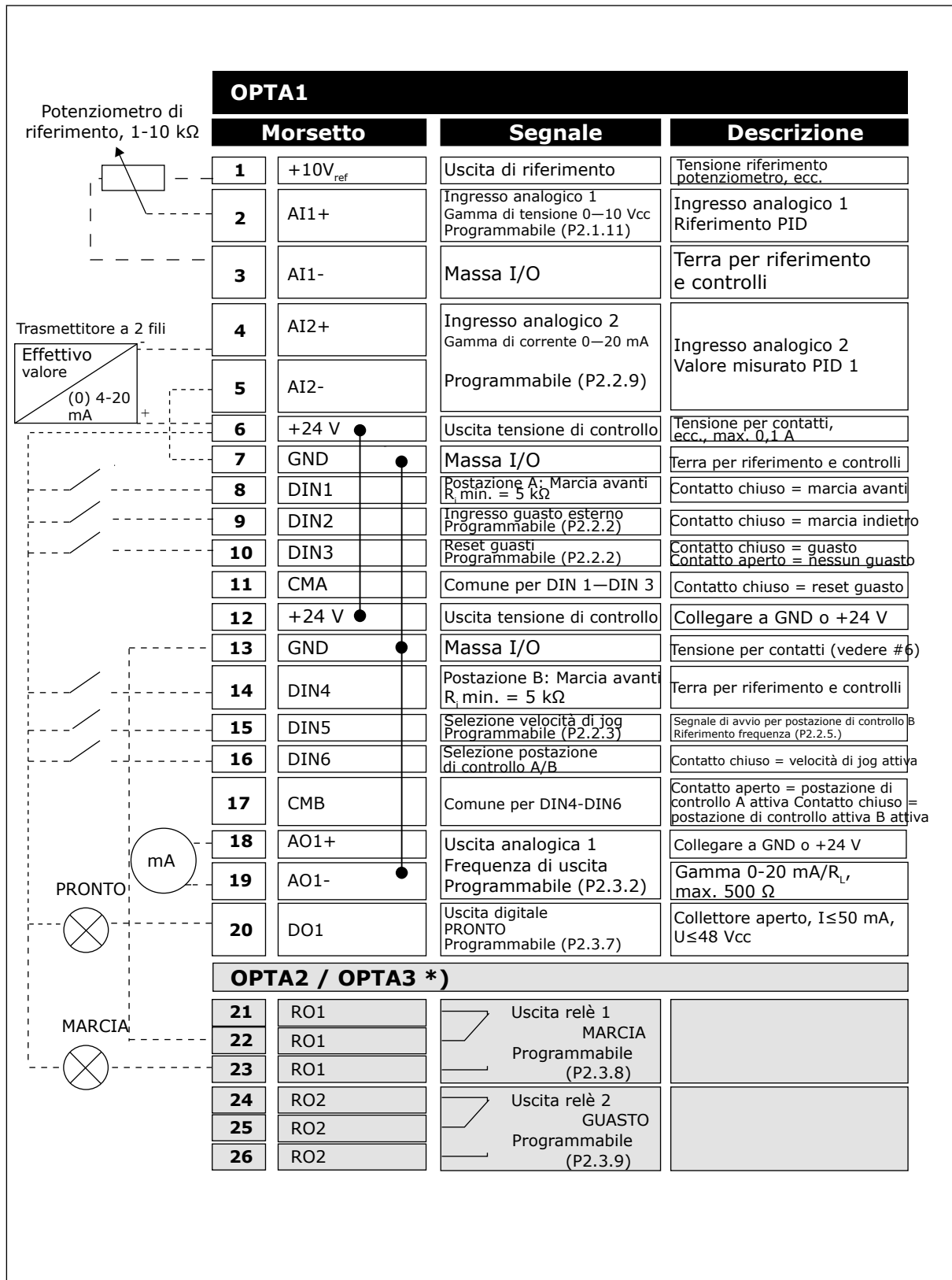
Fig. 13: Configurazione I/O predefinita per l'Applicazione PID (con trasmettitore a 2 fili)
