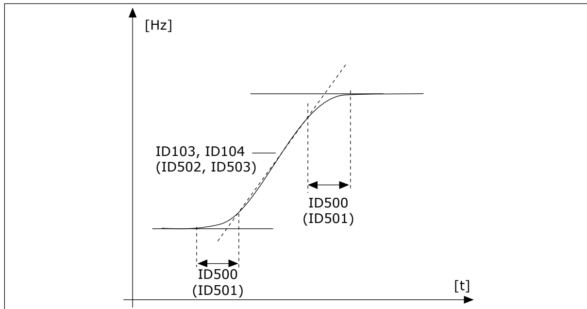
Fig. 67: Accelerazione/decelerazione (sinusoidale)
