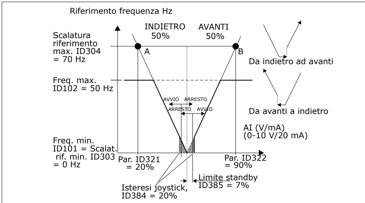
Fig. 59: Esempio della funzione del limite di standby
