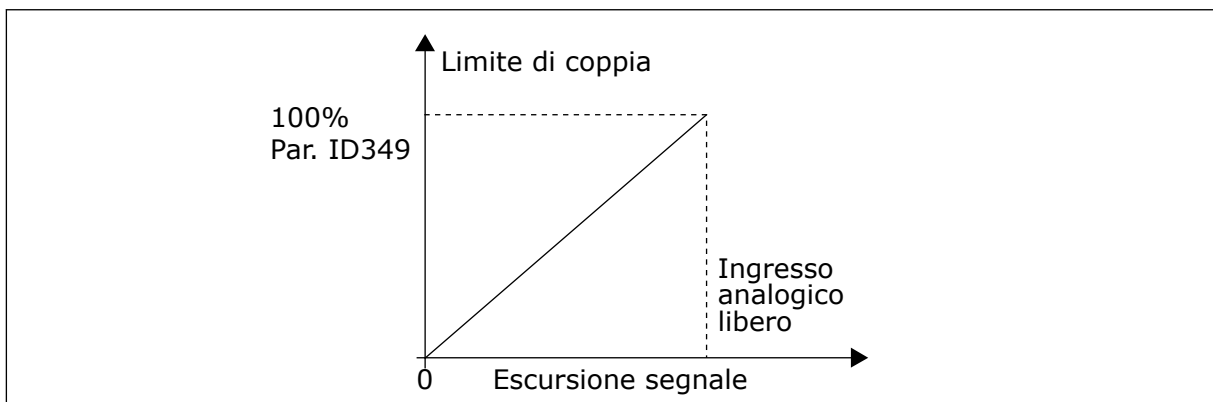
Fig. 53: Riduzione del limite di supervisione della coppia
