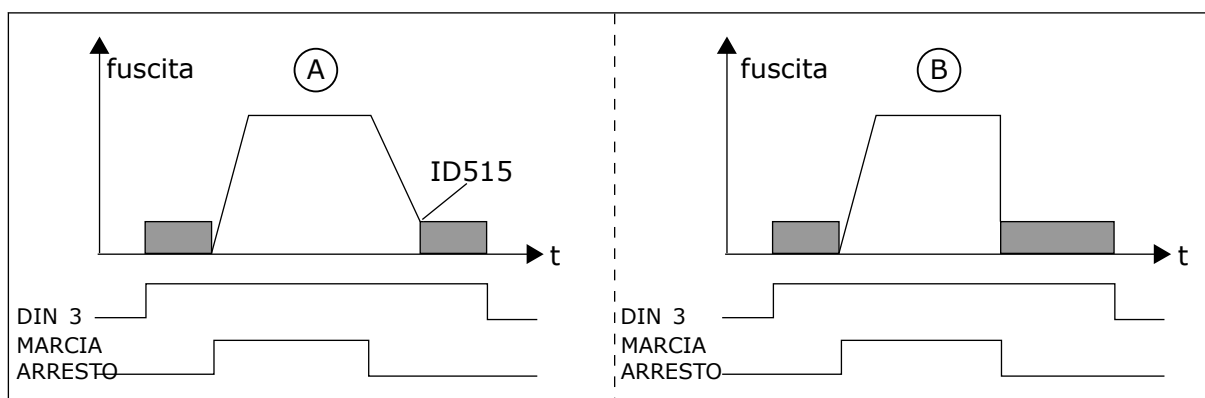
Fig. 33: DIN3 come ingresso comando freno CC
