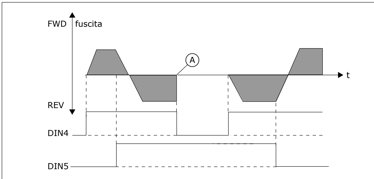
Fig. 55: Marcia, Arresto, Indietro
