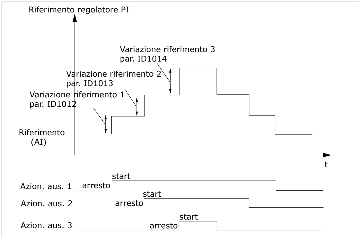
Fig. 80: Variazioni riferimento dopo l'avviamento degli azionamenti ausiliari
