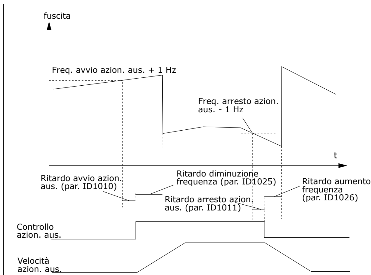
Fig. 85: Ritardi di diminuzione e aumento della frequenza
