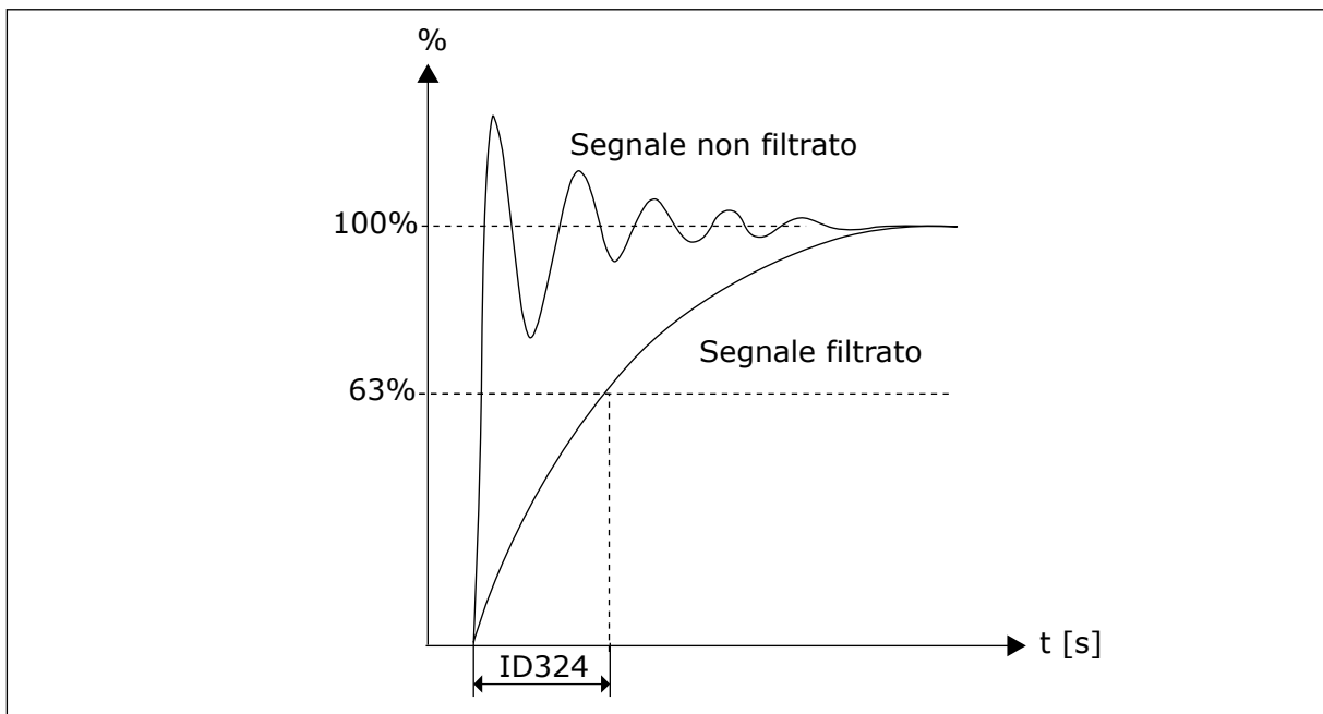
Fig. 44: Filtro segnale AI1
