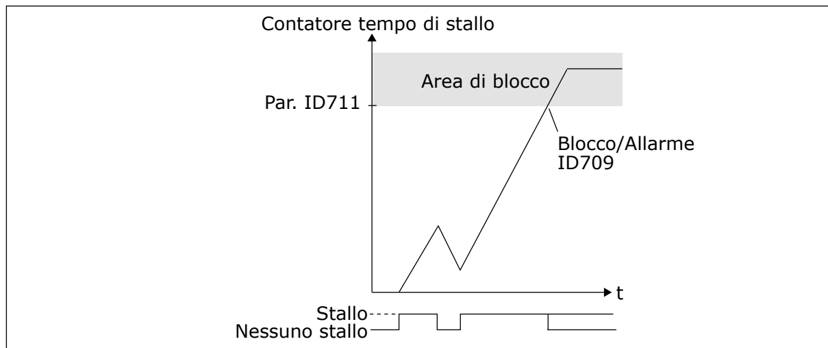
Fig. 75: Calcolo del tempo di stallo
