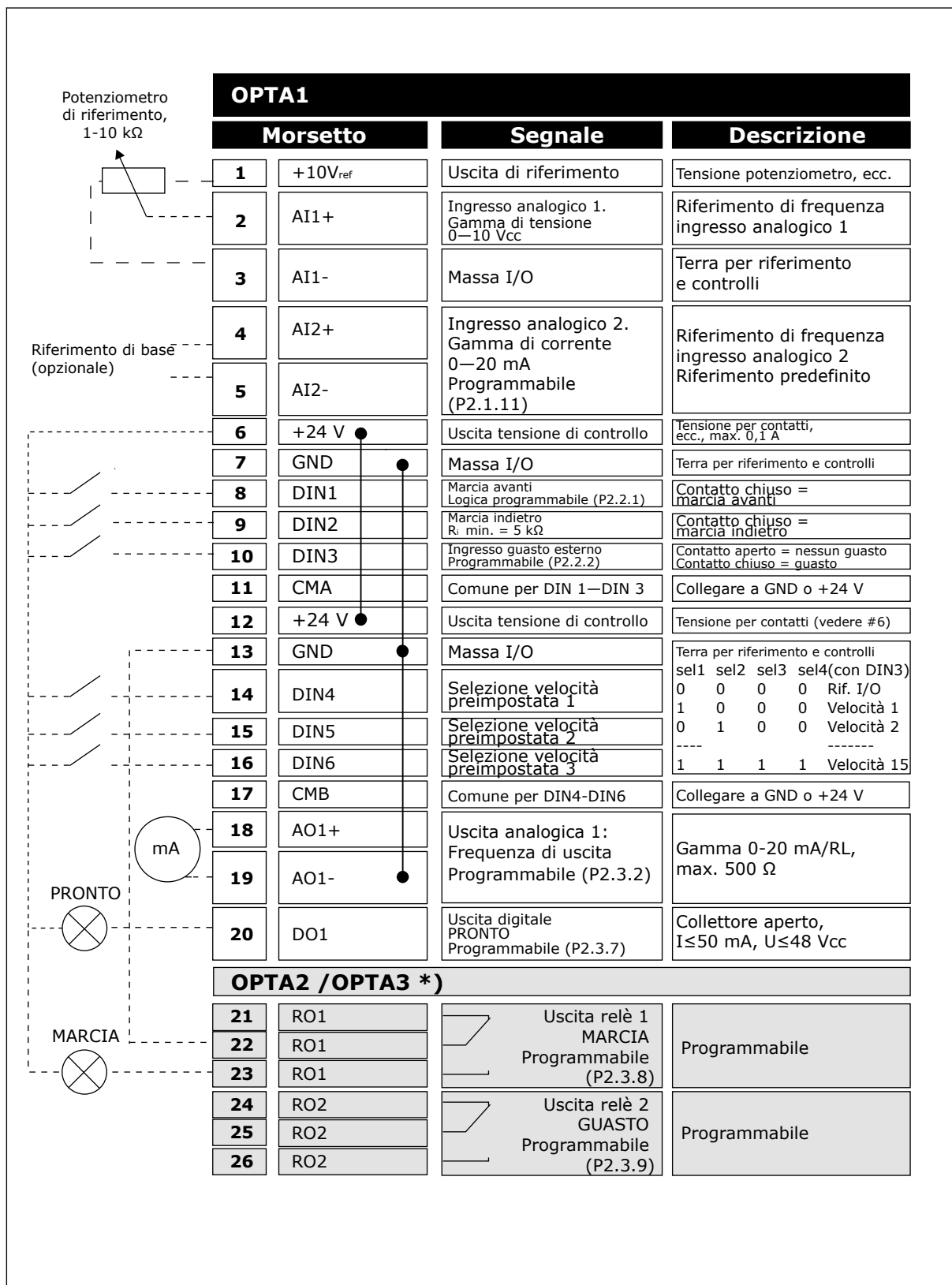
Fig. 10: Configurazione I/O predefinita per l'Applicazione di Controllo della Velocità Multistep
