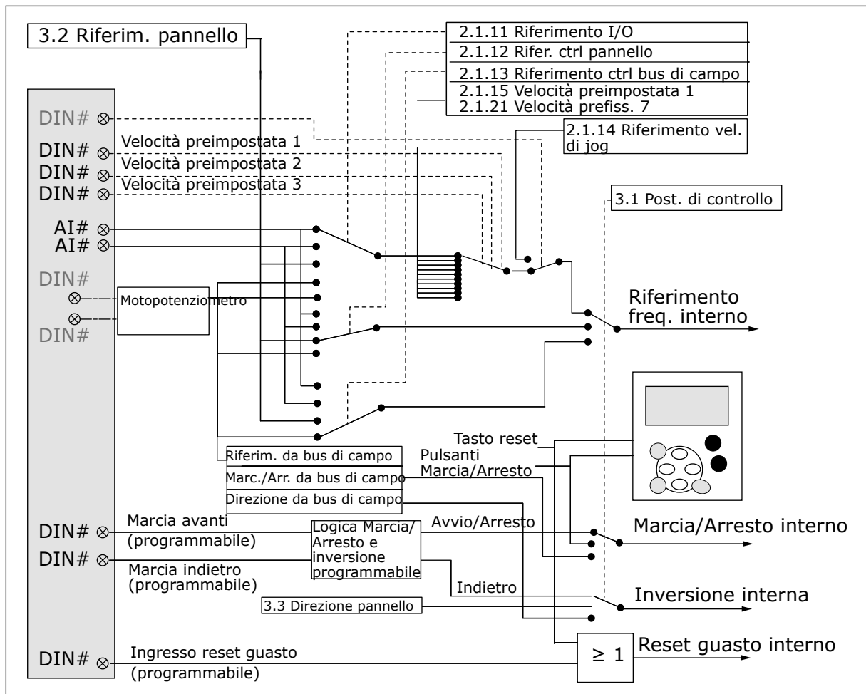
Fig. 18: Logica del segnale di controllo dell'Applicazione di Controllo Multifunzione
