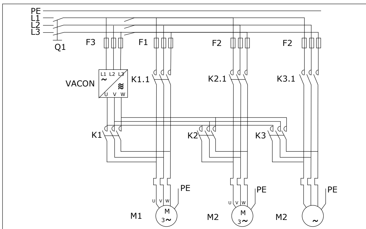
Fig. 99: Esempio di rotazione ausiliari con 3 pompe, schema principale
