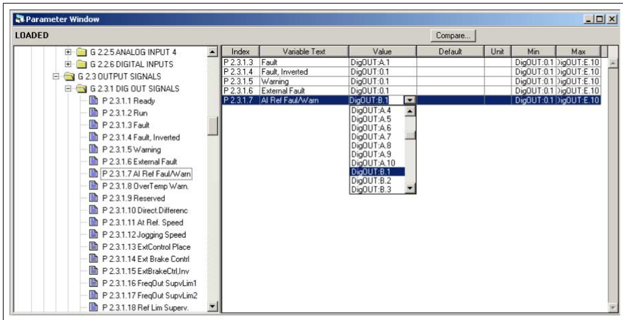
Fig. 95: Schermata dello strumento di programmazione NCDrive: inserimento del codice indirizzo
