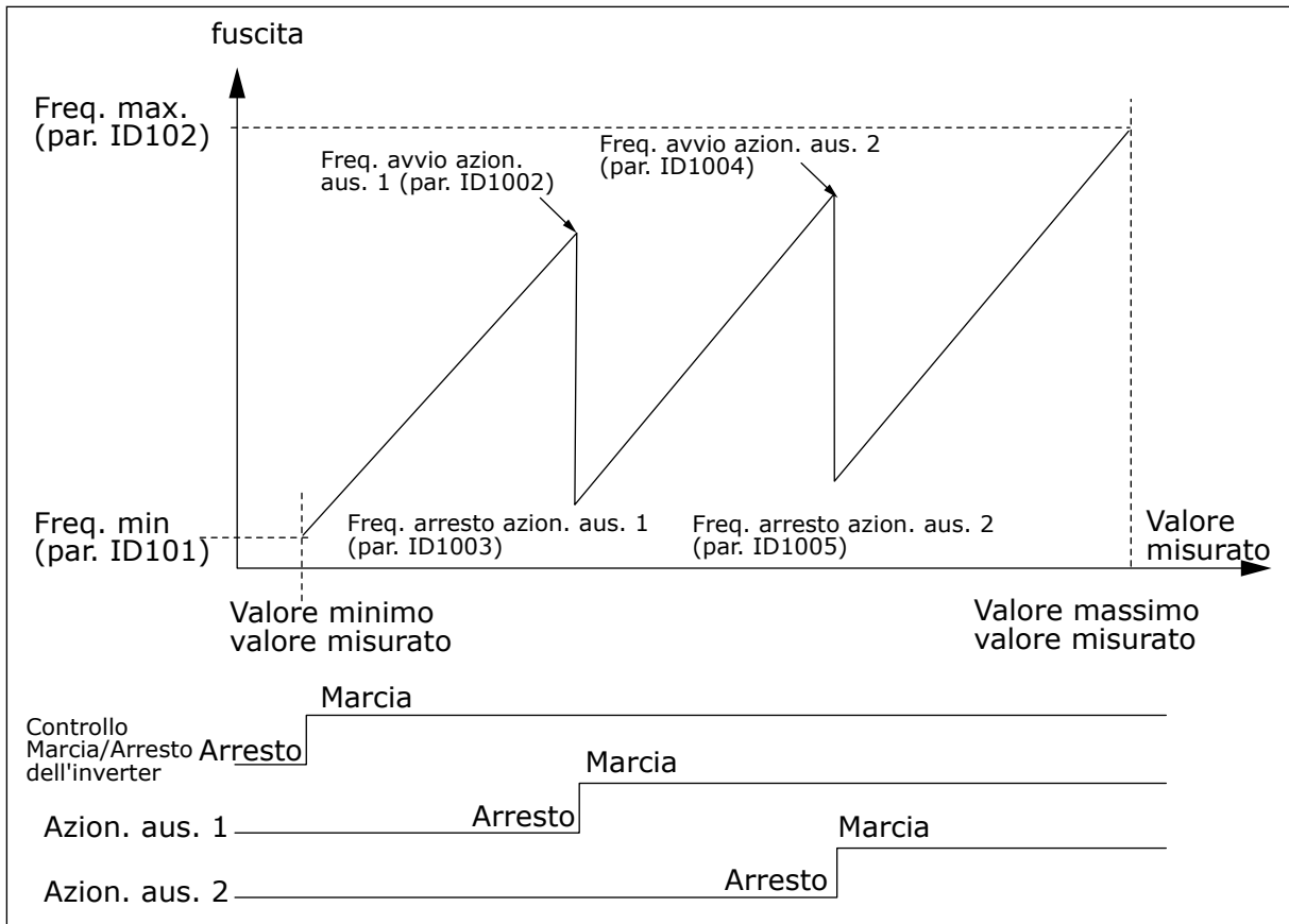
Fig. 82: Esempio di un azionamento a velocità variabile e di due azionamenti ausiliari con controllore PID
