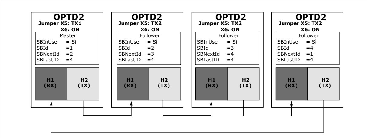
Fig. 91: Collegamenti fisici SystemBus con la scheda OPTD2
