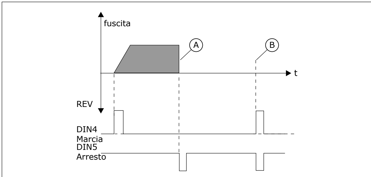
Fig. 56: Impulso di marcia/Impulso di arresto
