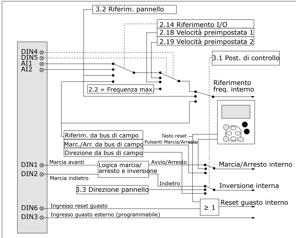
Fig. 3: Logica del segnale di controllo dell'Applicazione Base
