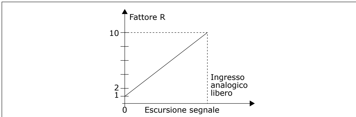
Fig. 52: Riduzione dei tempi di accelerazione e decelerazione
