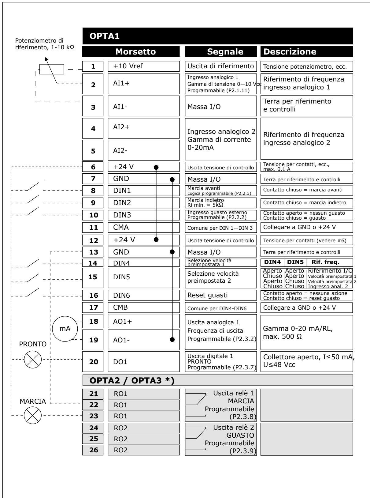
Fig. 4: Configurazione I/O predefinita dell'Applicazione Standard
