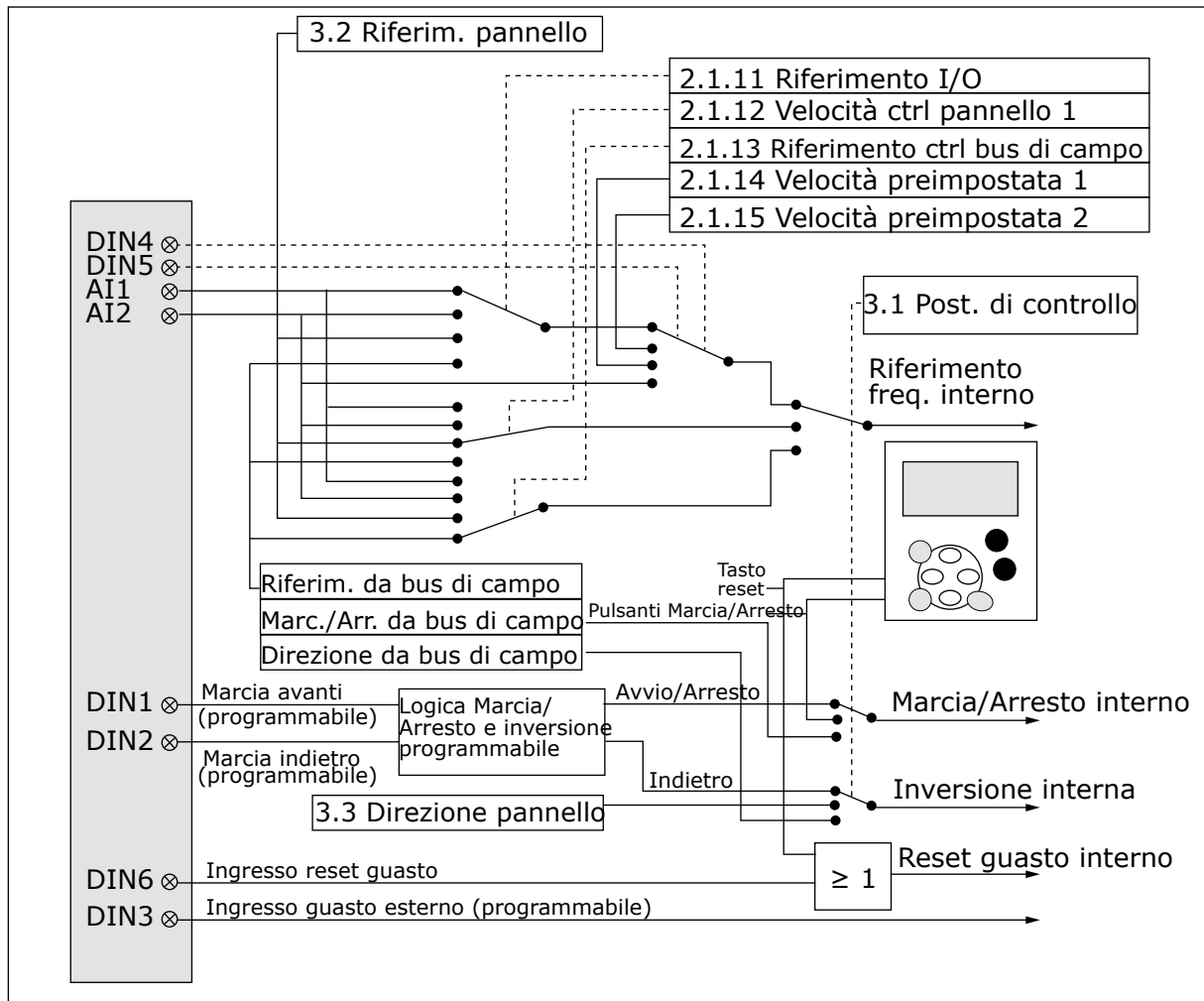
Fig. 6: Logica del segnale di controllo dell'Applicazione Standard
