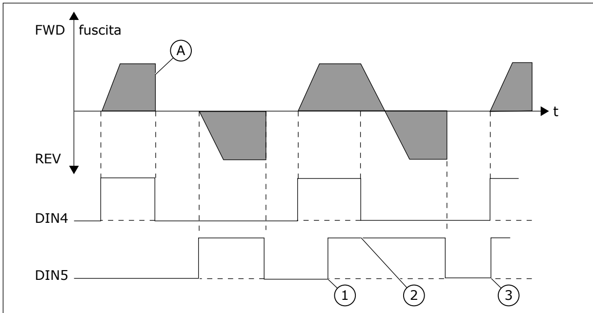
Fig. 54: Marcia avanti/Marcia indietro
