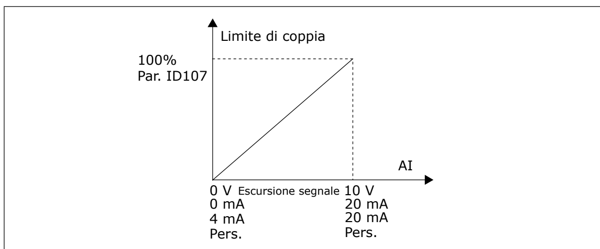
Fig. 50: Scalatura della corrente max. del motore
