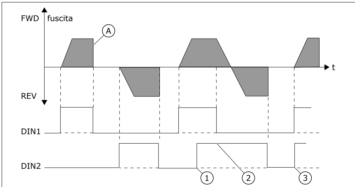
Fig. 30: Marcia avanti/Marcia indietro
