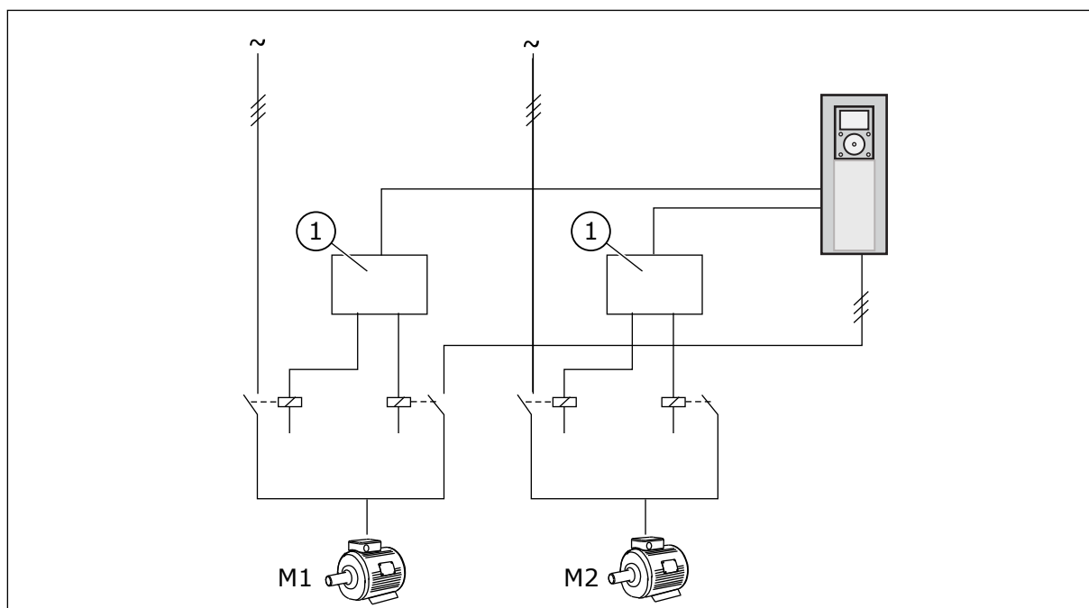
Fig. 87: Rotazione ausiliari con tutti gli azionamenti
