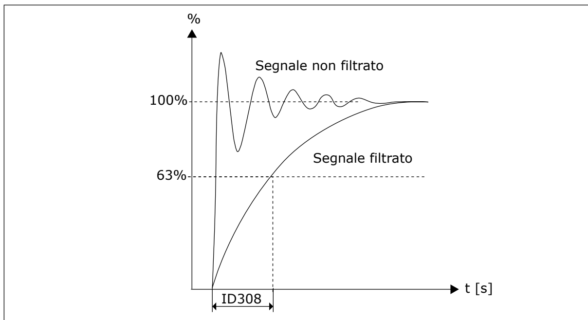
Fig. 37: Filtraggio uscita analogica
