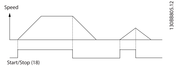
图 8.1 带 Safe Torque Off 的启动/停止
