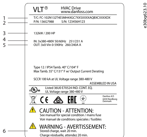
图 4.2 带有选件柜的变频器的铭牌示例（D5h-D8h）
