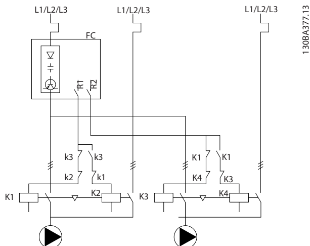
图 8.6 变频泵轮换接线图
