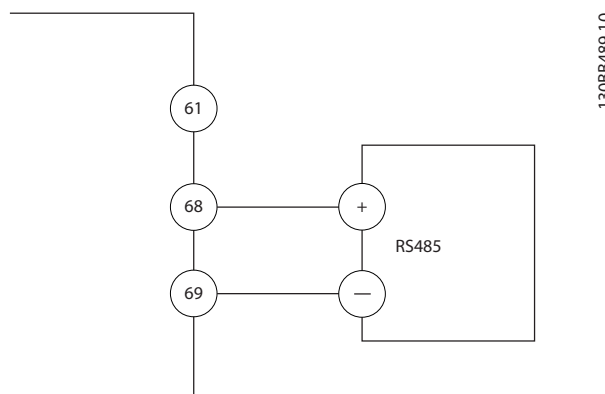
图 5.39 串行通讯接线图
