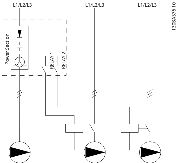
图 8.5 恒速泵/变速泵接线图
