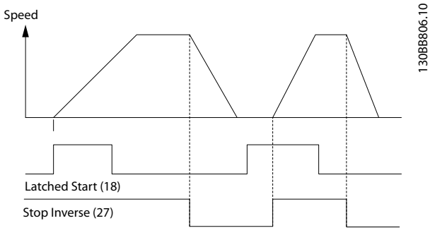
图 8.2 自锁启动/停止反逻辑
