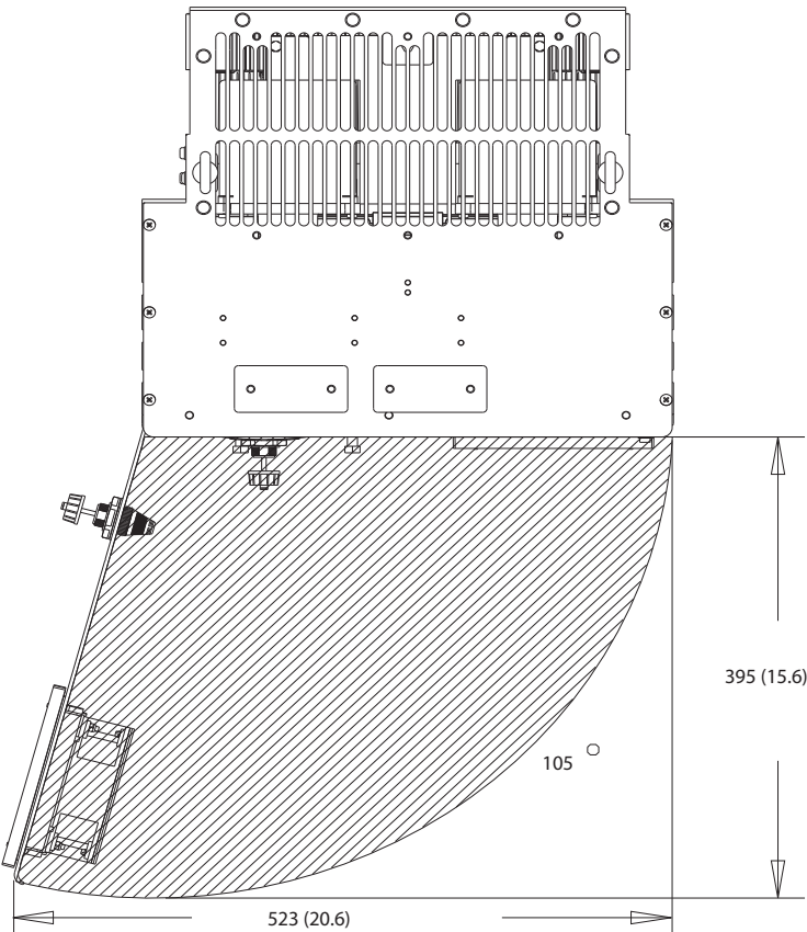
图 10.35 D7h 的门间隙
