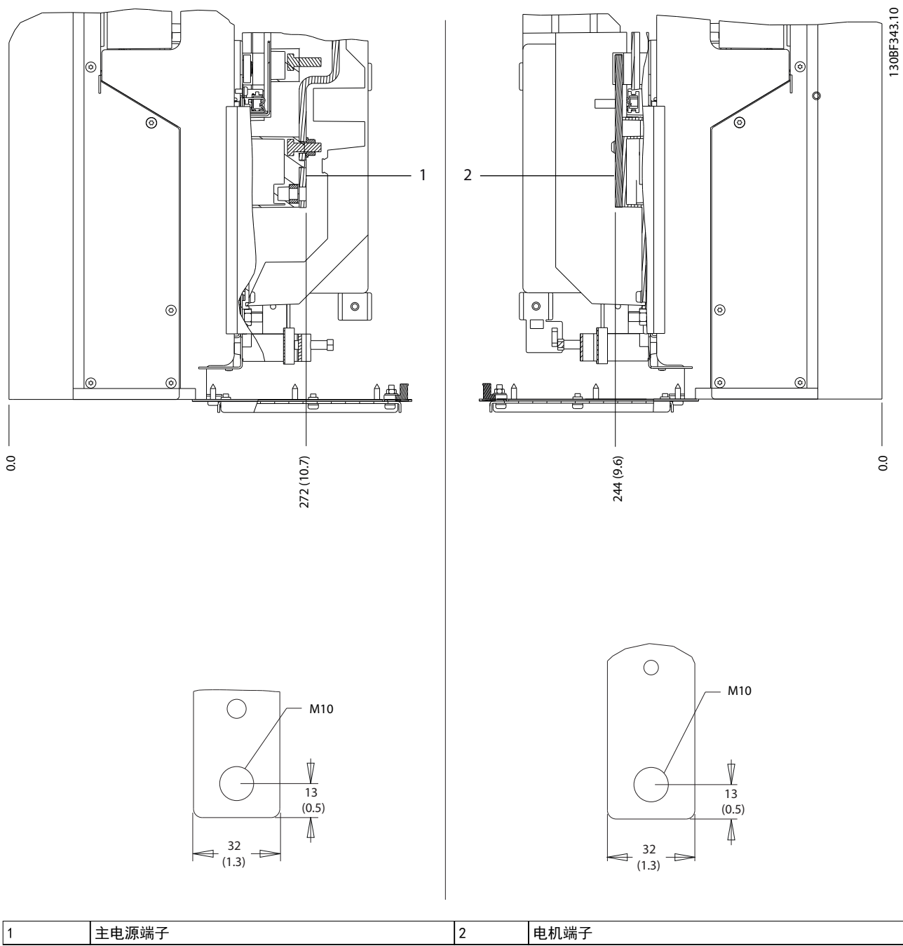
图 5.8 D1h 端子尺寸 (侧视图)
