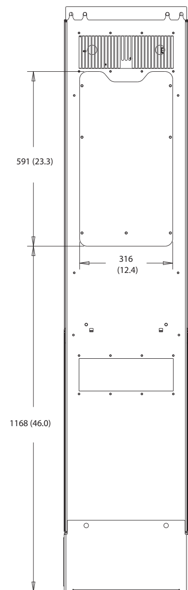
图 10.33 D7h 的散热片气流罩尺寸
