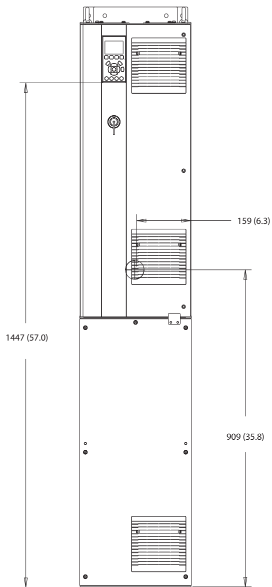
图 10.24 D6h 正视图
