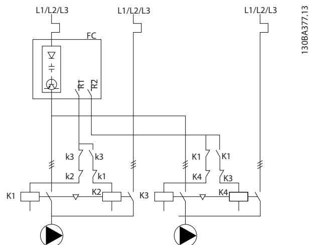
Illustrasjon 8.8 Koplingsskjema for styrepumpealternering
