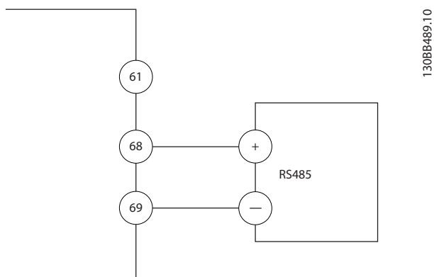
Illustrasjon 5.39 Koplingskjema, seriell kommunikasjon
