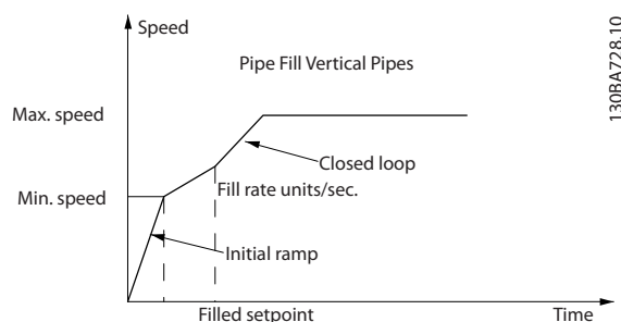
Illustrasjon 8.5 Ytelseskurve for rørfyllingsmodus
