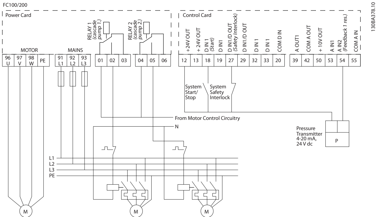
Illustrasjon 8.6 Kablingsskjema, kaskadekontroller
