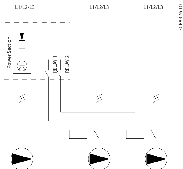
Illustrasjon 8.7 Koplingsskjema for pumpe med konstant variabel hastighet
