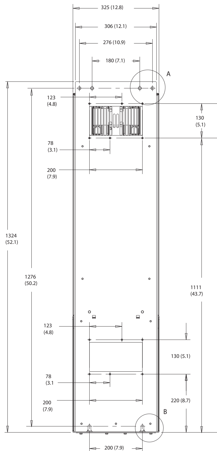
Illustrasjon 10.20 D5h sett bakfra
