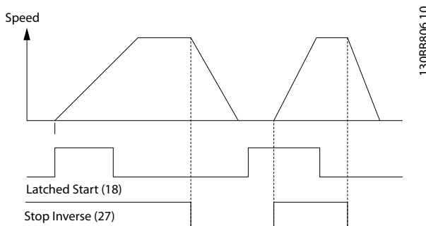
Illustrasjon 8.2 Låst start / stopp invers
