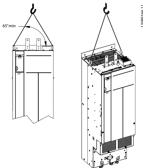
Illustrasjon 4.3 Løfting av omformeren
