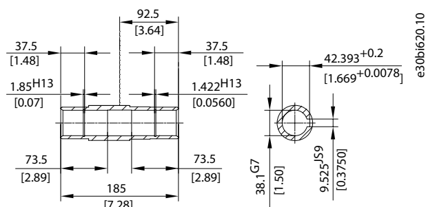
Ilustración 28: Eje I3 de acero/acero inoxidable
