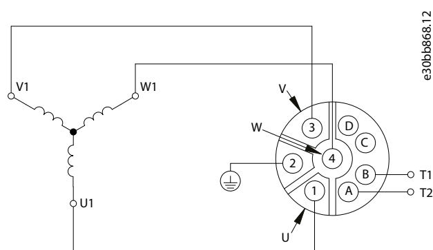
Ilustración 10: Diagrama de conexiones del CleanConnect® para OneGearDrive
