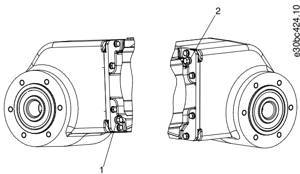
Ilustración 13: Tornillos 1 y 2 del aceite del VLT® OneGearDrive®
