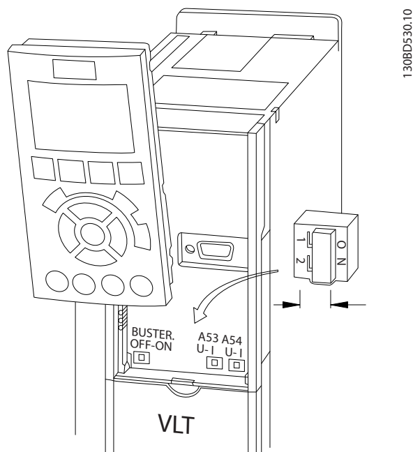
Εικόνα 4.16 Τοποθεσία διακοπών ακροδεκτών 53 και 54
