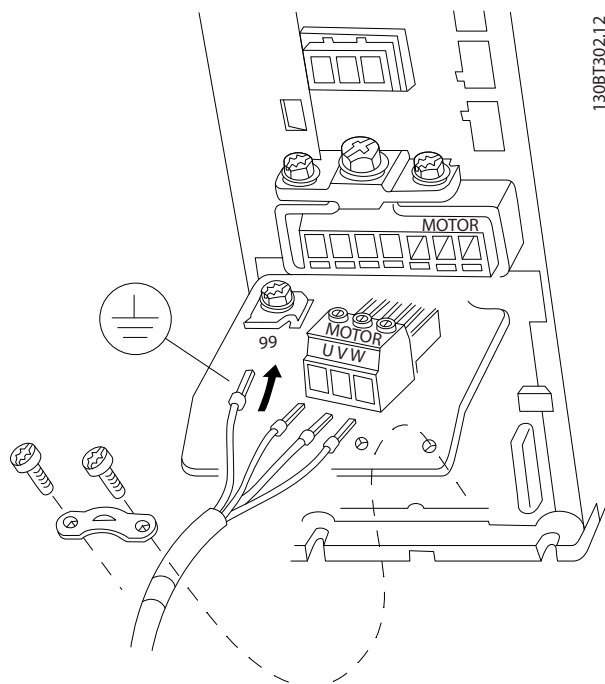
Εικόνα 4.7 Σύνδεση κινητήρα για περίβλημα Τύπου A2 και A3
