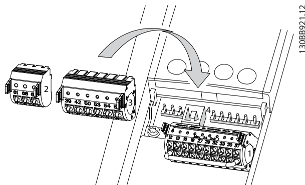
Εικόνα 4.13 Θέσεις ακροδεκτών ελέγχου
