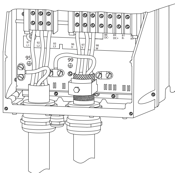
Εικόνα 4.11 Καλωδίωση κινητήρα, δικτύου ρεύματος και γείωσης για περιβλήματα τύπου B και C, με τη χρήση θωρακισμένου καλωδίου
