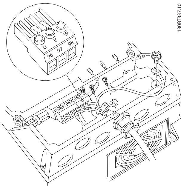
Ilustrasi 4.7 Sambungan Motor untuk jenis penutup A4/A5 (IP55/66/NEMA jenis 12)
