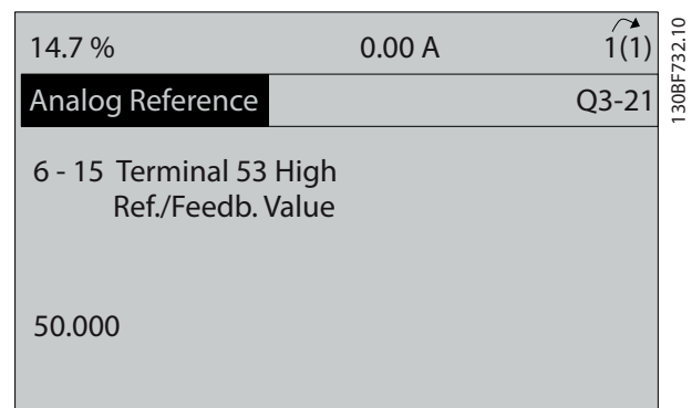
Illustration 6.11 Paramètre 6-15 Val.ret./Réf.haut.born.53
