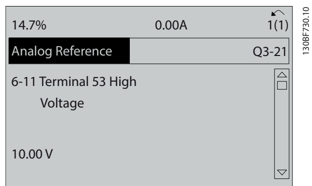
Illustration 6.9 Paramètre 6-11 Ech.max.U/born.53
