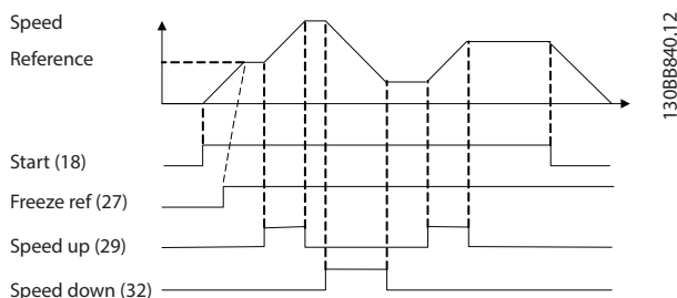
图 8.3 加速/减速
