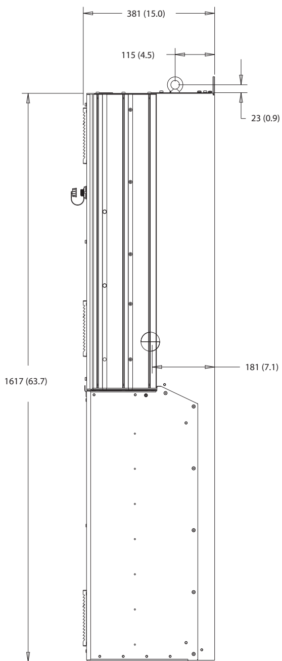
图 10.25 D6h 侧视图
