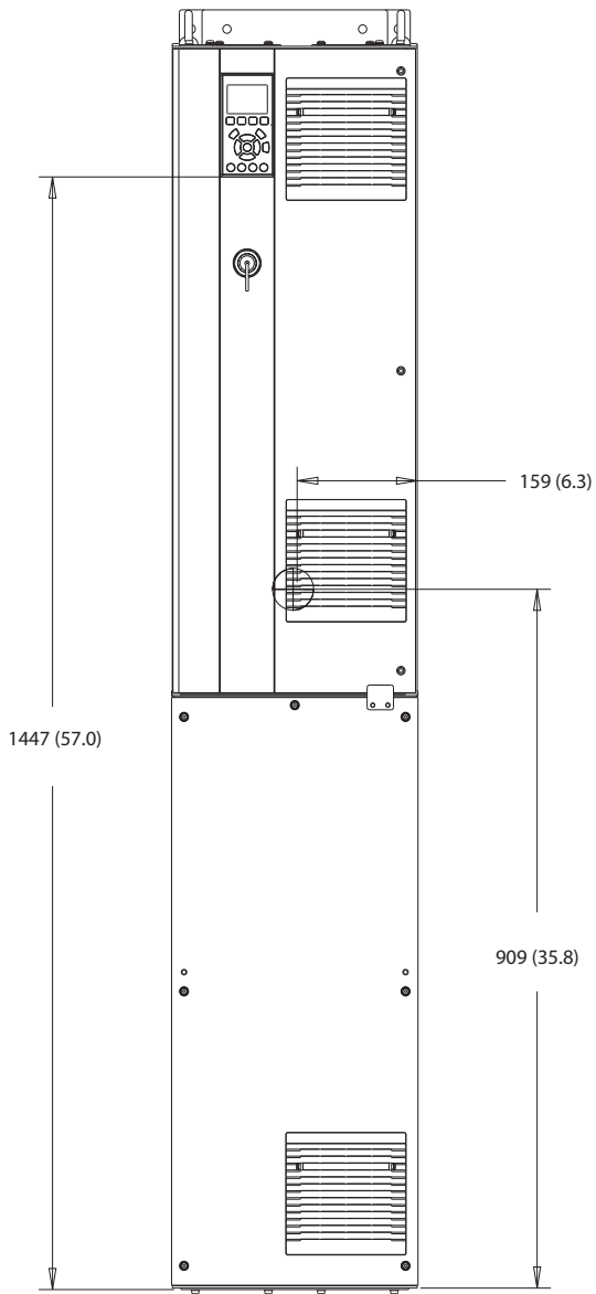
图 10.24 D6h 正视图
