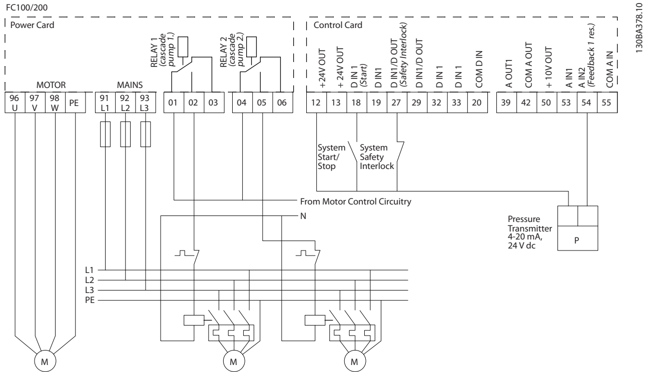
图 8.6 多泵控制器接线图
