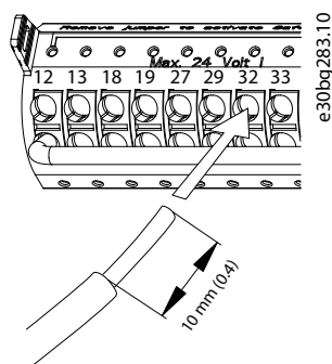
Ilustrația 5.19 Conectarea conductorilor de control solizi
