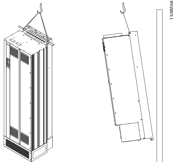
Ilustrația 4.2 Metodă de ridicare recomandată
