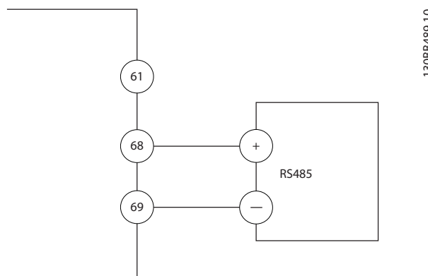
Ilustrația 5.21 Diagrama de cablare pentru comunicația serială
