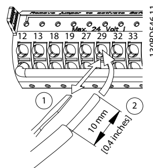
Ilustrația 5.20 Conectarea conductorilor de control flexibili
