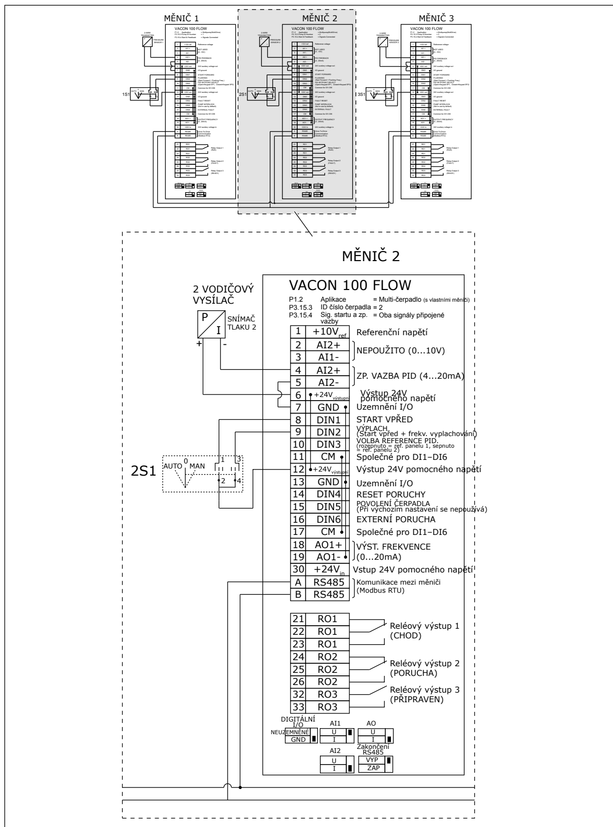
Obr. 19: Schéma elektrického zapojení systému multi-čerpadla (s vlastními měniči), příklad 1B
