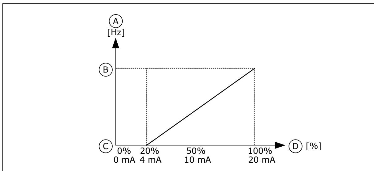
Obr. 58: Rozsah analogového vstupního signálu, volba 1
