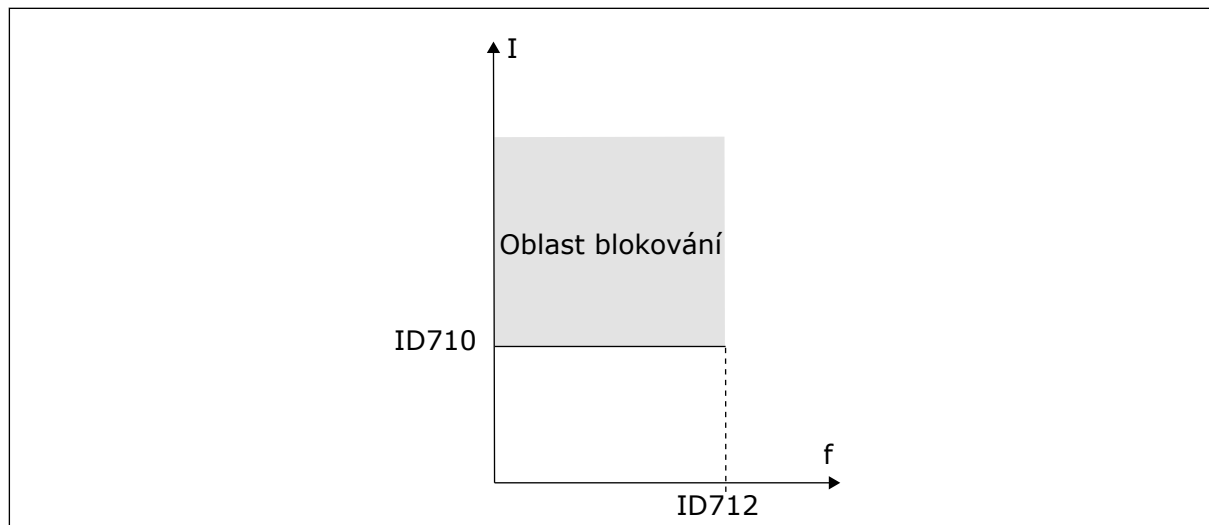
Obr. 68: Nastavení charakteristik zablokování
