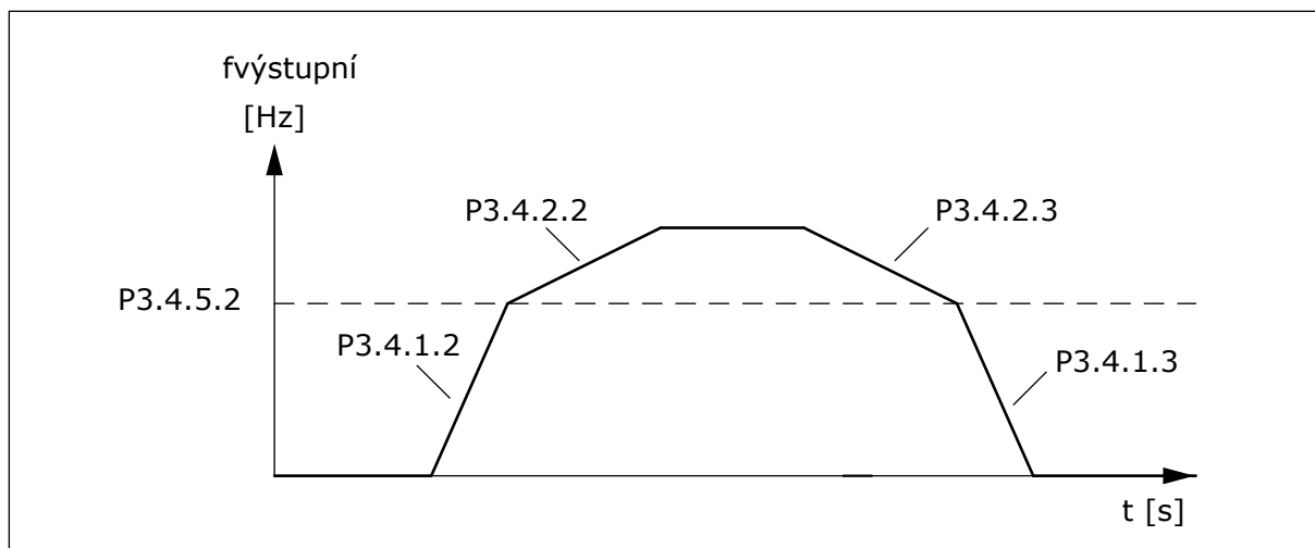
Obr. 50: Rampa 2 se aktivuje tehdy, jestliže výstupní frekvence překročí prahovou úroveň. (P. 3.4.5.2 = Prahová frekvence rampy, P3.4.1.2 = Doba rozběhu 1, P3.4.2.2 = Doba rozběhu 2, P3.4.1.3 = Doba doběhu 1, P3.4.2.3 = Doba doběhu 2)
