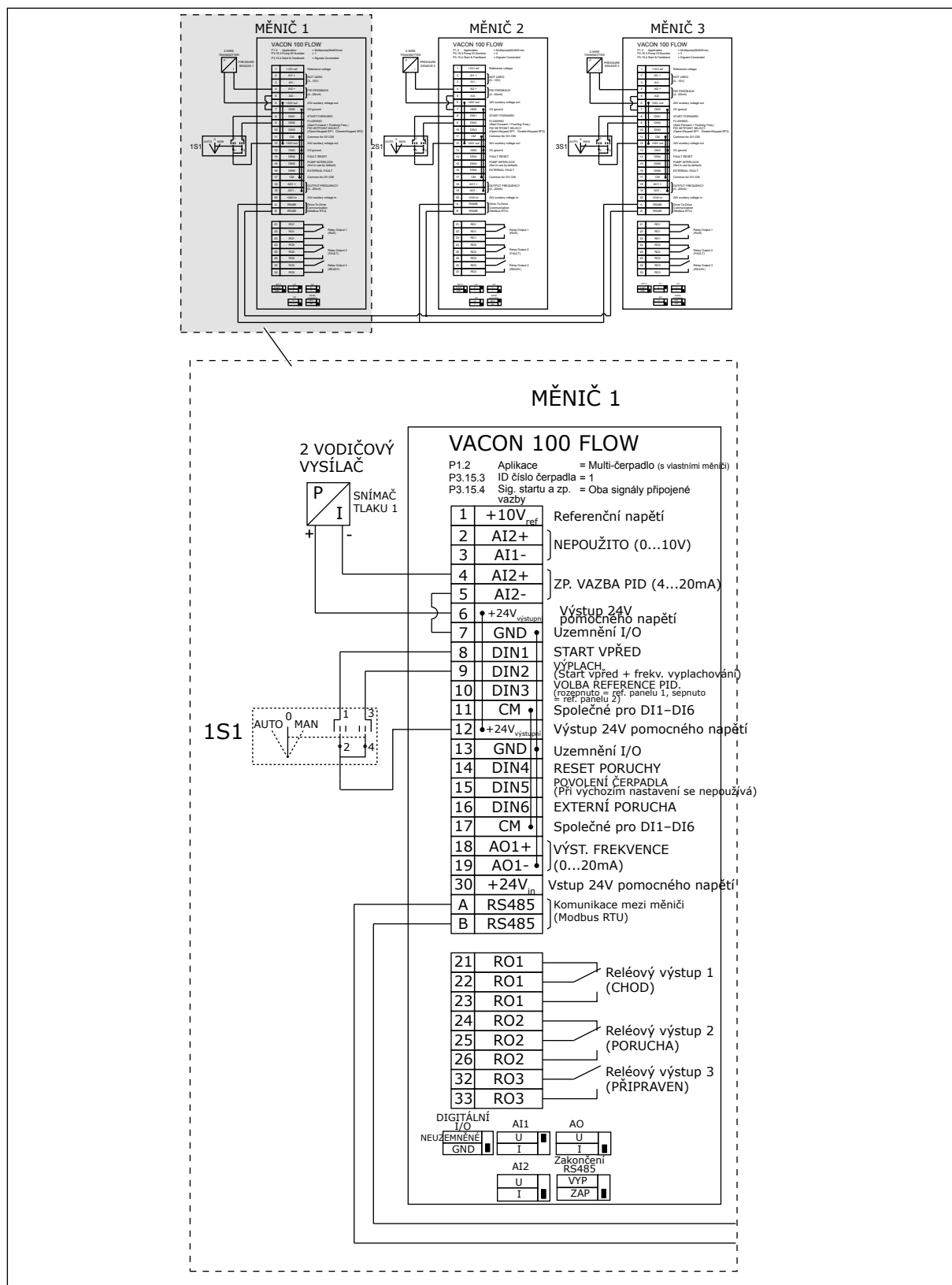
Obr. 18: Schéma elektrického zapojení systému multi-čerpadla (s vlastními měniči), příklad 1A
