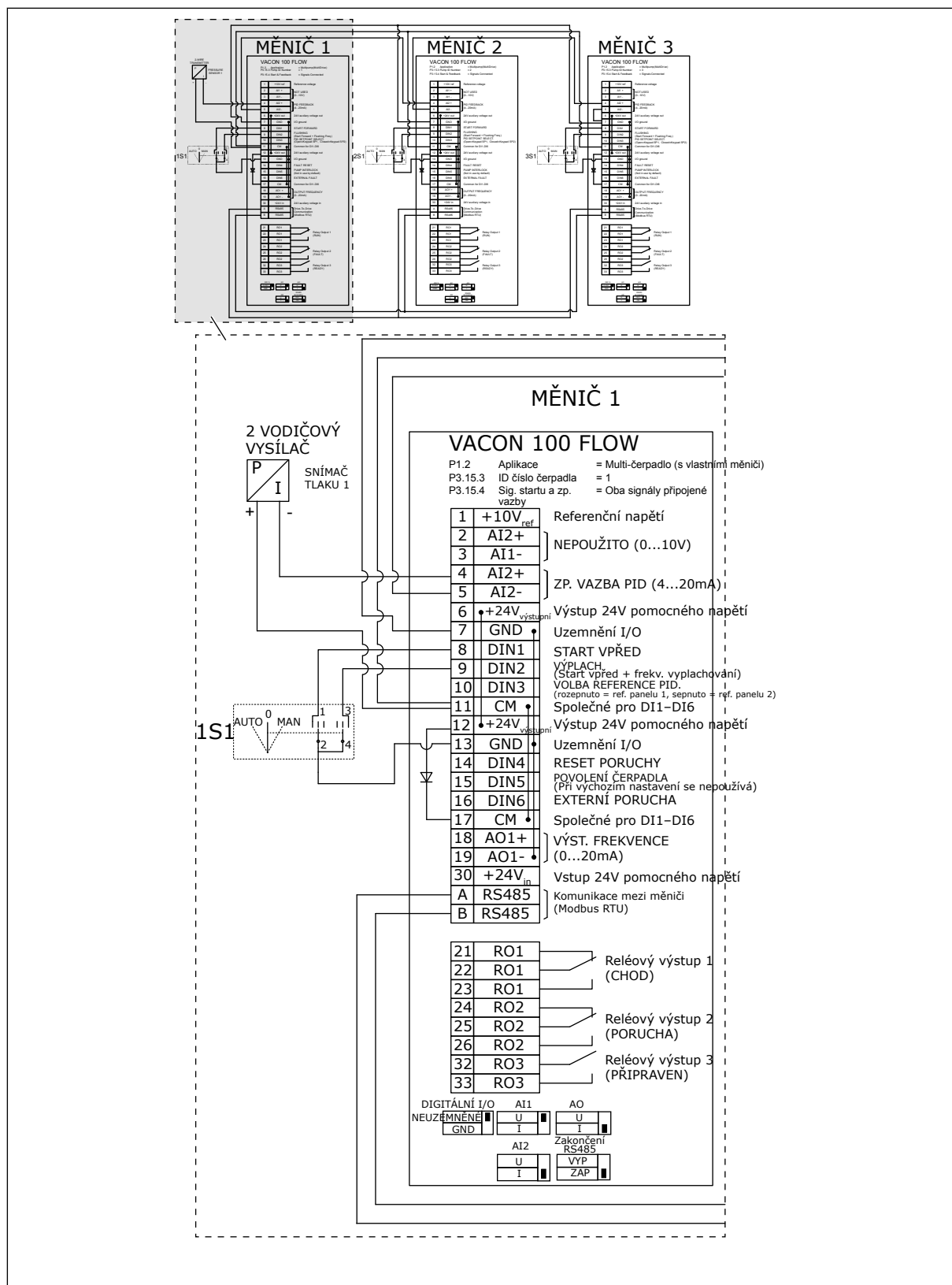
Obr. 21: Schéma elektrického zapojení systému multi-čerpadla (s vlastními měniči), příklad 2A
