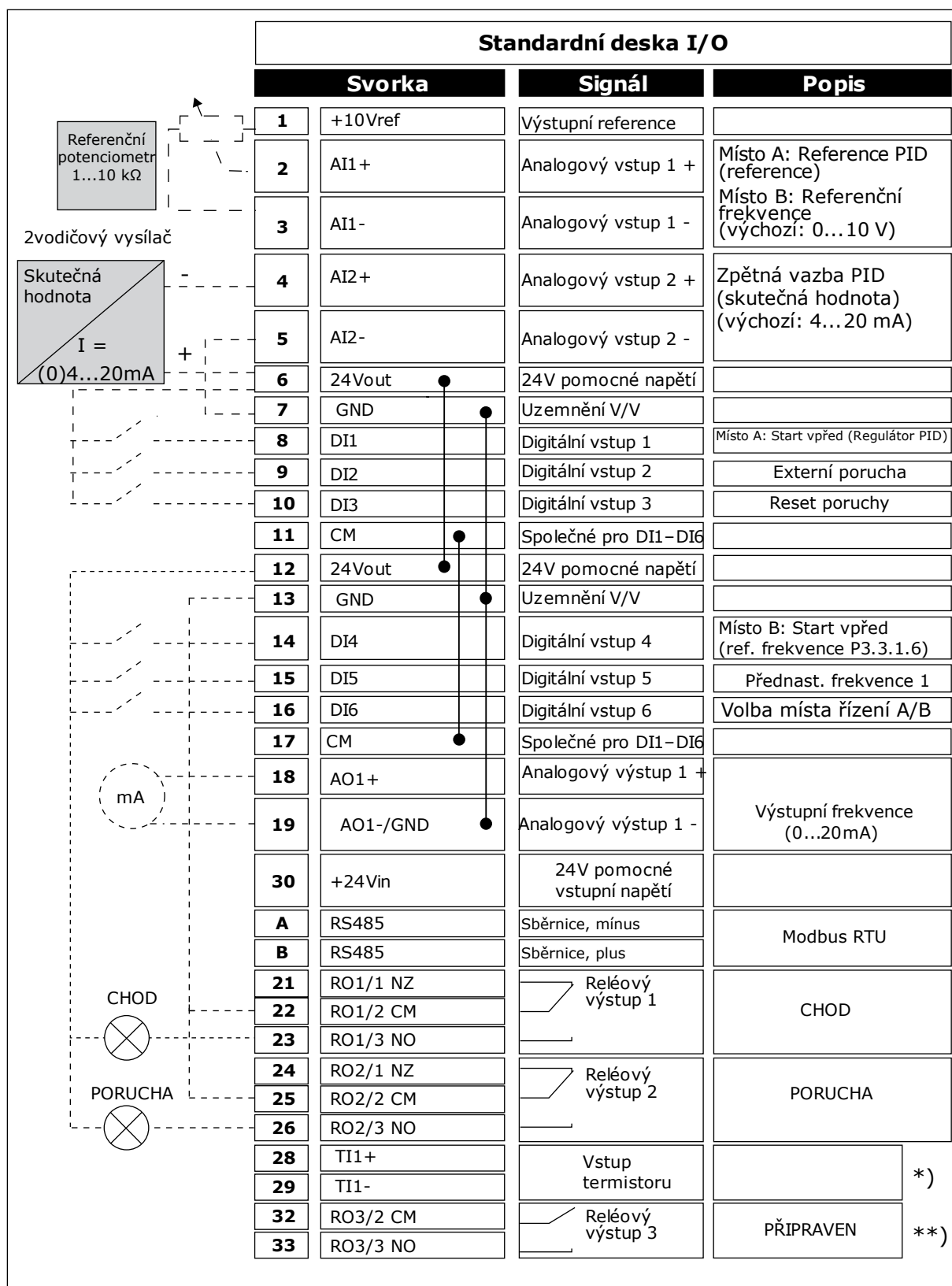
Obr. 6: Výchozí připojení řízení v aplikaci PID řízení
