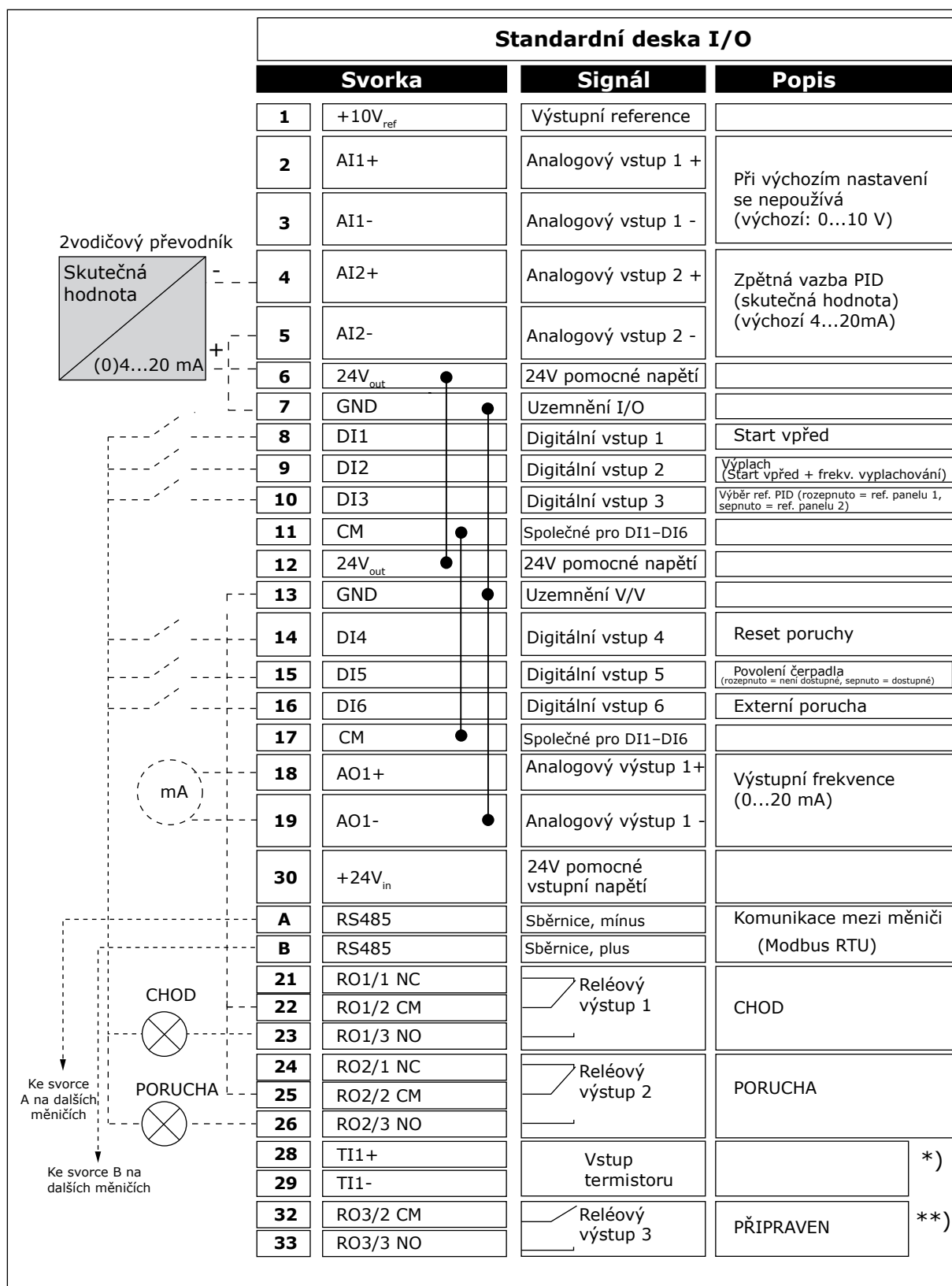
Obr. 16: Výchozí připojení řízení v aplikaci multi-čerpadla (s vlastními měniči)
