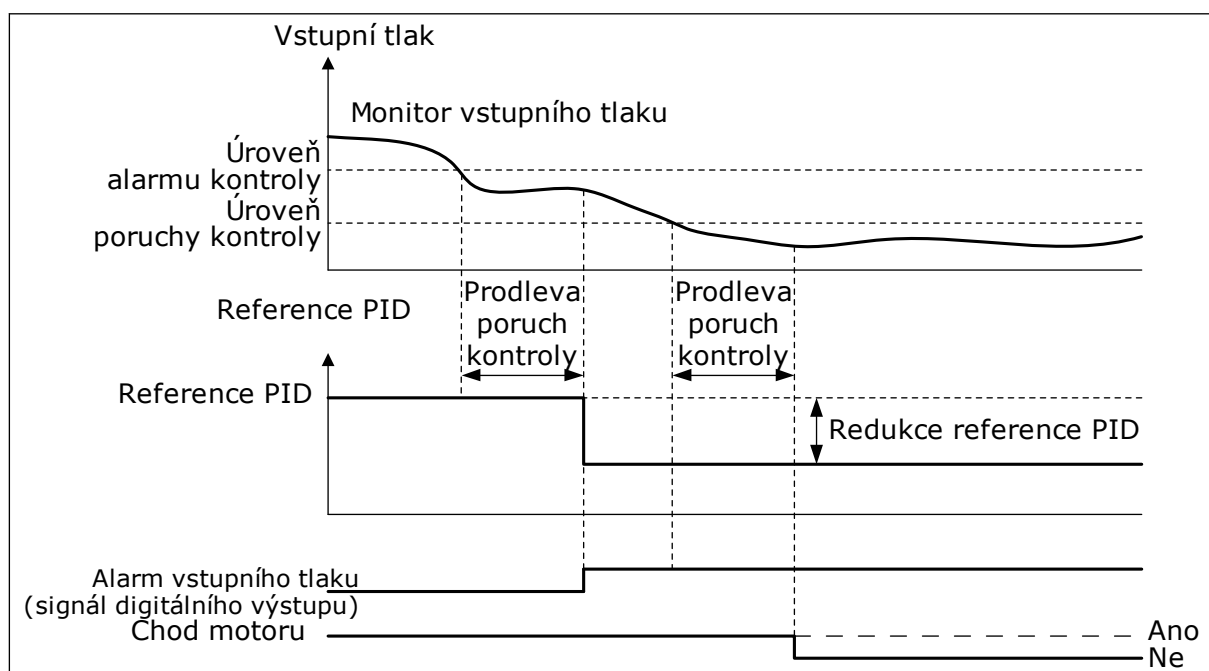
Obr. 87: Funkce kontroly vstupního tlaku
