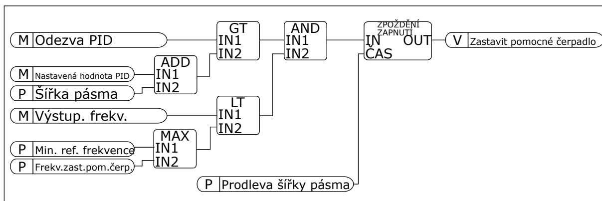
Obr. 102: Frekv.zast.pom.čerp.
