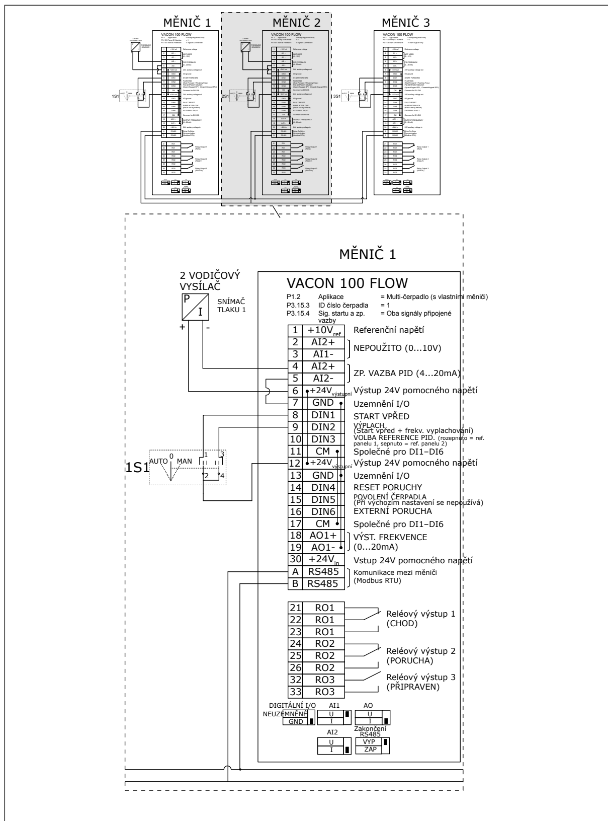
Obr. 25: Schéma elektrického zapojení systému multi-čerpadla (s vlastními měniči), příklad 3B
