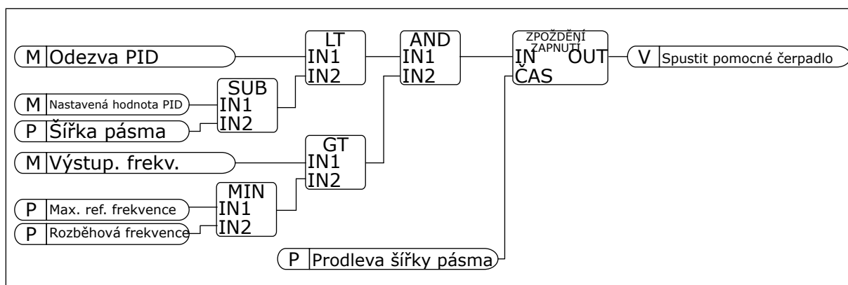
Obr. 101: Frekv.star.pom.čerp.
