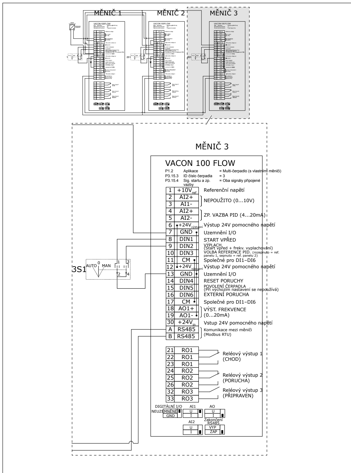
Obr. 29: Schéma elektrického zapojení systému multi-čerpadla (s vlastními měniči), příklad 4C
