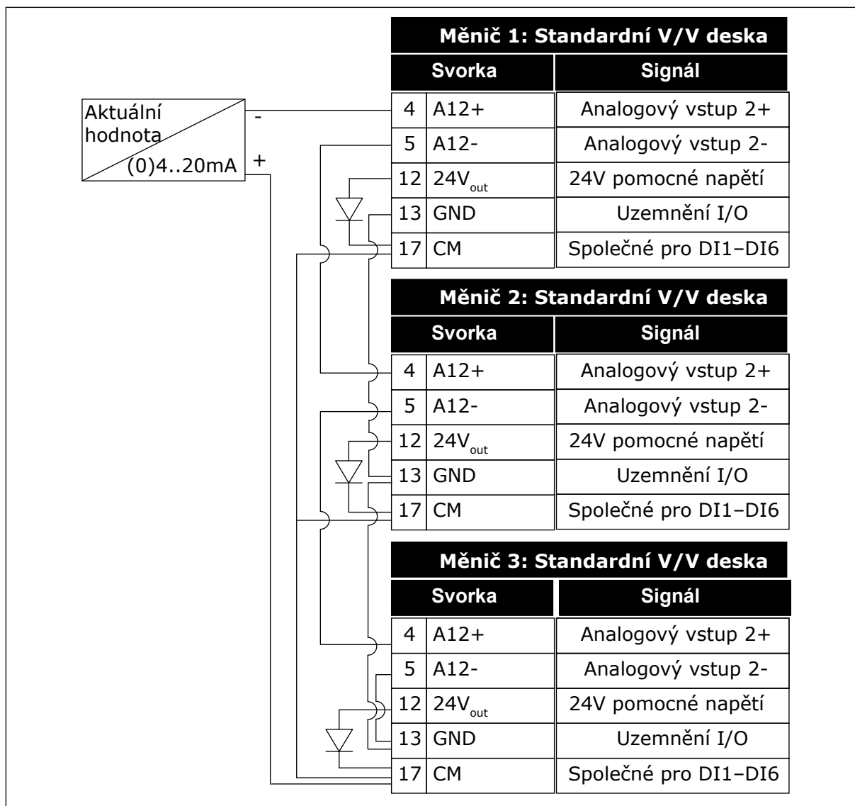
Obr. 95: Zapojení společného snímače pro všechny měniče (napájeného z desky I/O měniče)
