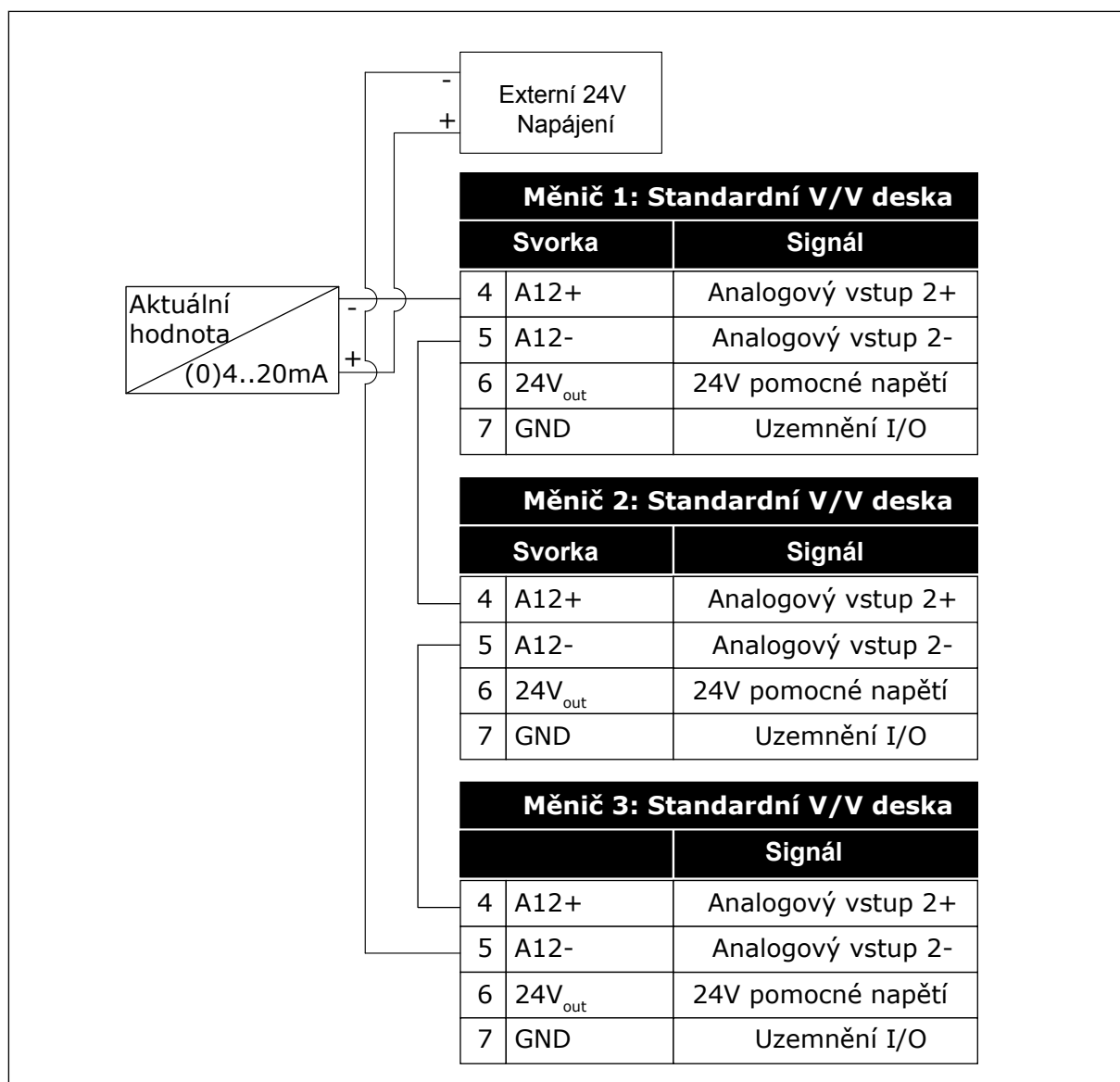
Obr. 96: Zapojení společného snímače pro všechny měniče (napájeného z externího 24V zdroje)
