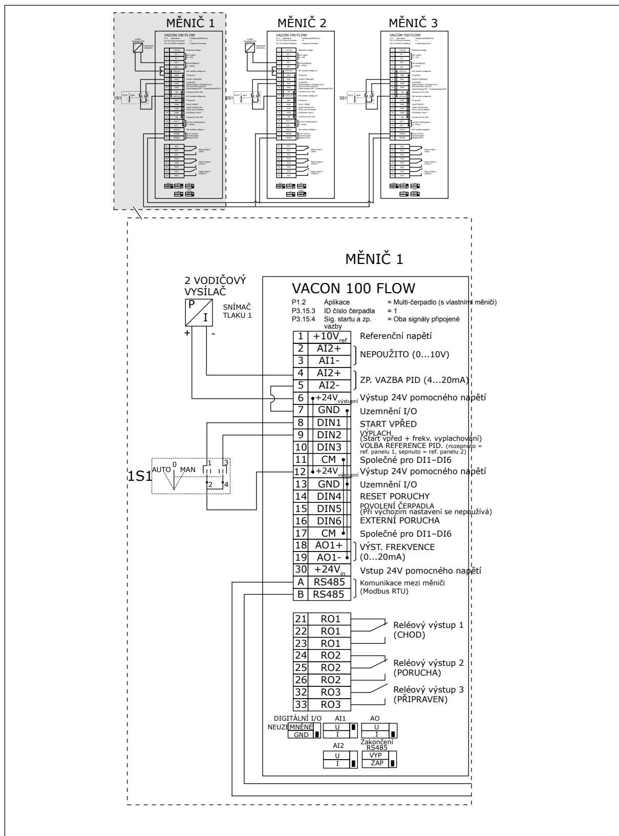
Obr. 24: Schéma elektrického zapojení systému multi-čerpadla (s vlastními měniči), příklad 3A
