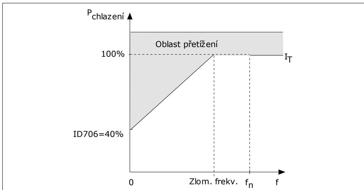
Obr. 65: Křivka tepelného proudu motoru I_T
