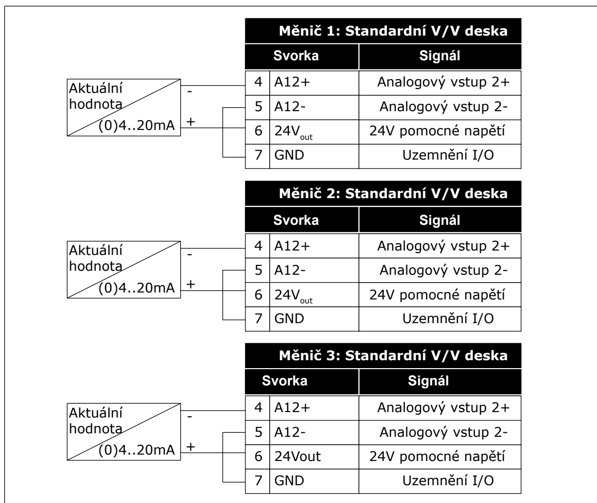
Obr. 94: Zapojení snímače zpětné vazby pro každý měnič
