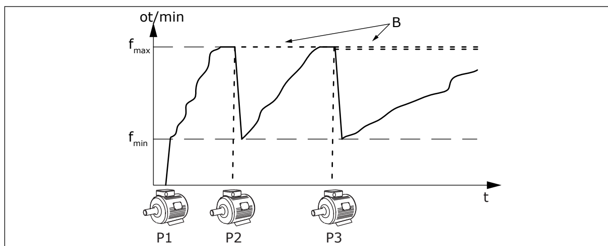
Obr. 91: Řízení v režimu se společným měničem
