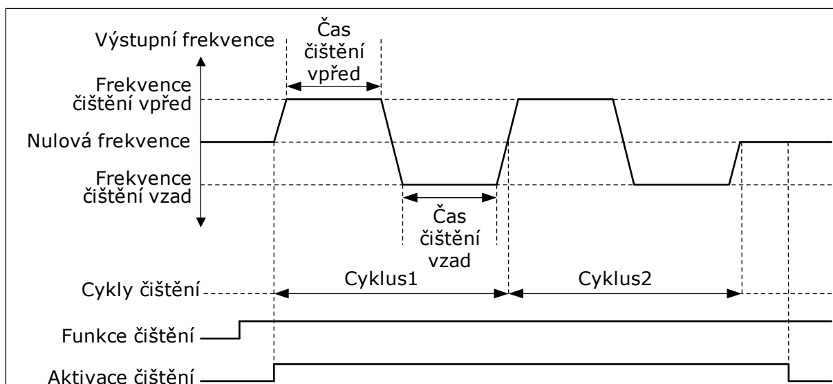
Obr. 104: Funkce automatického čištění
