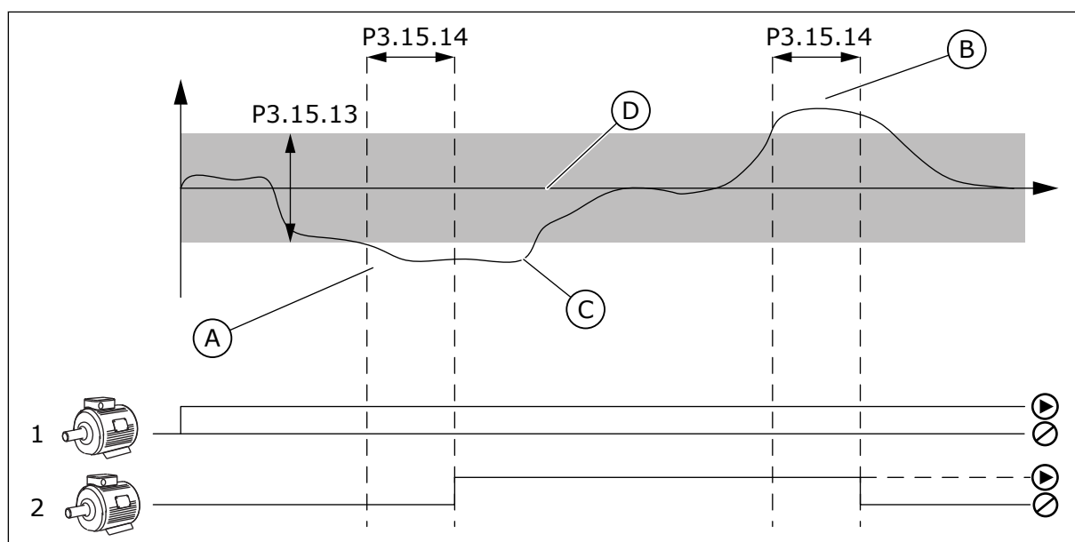
Obr. 99: Spouštění a zastavování pomocných čerpadel (P3.15.13 = Šířka pásma, P3.15.14 = Prodleva mimo pásmo)
