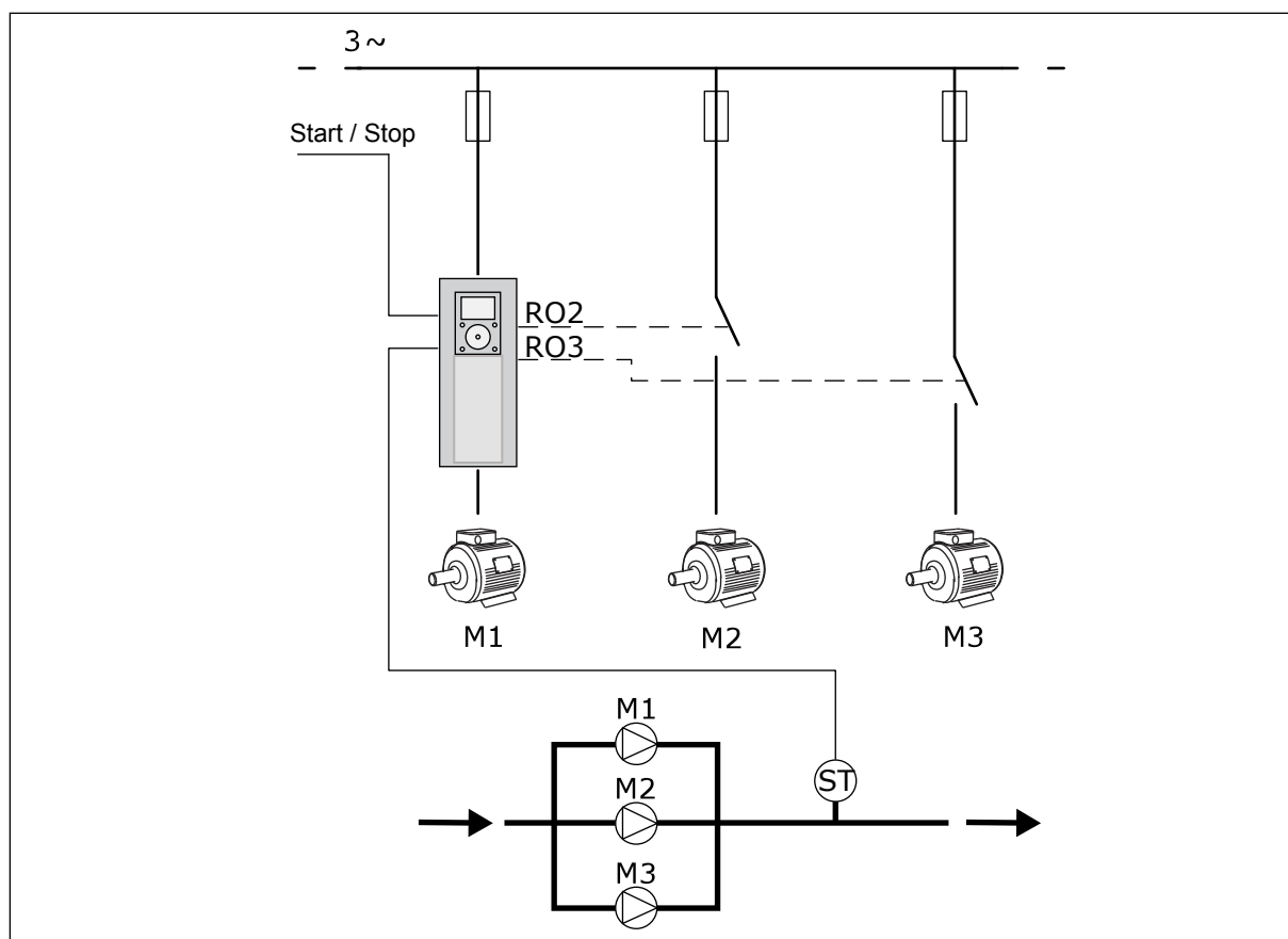
Obr. 8: Konfigurace multi-čerpádky (se samostatným měničem)
