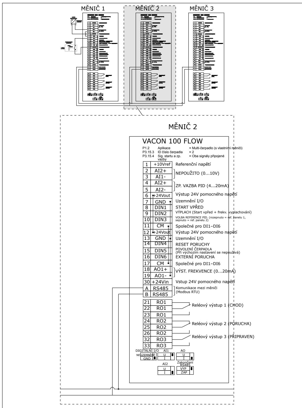
Obr. 31: Schéma elektrického zapojení systému multi-čerpadla (s vlastními měniči), příklad 5B
