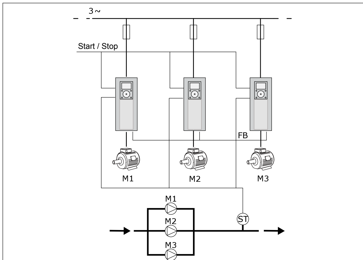
Obr. 13: Konfigurace multi-čerpadla (s vlastními měniči)
