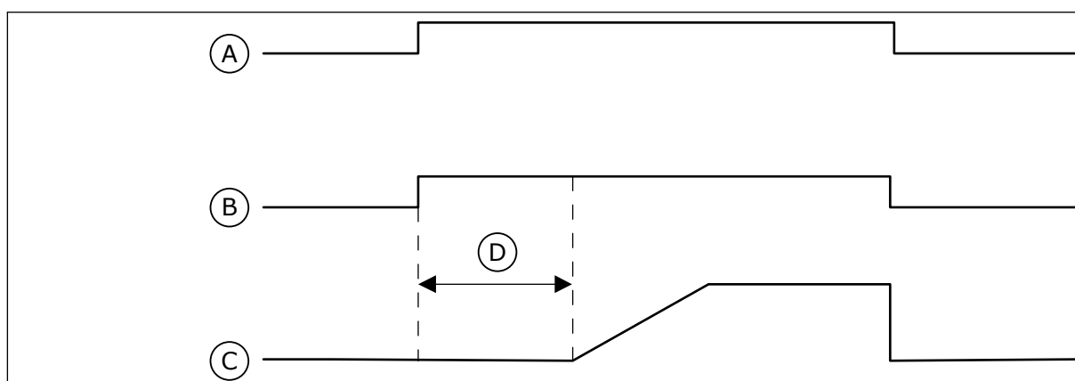
Obr. 106: Funkce plnicího čerpadla
