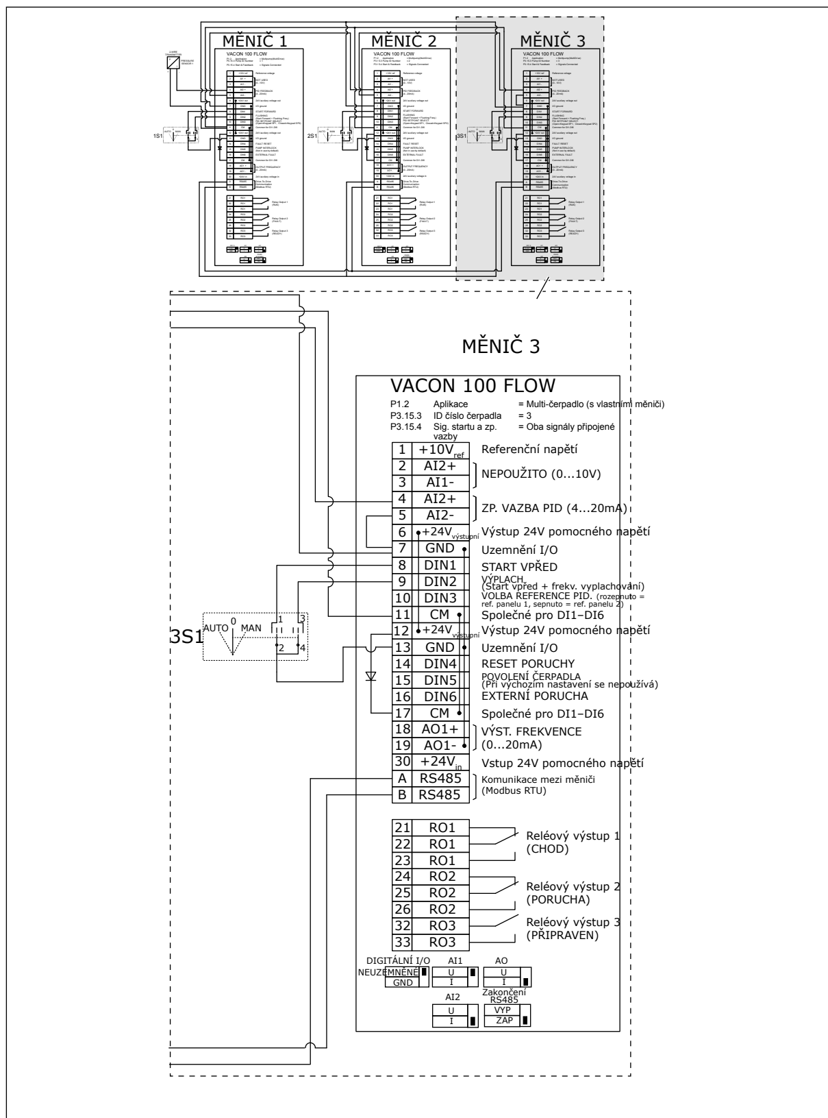
Obr. 23: Schéma elektrického zapojení systému multi-čerpadla (s vlastními měniči), příklad 2C
