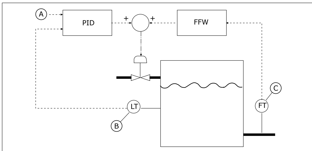
Obr. 80: Dopředná regulace
