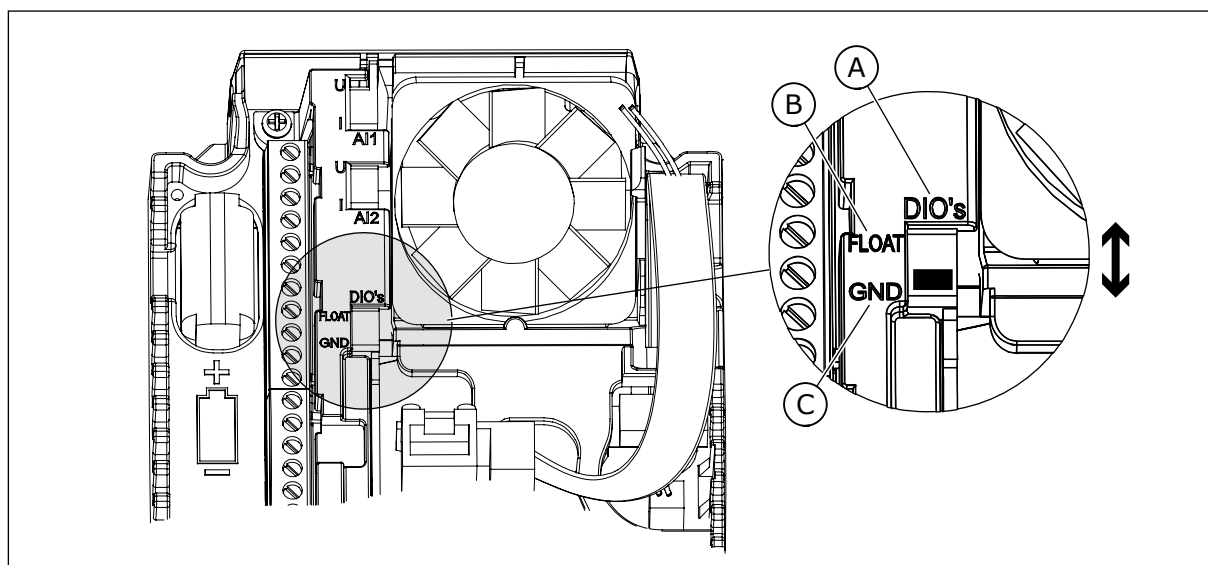
Obr. 5: Dvupolohový přepínač
