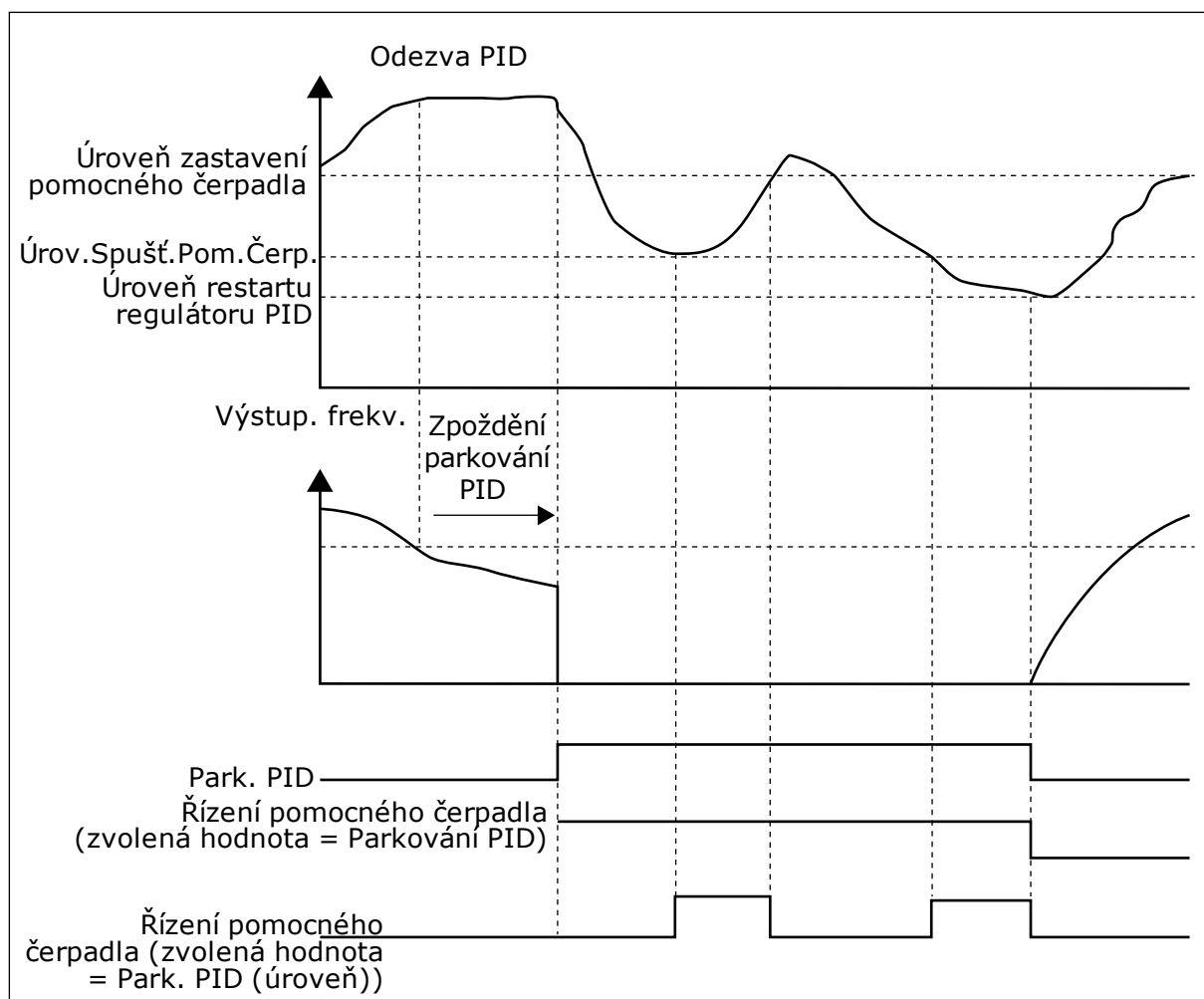
Obr. 105: Funkce pomocného čerpadla
