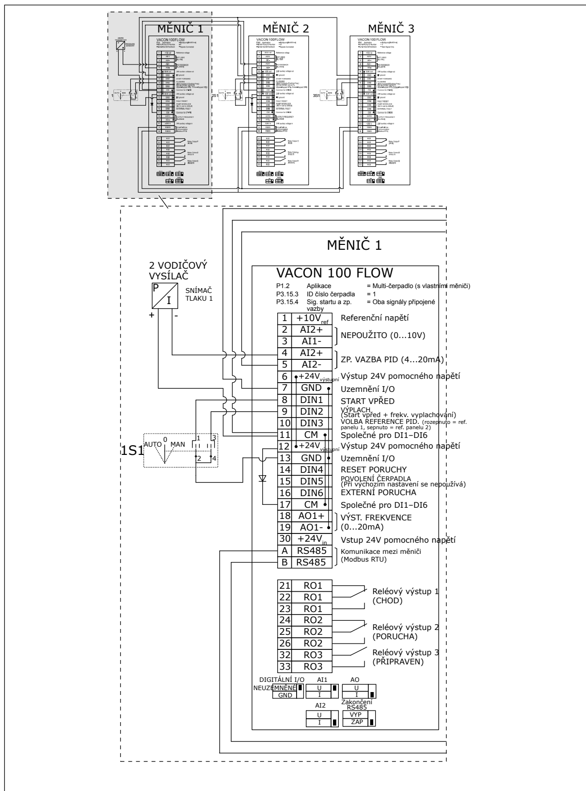
Obr. 27: Schéma elektrického zapojení systému multi-čerpadla (s vlastními měniči), příklad 4A
