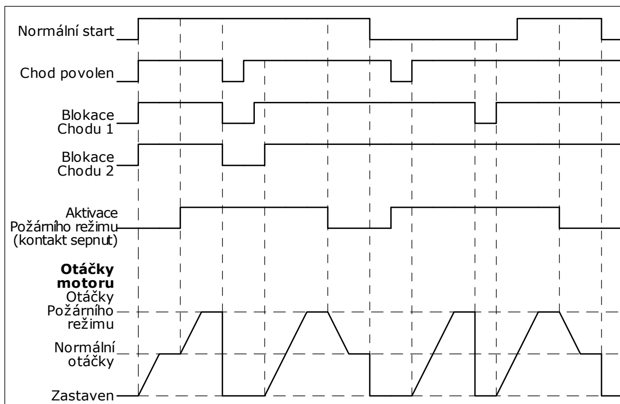
Obr. 103: Funkce požárního režimu
