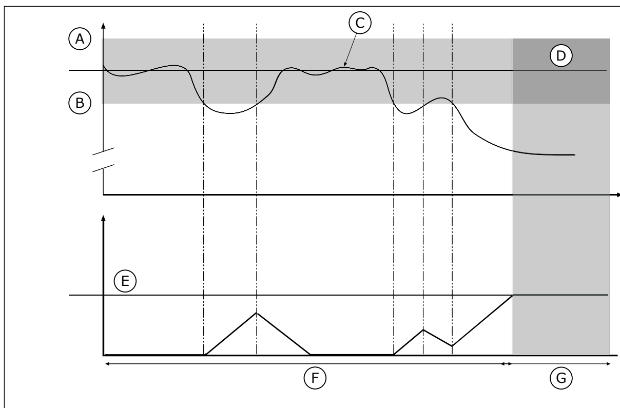
Obr. 83: Funkce kontroly zpětné vazby
