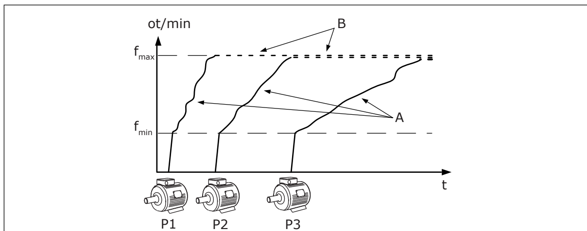
Obr. 93: Řízení v režimu Multimaster
