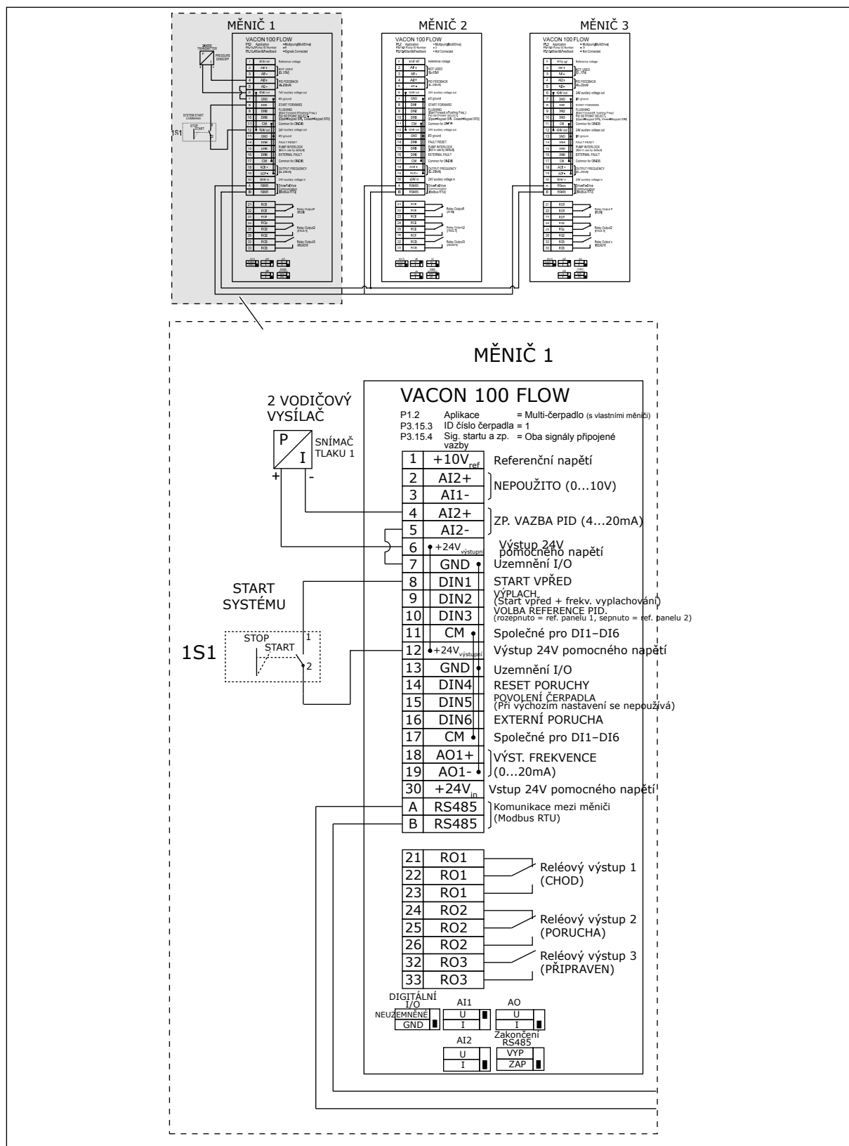
Obr. 30: Schéma elektrického zapojení systému multi-čerpadla (s vlastními měniči), příklad 5A
