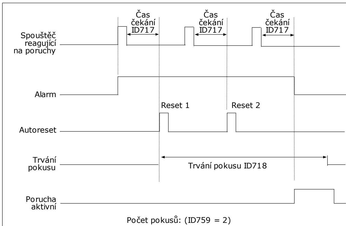
Obr. 72: Funkce automatického resetu
