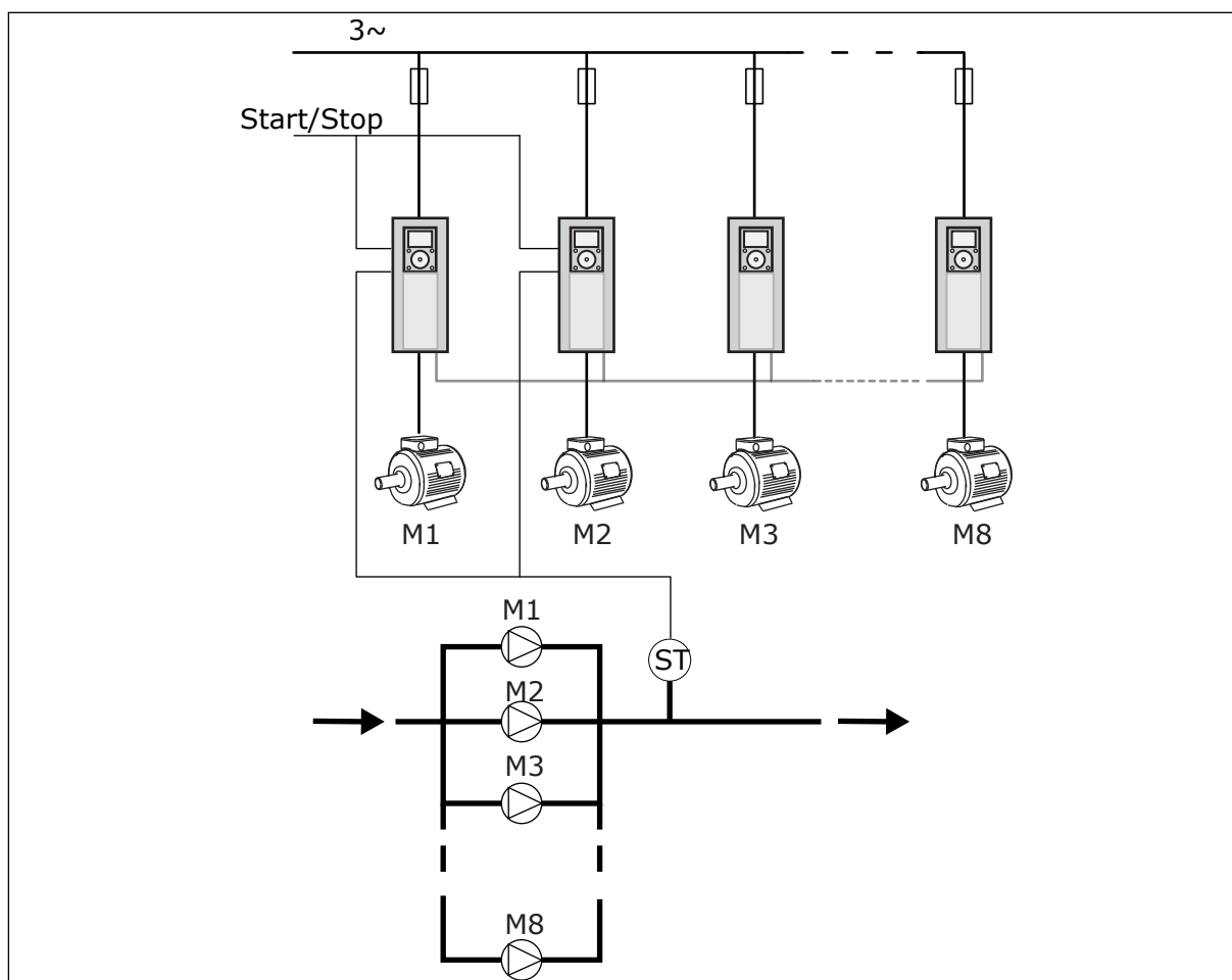
Obr. 90: Konfigurace s vlastními měniči (PT = snímač tlaku)
