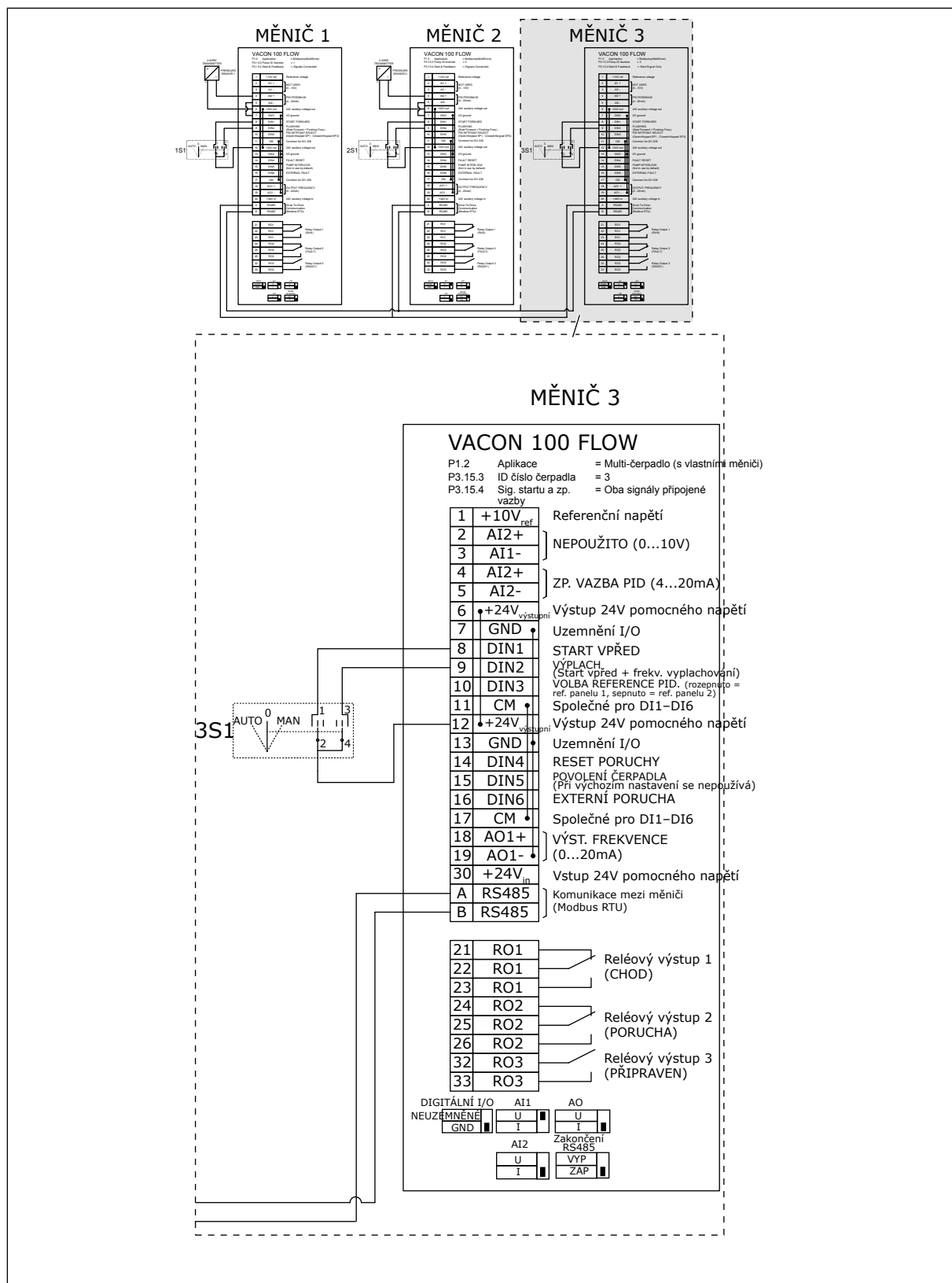
Obr. 26: Schéma elektrického zapojení systému multi-čerpadla (s vlastními měniči), příklad 3C
