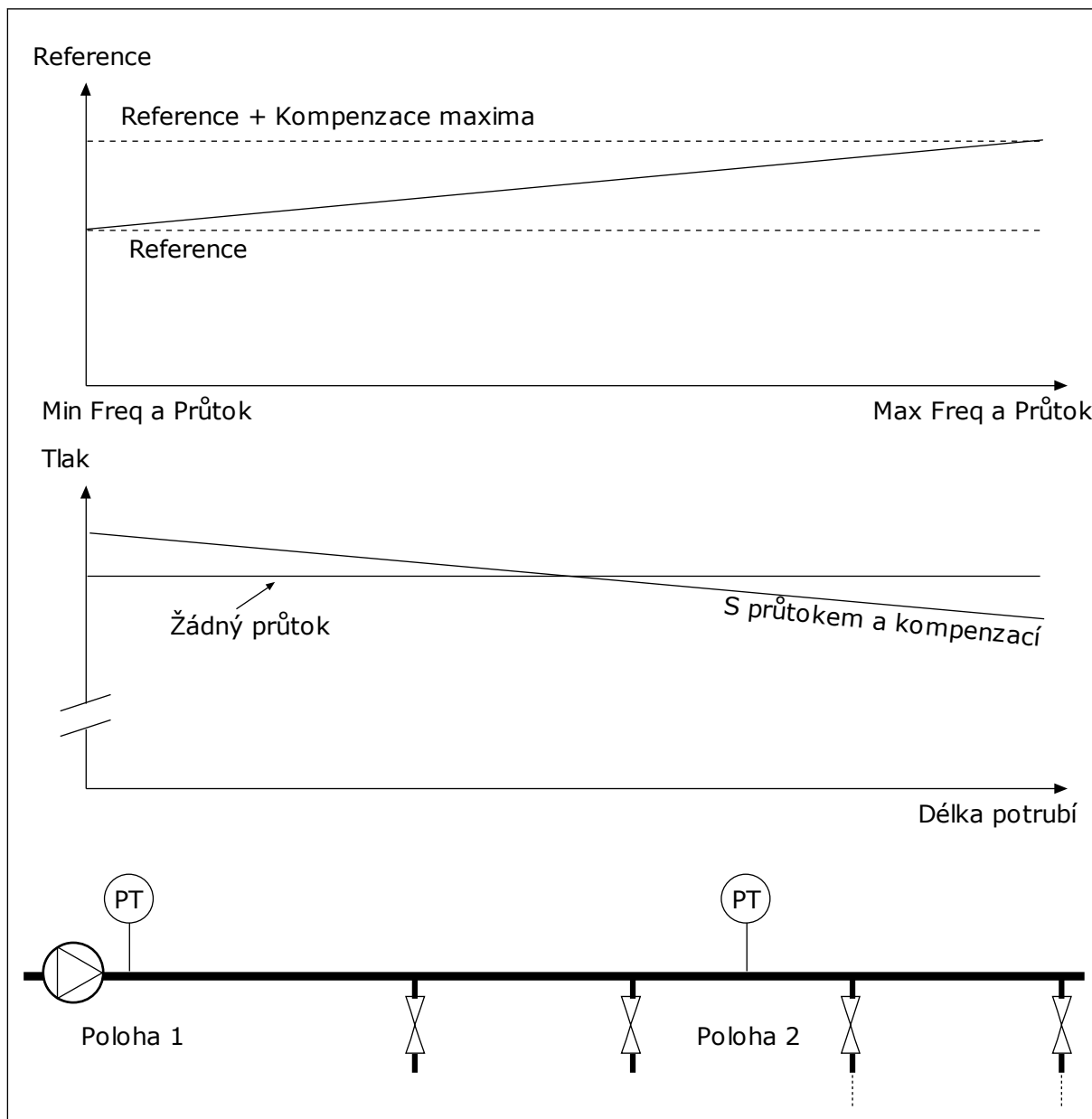
Obr. 85: Zapnutí reference 1 pro kompenzaci poklesu tlaku
