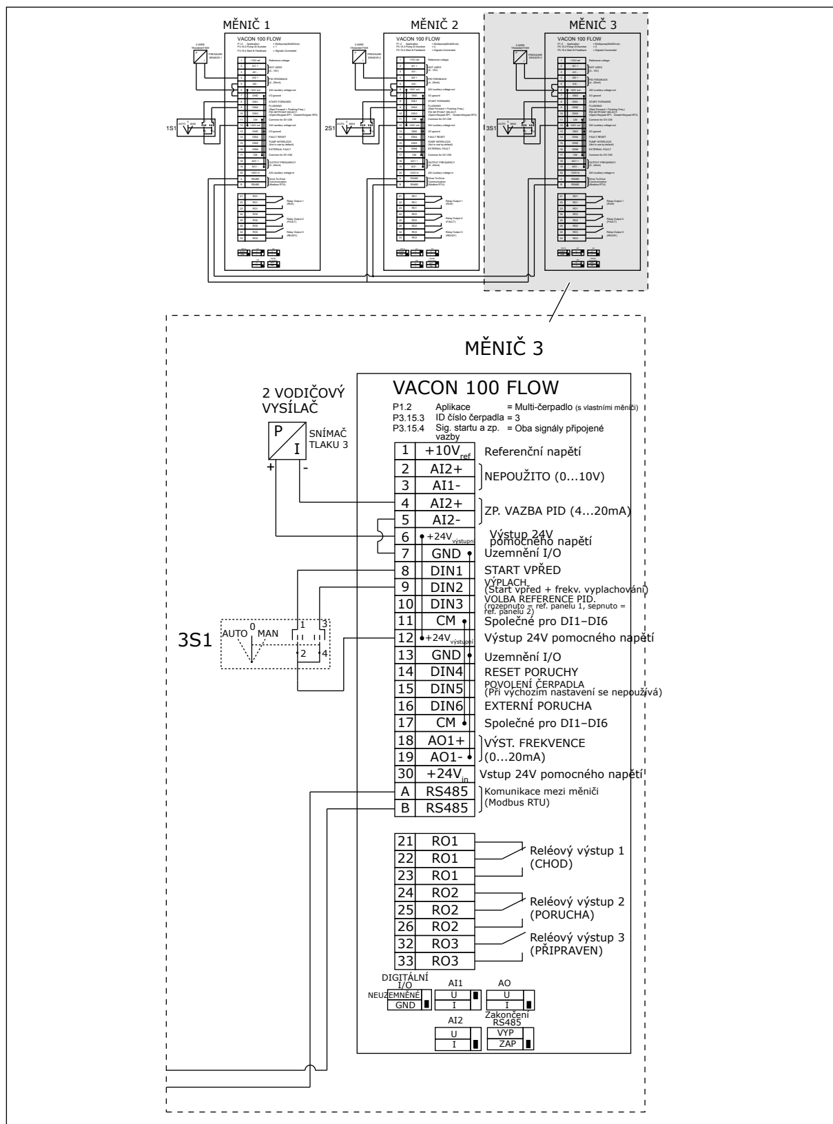
Obr. 20: Schéma elektrického zapojení systému multi-čerpadla (s vlastními měniči), příklad 1C
