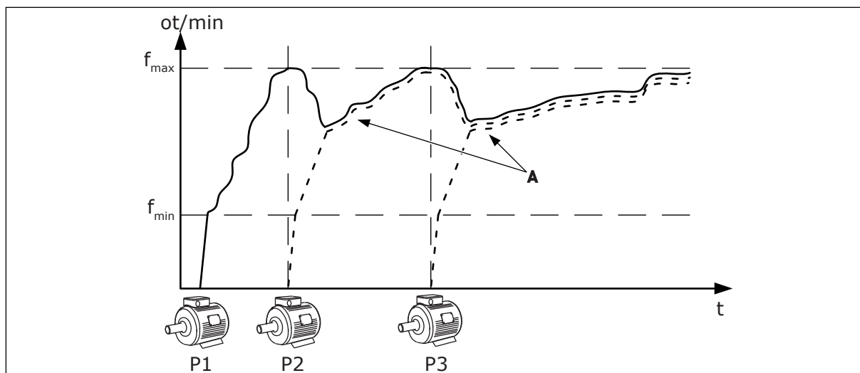
Obr. 92: Řízení v režimu Multifollower
