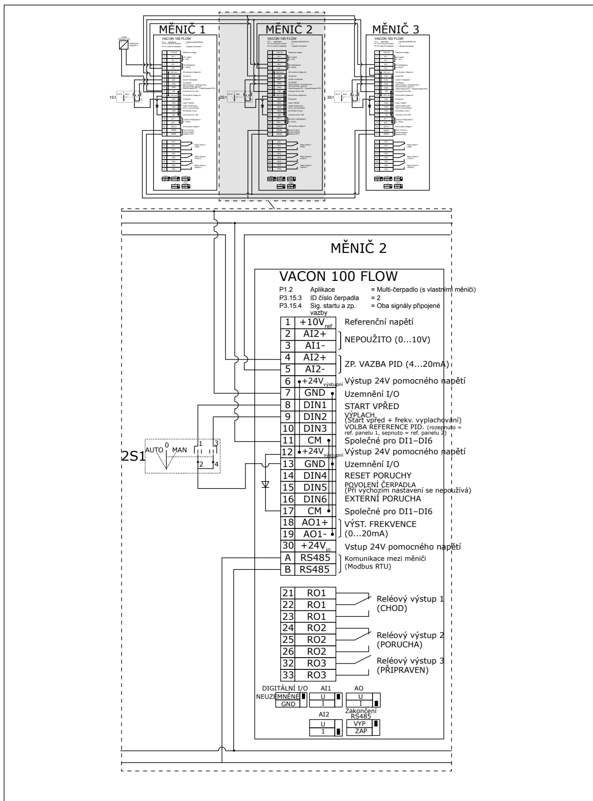
Obr. 22: Schéma elektrického zapojení systému multi-čerpadla (s vlastními měniči), příklad 2B
