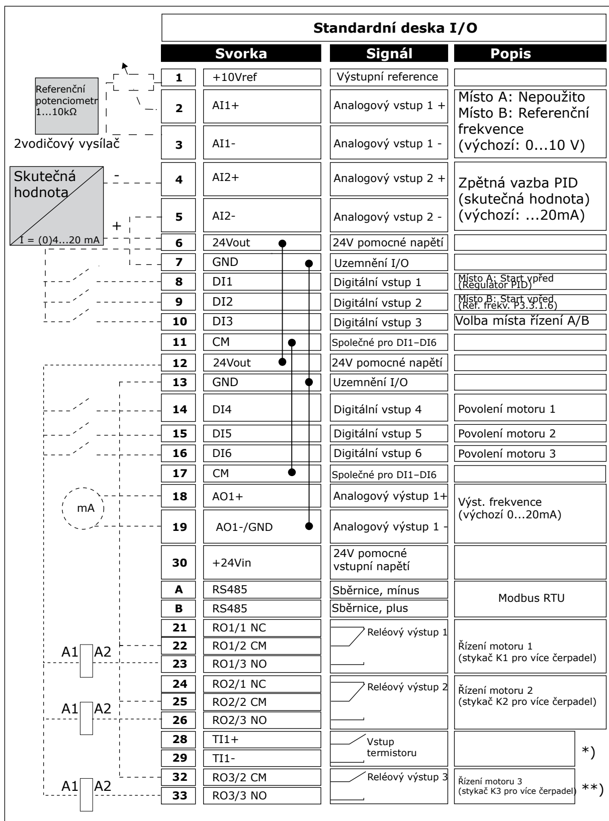
Obr. 11: Výchozí připojení řízení v aplikaci multi-čerpadla (se samostatným měničem)
