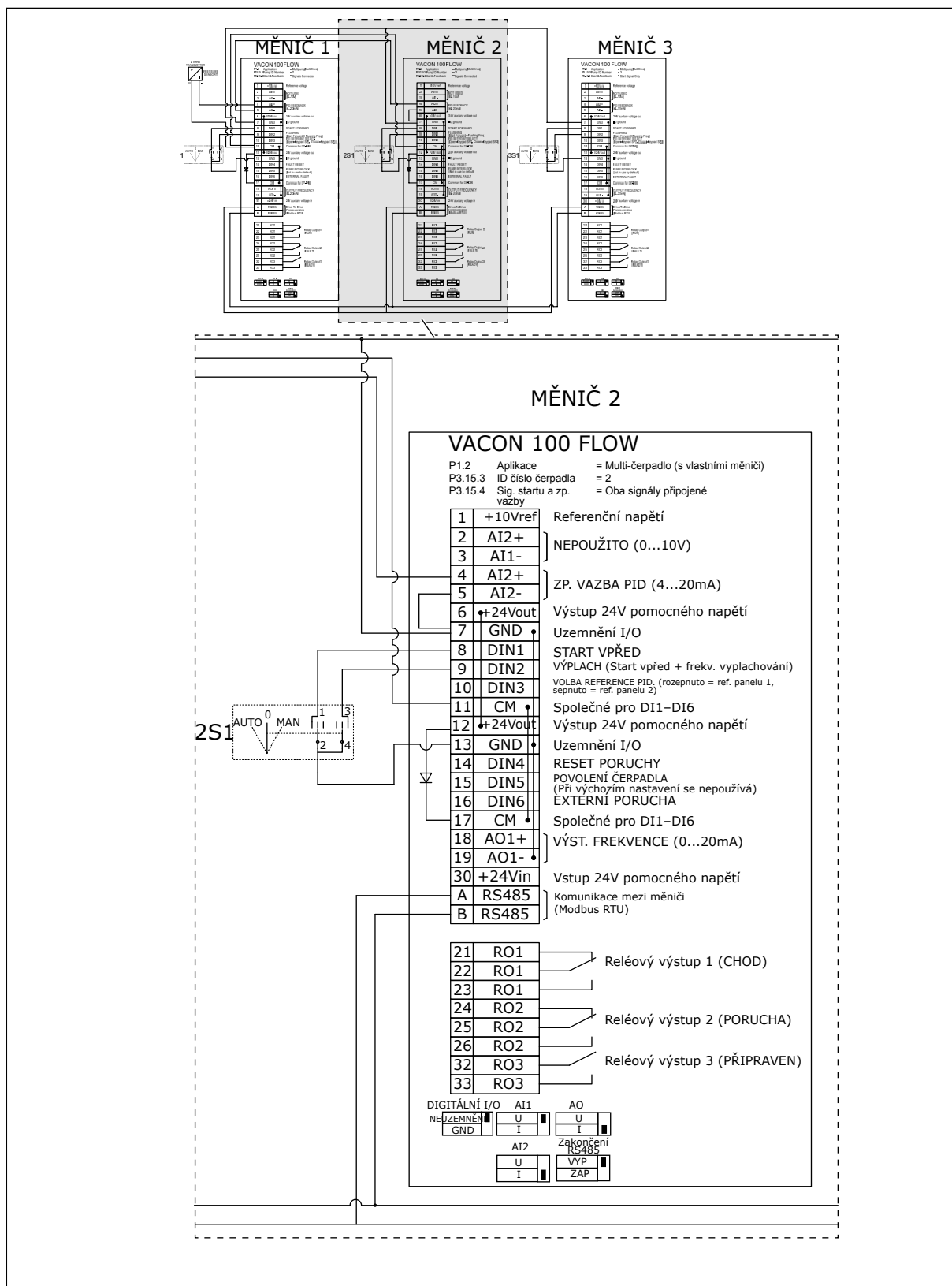
Obr. 28: Schéma elektrického zapojení systému multi-čerpadla (s vlastními měniči), příklad 4B
