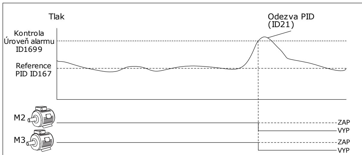
Obr. 100: Funkce kontroly přetlaku
