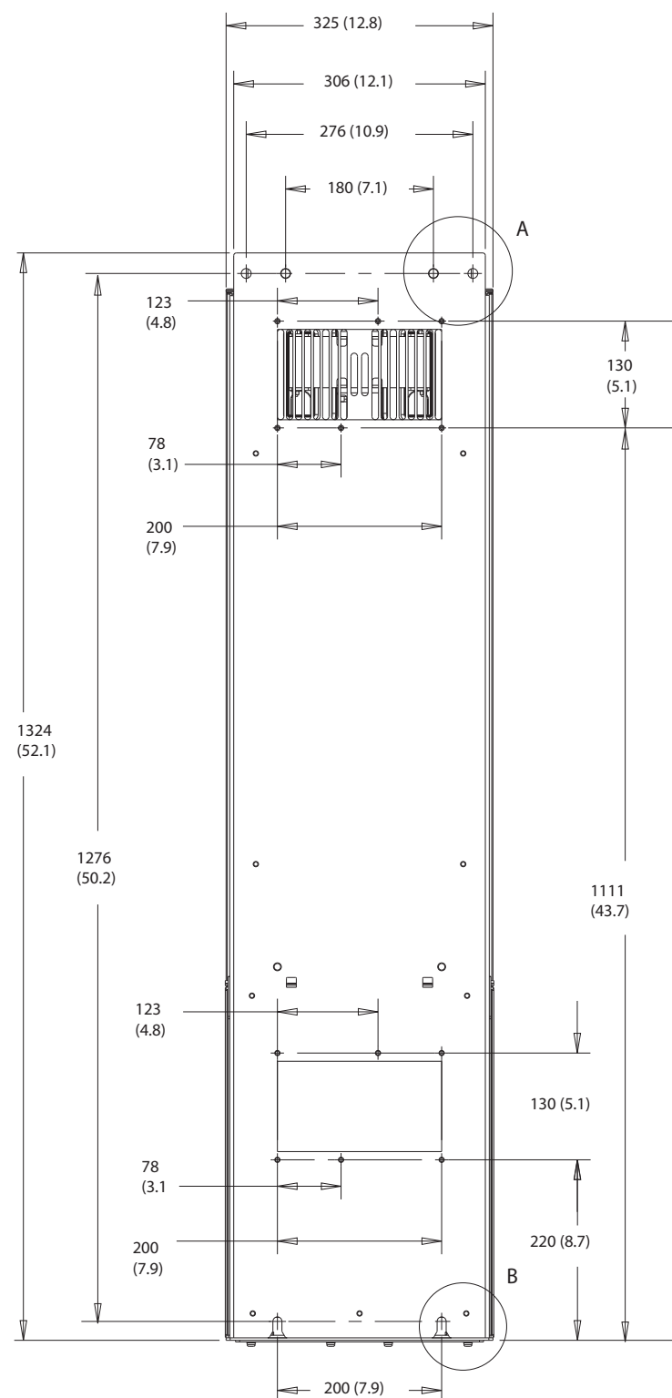
Illustration 10.20 D5h set bagfra
