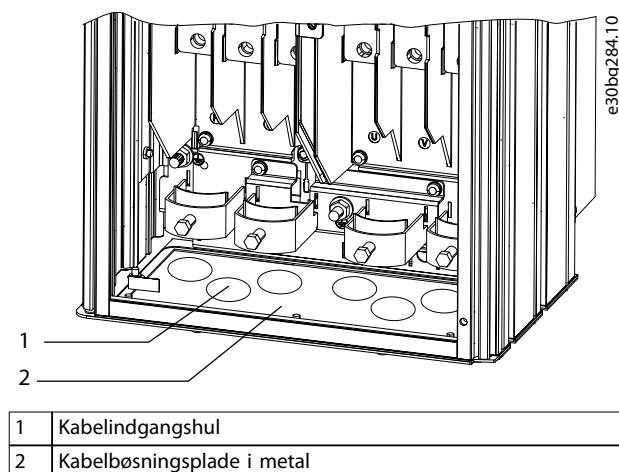
Illustration 4.4 Kabelåbninger i kabelbøsningssplade i metal
