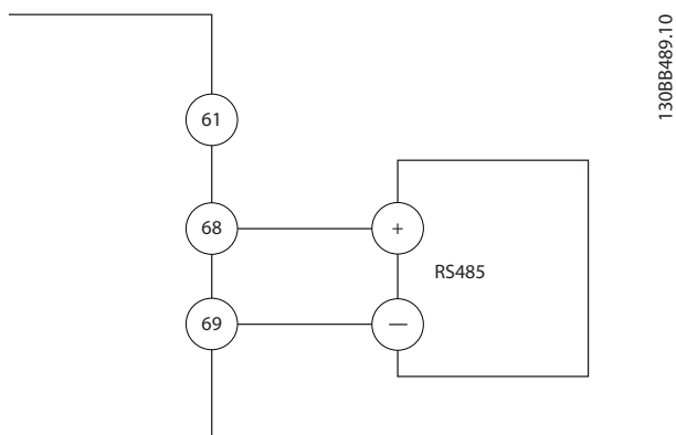
Illustration 5.39 Forbindelsesdiagram for serie kommunikation
