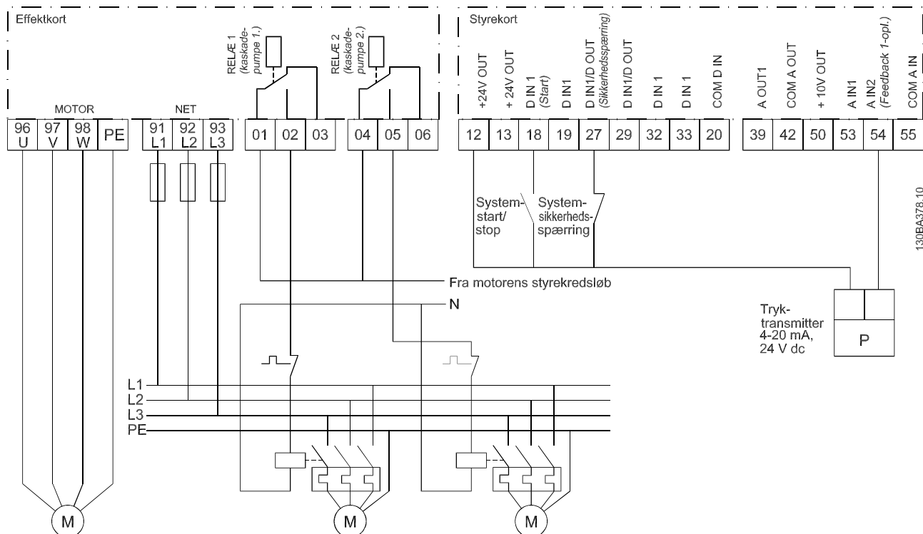
Illustration 8.4 Ledningsdiagram for kaskadestyreenhed
