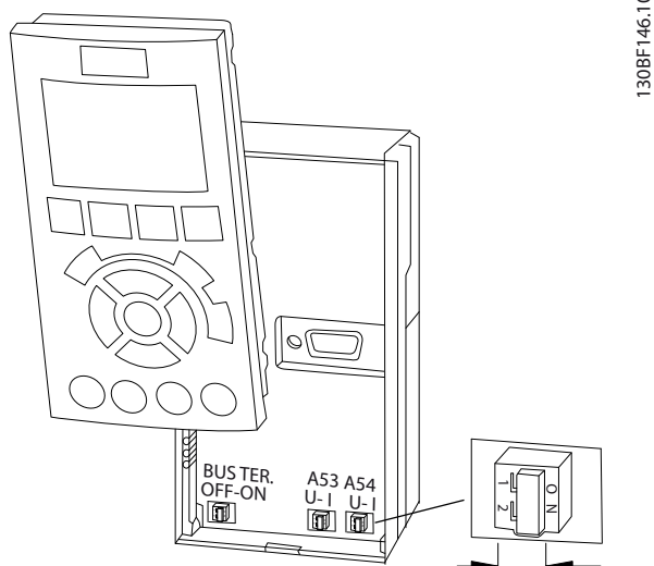
Illustration 5.40 Placering af kontakter til klemme 53 og 54
