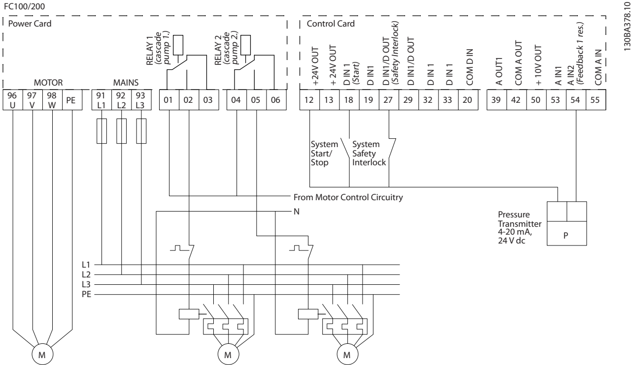
Εικόνα 8.4 Διάγραμμα καλωδίωσης ελεγκτή διαδοχικών βαθμίδων
