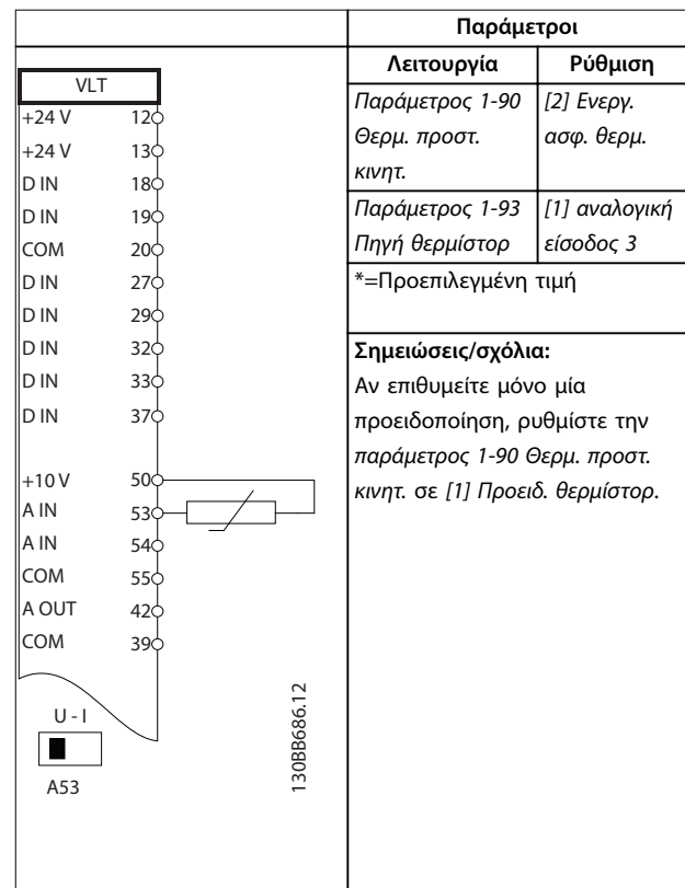
Πίνακας 8.13 Διαμόρφωση καλωδίωσης για θερμίστορ κινητήρα
