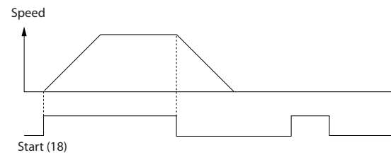
그림 6.2 안전 정지 기능이 있는 기동/정지 명령
