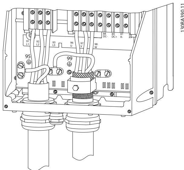
그림 4.8 차폐 케이블을 사용한 외함 유형 B 및 C의 모터, 주전원 및 접지 배선
