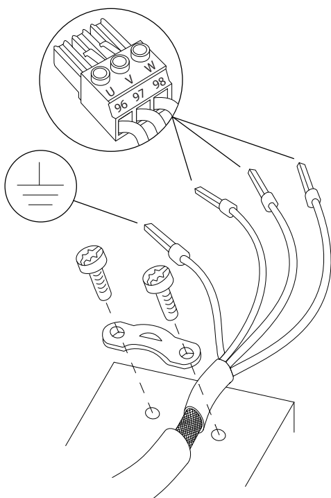
그림 4.5 모터 연결
