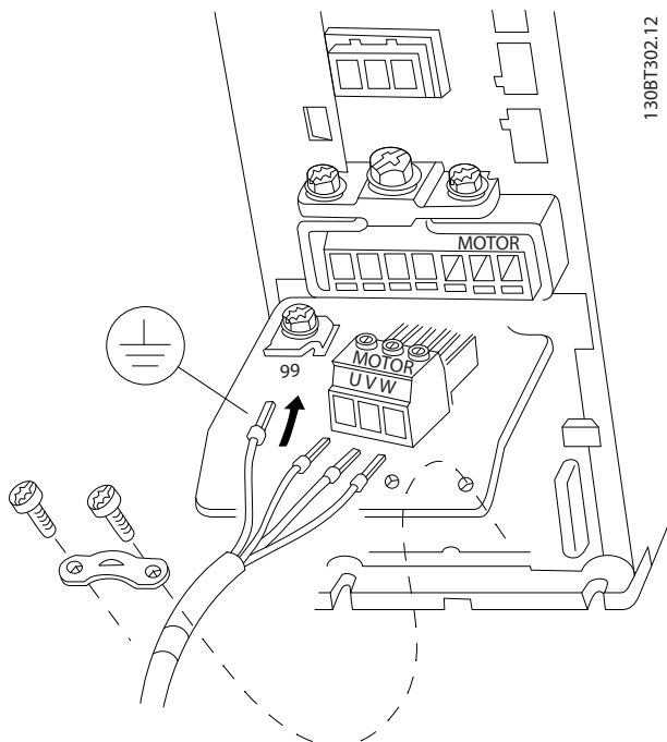
그림 4.6 외함 유형 A2 및 A3의 모터 연결부
