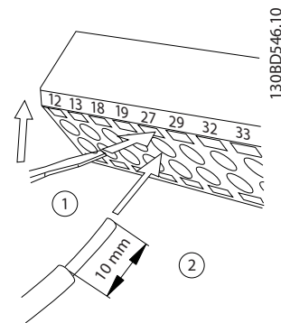
그림 4.12 제어 와이어 연결
