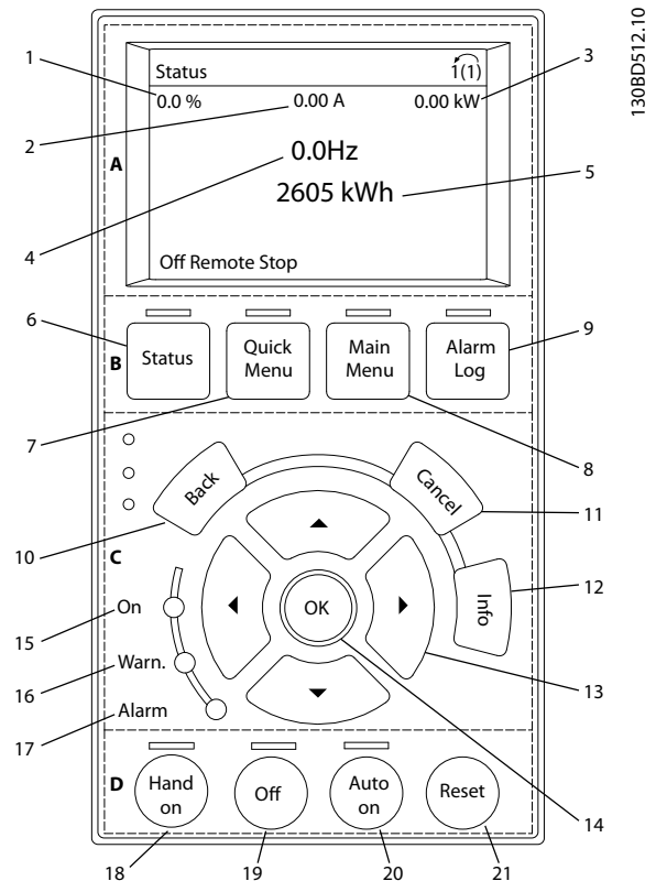
그림 5.1 현장 제어 패널(LCP)
