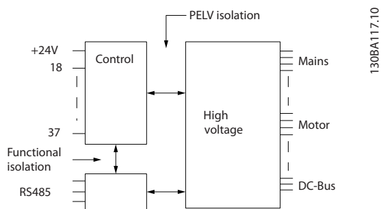
그림 8.1 PELV 절연
