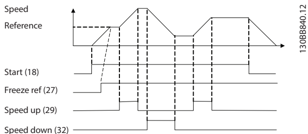
Illustration 8.3 Accélération/décélération
