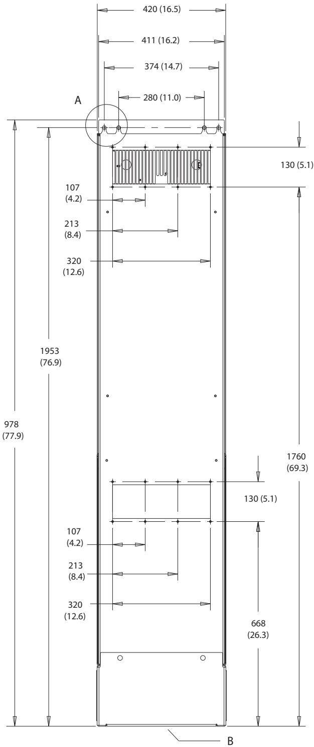
Illustration 10.32 Vue arrière du boîtier D7h
