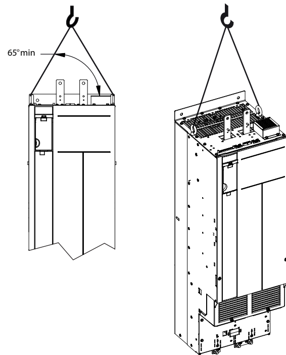
Illustration 4.3 Levage du variateur
