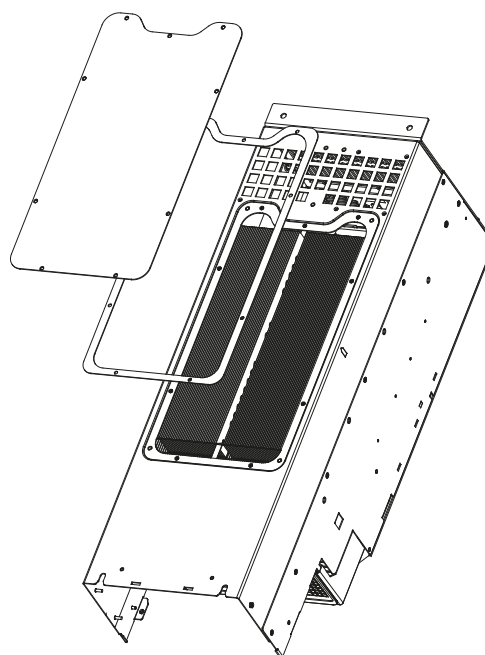
Ábra 9.1 A hűtőborda fedőlapja
