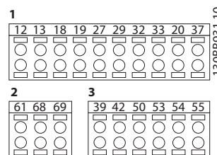
Afbeelding 4.11 Klemnummers
