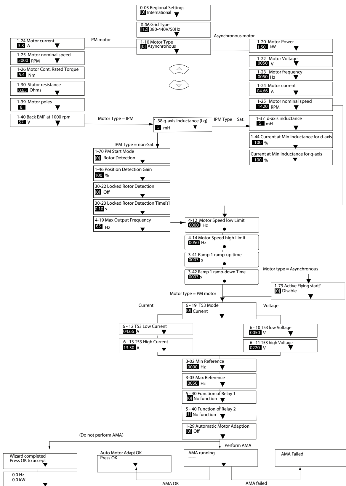
Obrázek 5.7 Konfigurace pro aplikace bez zpětné vazby
