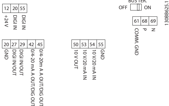
Obrázek 4.11 Řídicí svorky
