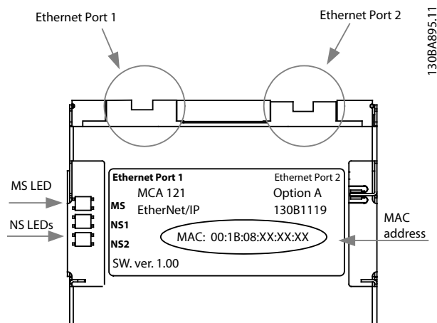
Abbildung 4.1 Übersicht der EtherNet/IP-Schnittstelle
