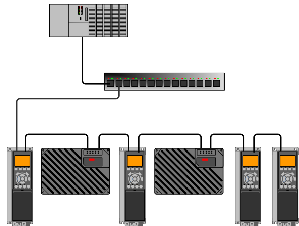
Abbildung 3.3 Reihentopologie
