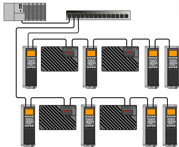
Abbildung 3.5 Empfohlene Projektierungsregeln
