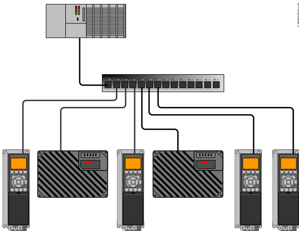
Abbildung 3.2 Sterntopologie
