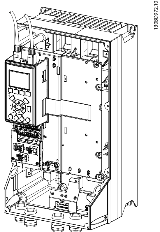
Abbildung 3.11 Verkabelung für Gehäusetypen A4-A5, B1-B4 und C1-C4
