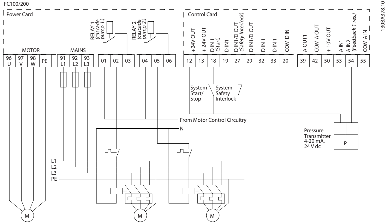
그림 8.4 캐스케이드 컨트롤러 배선 다이어그램
