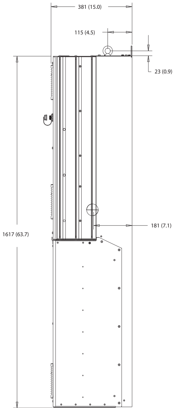
그림 10.25 D6h의 측면 보기
