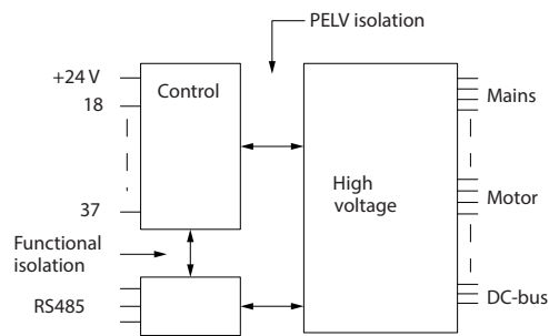
그림 10.1 PELV 절연
