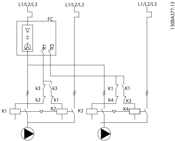
그림 8.6 리드 펌프 절체 배선 다이어그램
