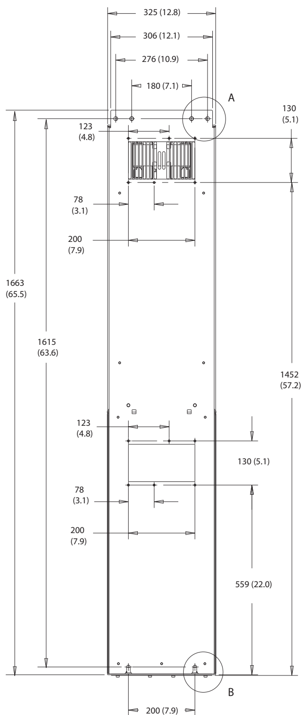
그림 10.26 D6h의 뒷면 보기
