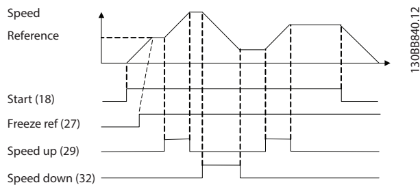
그림 8.3 가속/감속
