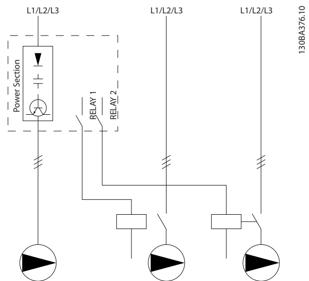
그림 8.5 고정 가변 속도 펌프 배선 다이어그램
