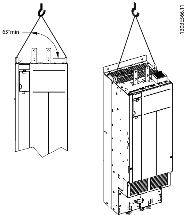
그림 4.3 드라이브 들어 올리기
