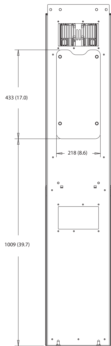
그림 10.27 D6h의 방열판 액세스 치수
