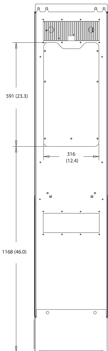
그림 10.33 D7h의 방열판 액세스 치수
