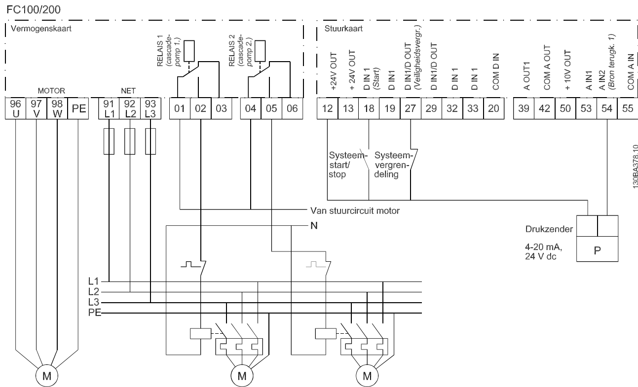
Afbeelding 8.4 Bedradingsschema cascaderelgaar
