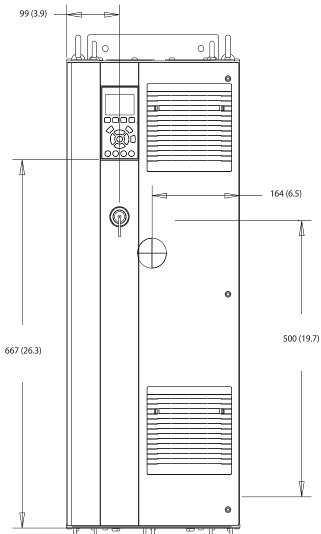
Afbeelding 10.2 Vooraanzicht D1h
