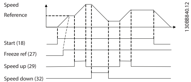
Afbeelding 8.3 Snelheid omhoog/omlaag
