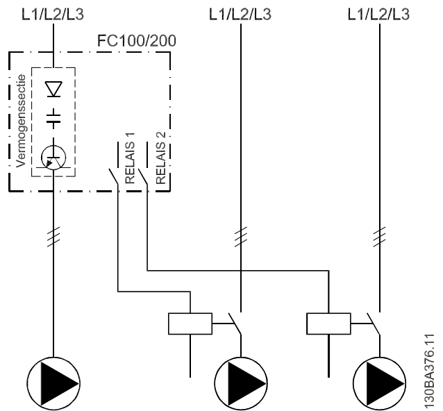
Afbeelding 8.5 Bedradingschema voor pomp met variabel toerental
