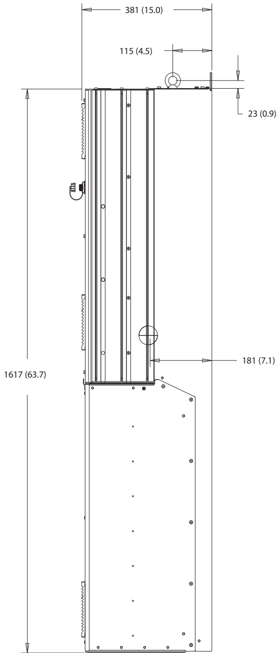
Afbeelding 10.25 Zijaanzicht D6h
