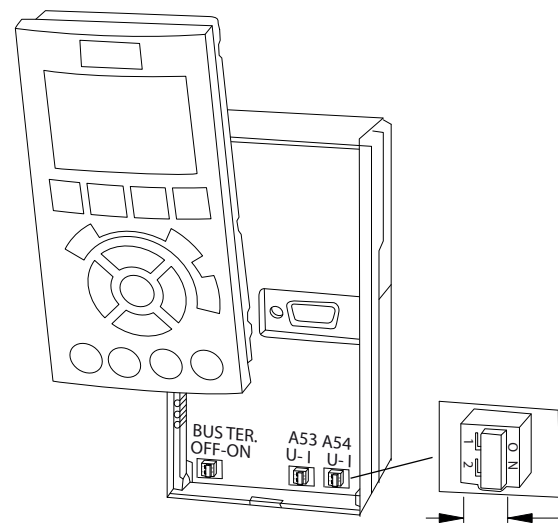
Afbeelding 5.40 Positie van de schakelaars voor klem 53 en 54
