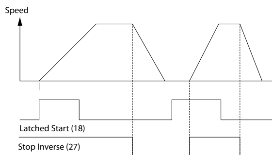
Afbeelding 8.2 Pulsstart/Stop geïnverteerd
