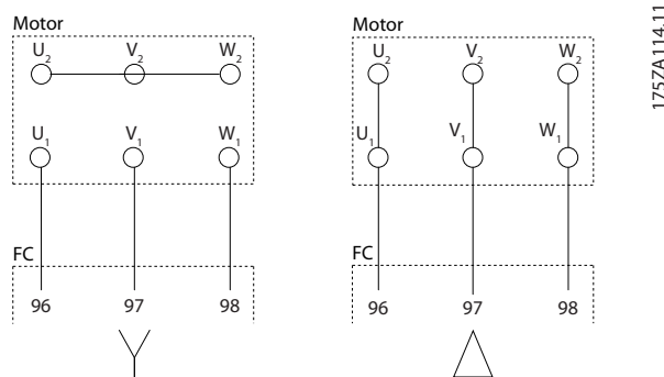
图 10.5 电动机电缆连接
