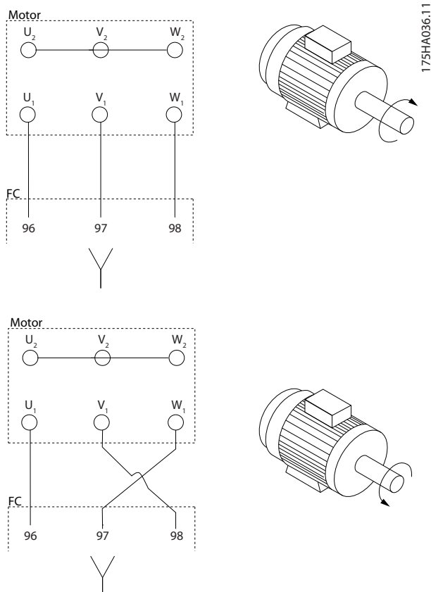
图 10.19 更改电动机旋转情况
