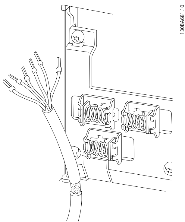
图 10.16 控制电缆的屏蔽丝网端接和应力消除装置
