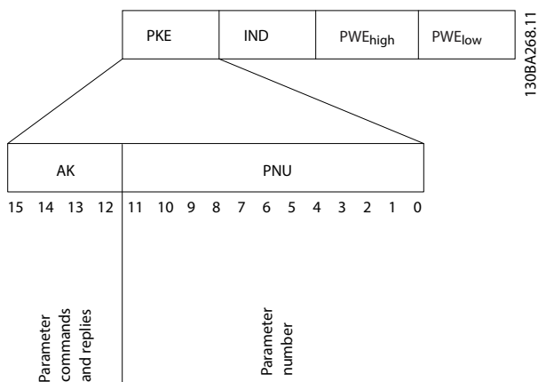
图 14.10 PKE 字段
