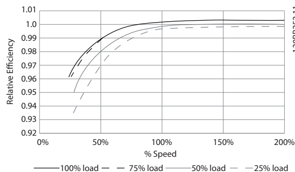
图 10.26 典型效率曲线
