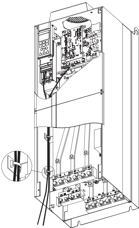
图 10.8 E1 和 E2 机箱的控制卡接线路径
