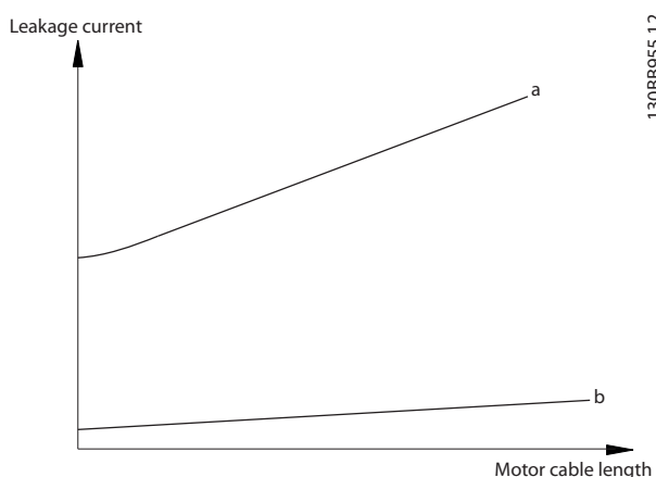
图 10.22 电机电缆长度和功率规格会影响漏电电流。功率规格 a > 功率规格 b。
