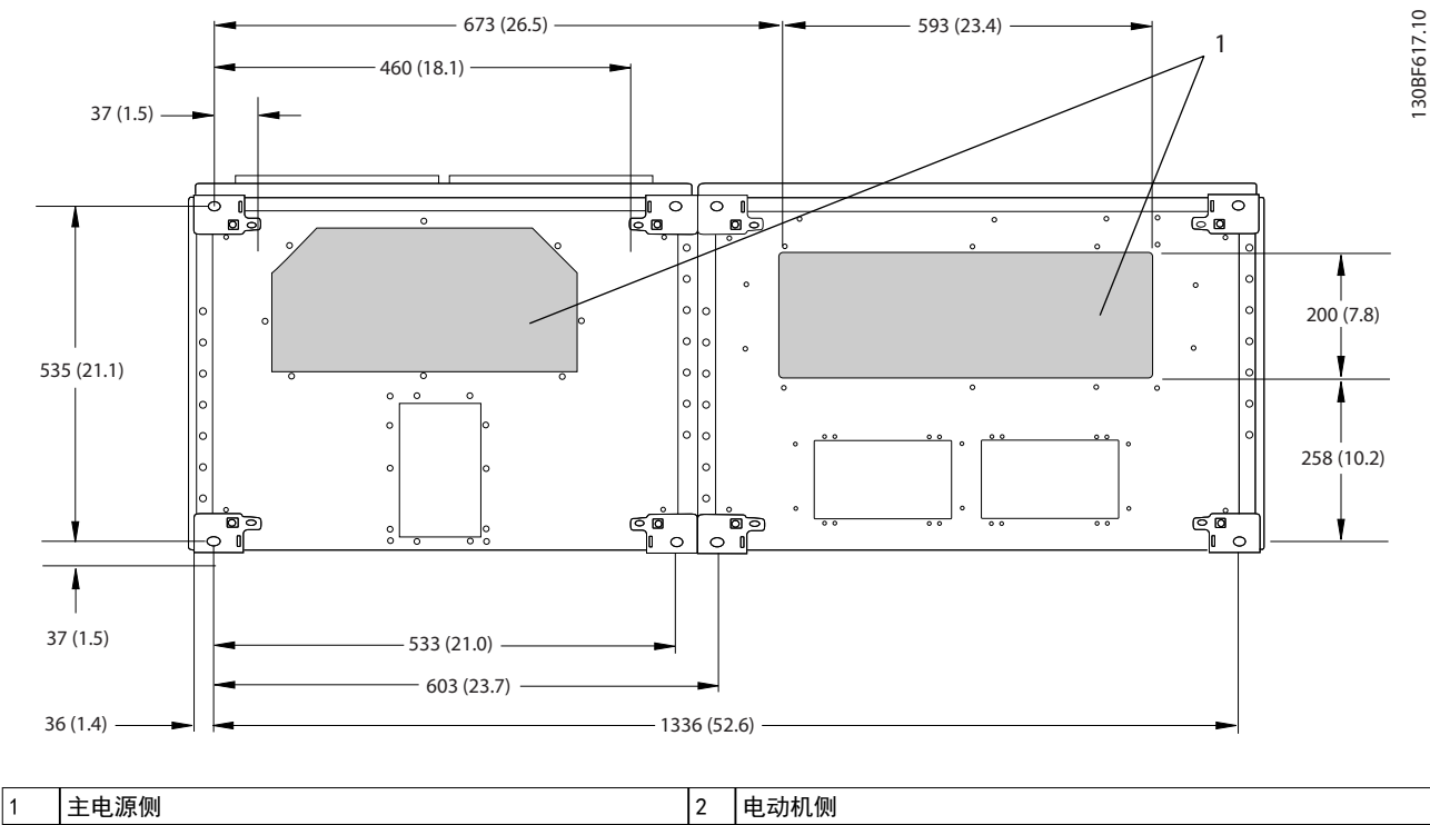
图 8.61 F9 的密封板尺寸
