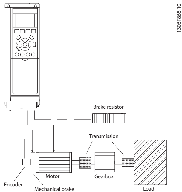
图 12.1 FC 302 闭环速度控制的基本设置
