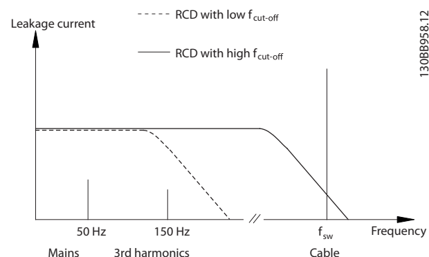
图 10.24 漏电电流的主要成分
