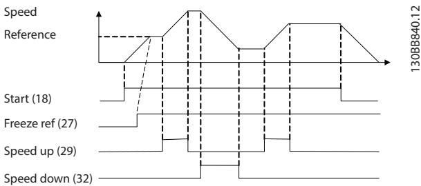
图 12.4 加速/减速
