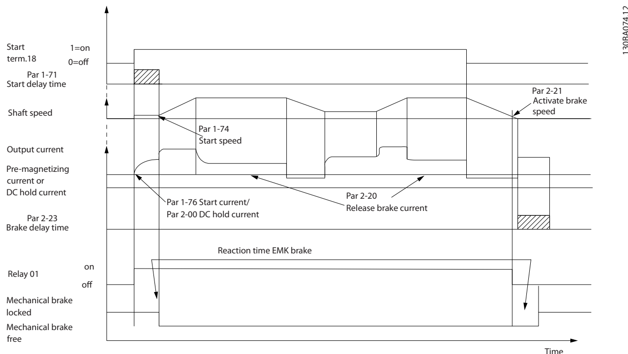
图 5.7 开环中的机械制动控制
