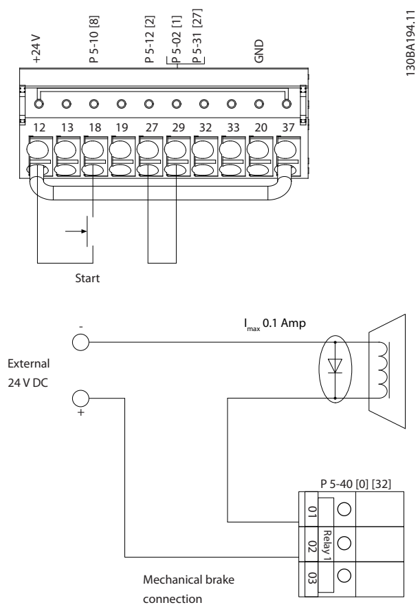
图 12.8 用于转矩和停止极限的接线配置
