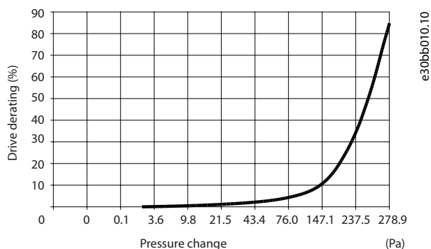
图 9.5 以下机箱随压力变化发生的降容：E1 - E2 机箱 380 - 500 V 型号：P250 和 525 - 690 V 型号：P355 - P400。气流：650 cfm (1105 m³/h)
