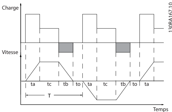
图 10.21 典型的制动周期
