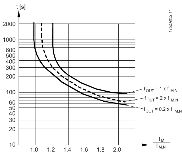
图 5.1 ETR 特性
