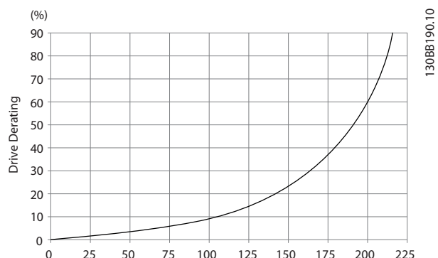
图 9.7 以下机箱随压力变化发生的降容：F1 - F4 机箱。气流：580 cfm (985 m³/h)
