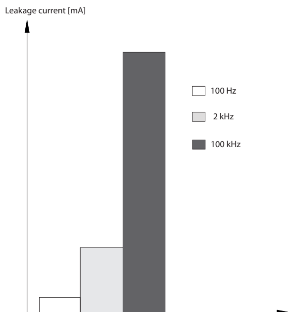
图 10.25 RCD 截止频率对漏电电流的影响
