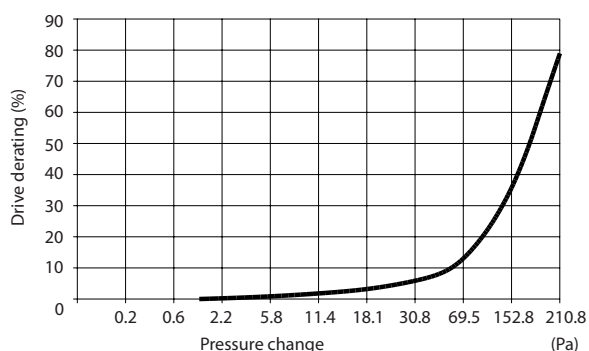
图 9.6 以下机箱随压力变化发生的降容：E1 - E2 机箱 380 - 500 V 型号：P315 - P400 和 525 - 690 V 型号：P500 - P560。气流：850 cfm (1445 m³/h)
