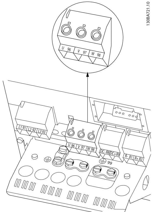
图 8.15 机箱 B4 的电动机接线
