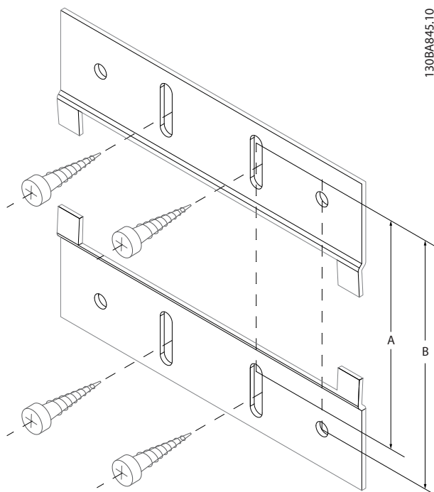
图 3.40 上托架
