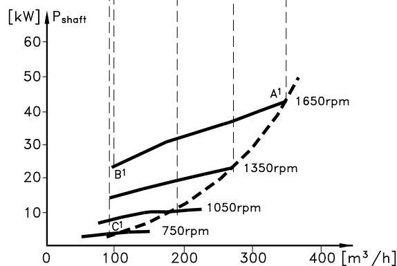
图 2.4 不同速度的能耗
