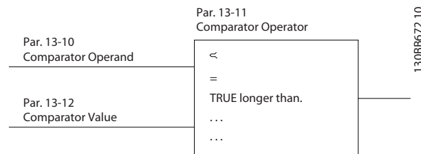
图 2.18 比较器
