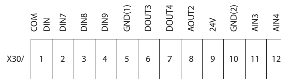
图 7.4 MCB 101 选项
