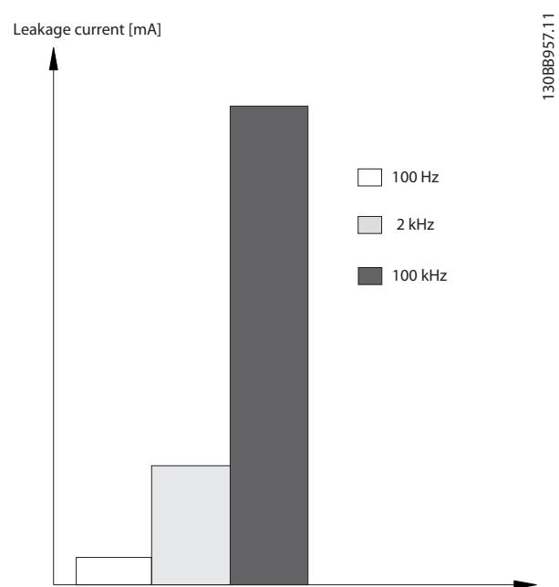
图 3.9 RCD 截止频率对漏电电流的影响
