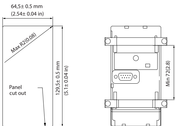
图 3.38 LCP 套件尺寸
