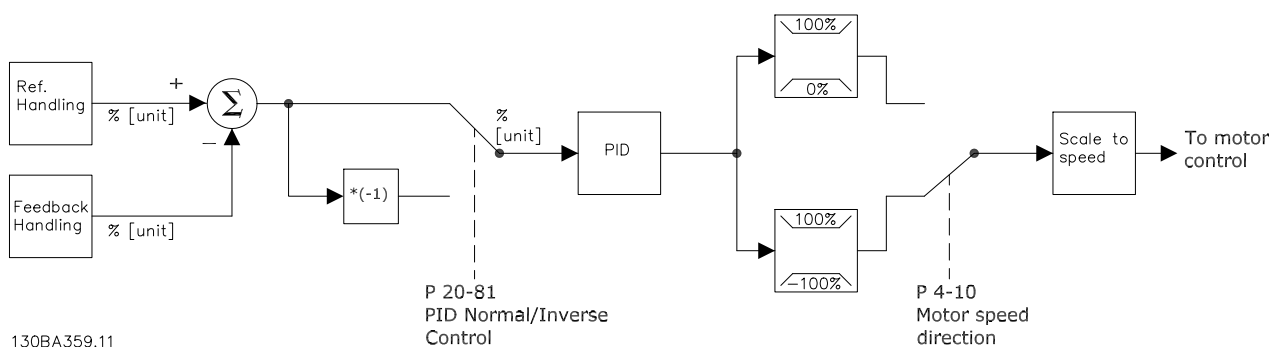
图 2.9 闭环控制器框图
