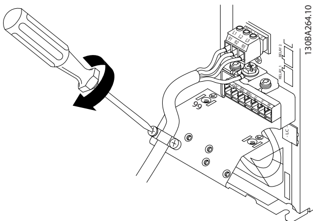
图 8.1 支撑托架
