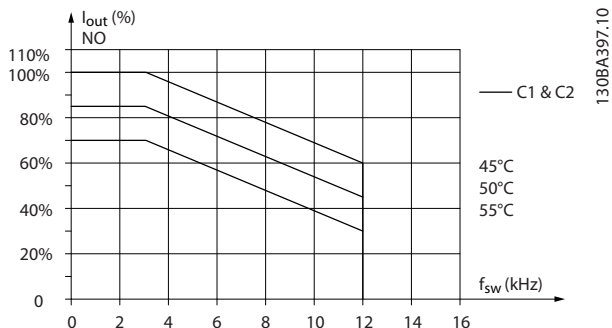
图 5.14 I out 在不同 T AMB, MAX 下的降容, 机箱规格 C1 和 C2., 正常过载模式 (110% 过转矩)
