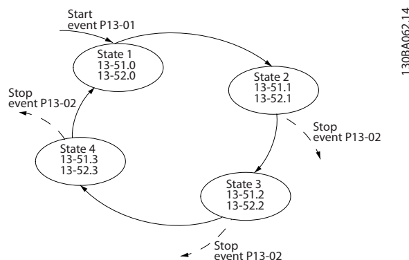
图 2.17 对 4 个事件/操作编程时的执行顺序
