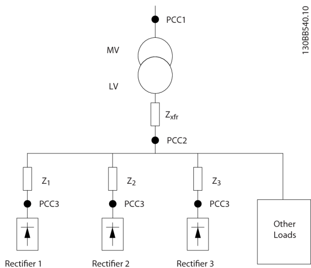
图 3.4 小配电系统
