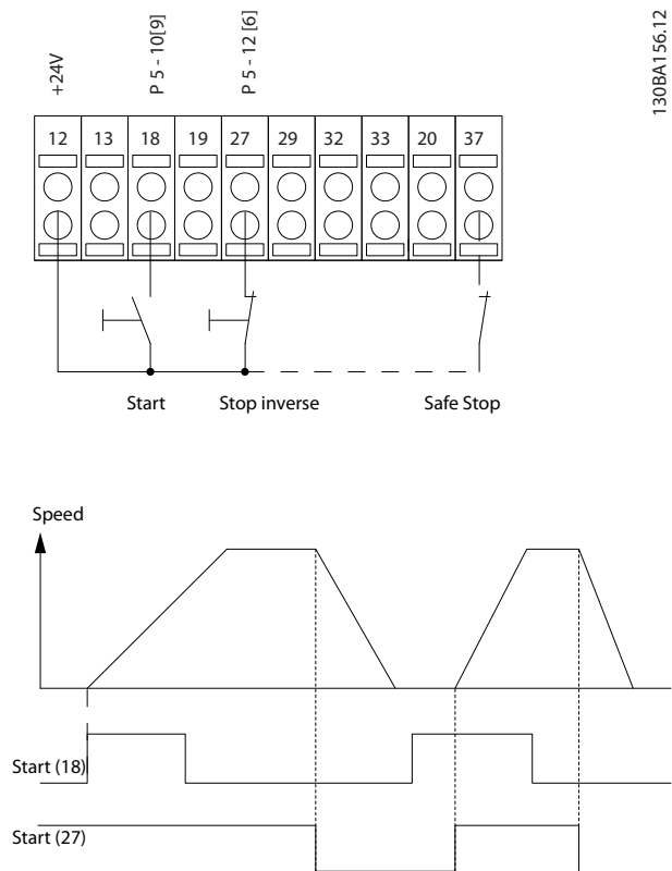
图 4.2 端子 37: 仅随 ST0 一起提供
