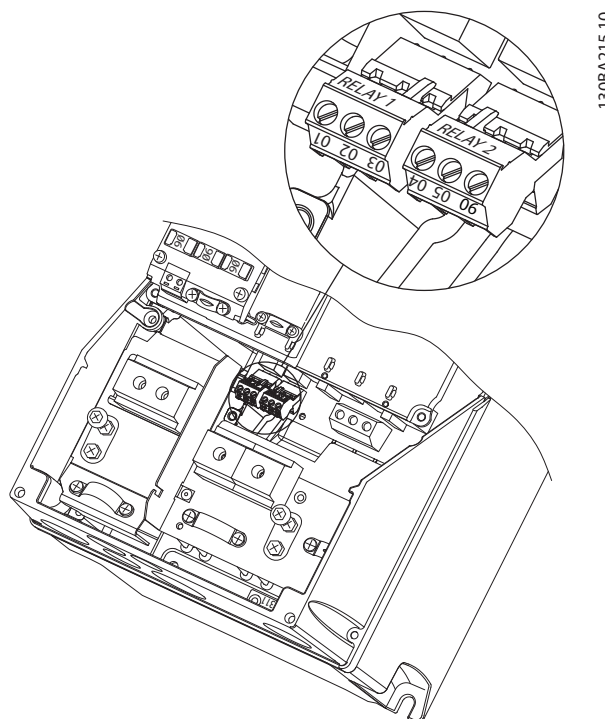
图 8.20 继电器连接端子 (机箱规格 A5、B1 和 B2)。
