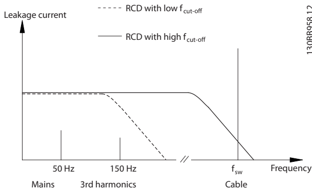
图 3.8 漏电电流的主要成分
