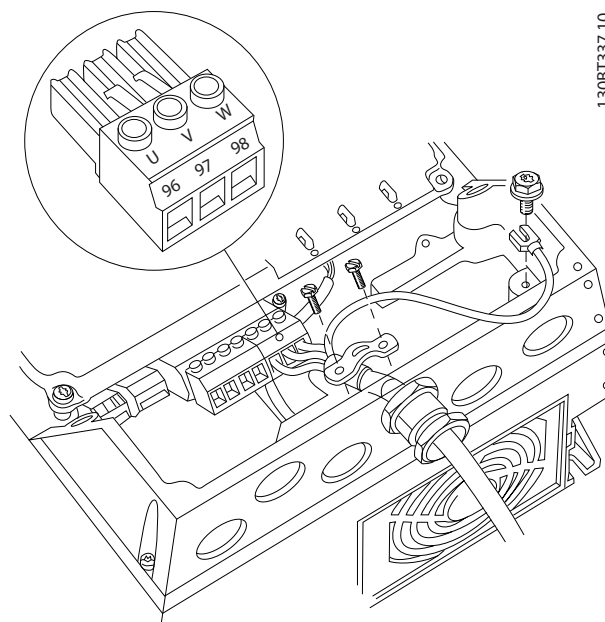
图 8.12 机箱类型 A4/A5 的电动机接线
