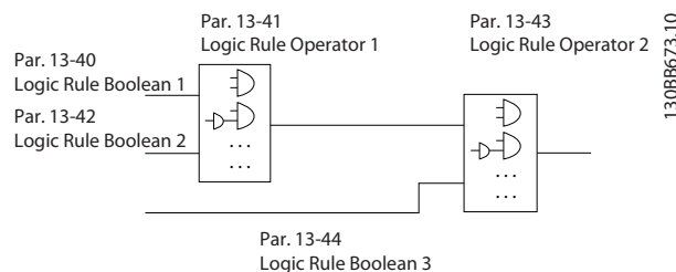
图 2.19 逻辑规则
