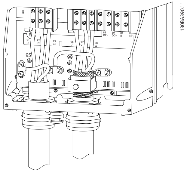
图 8.16 机箱类型 C1 和 C2 (IP 21/NEMA 类型 1 和 IP55/66/NEMA 类型 12) 的主电源接线
