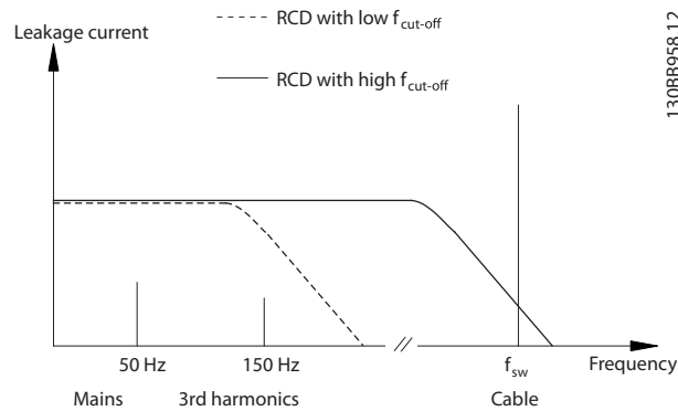
Kuva 2.23 Vuotovirran päätekijät
