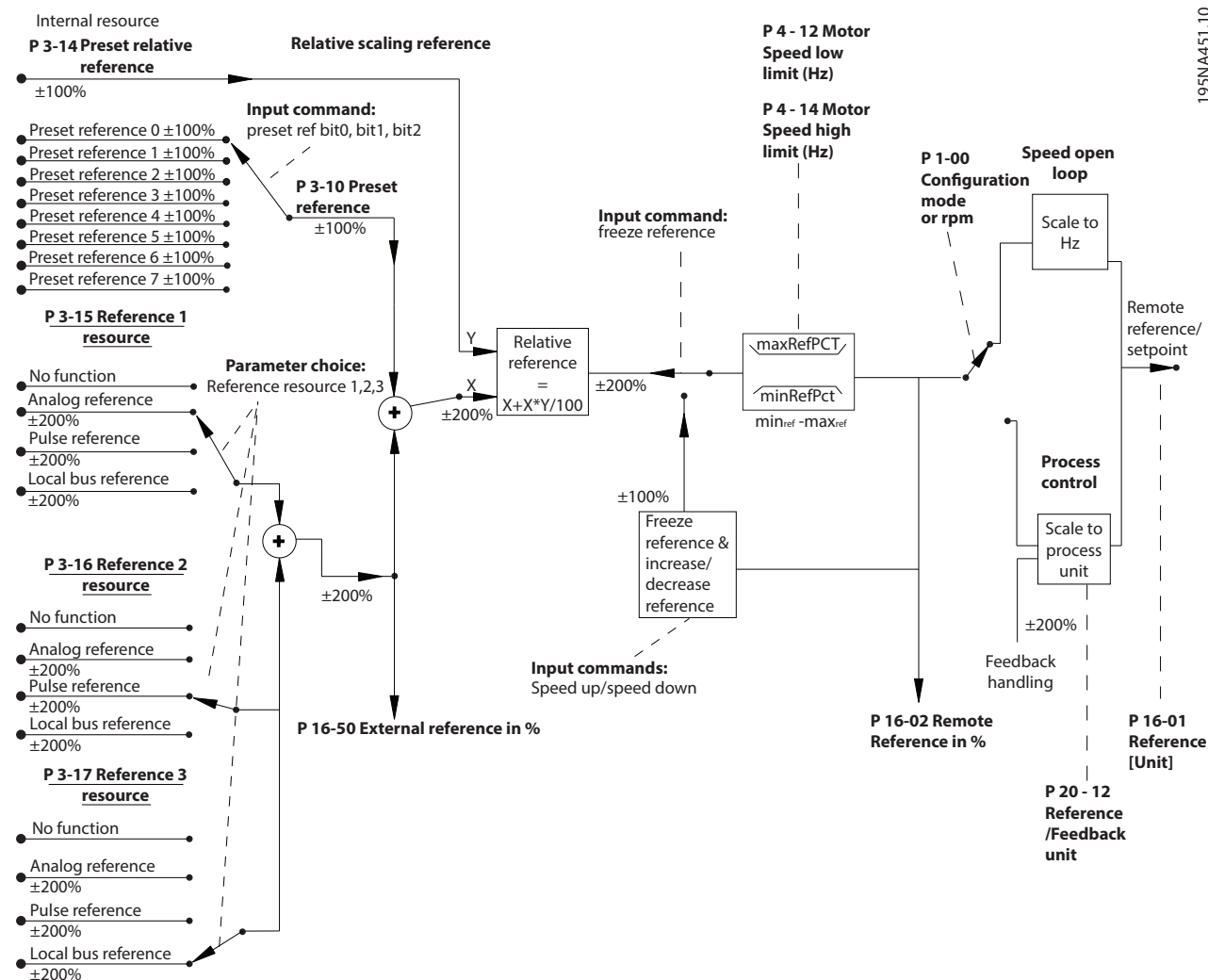
Kuva 2.16 Lohkokaavio, jossa näkyy etäohjearvo
