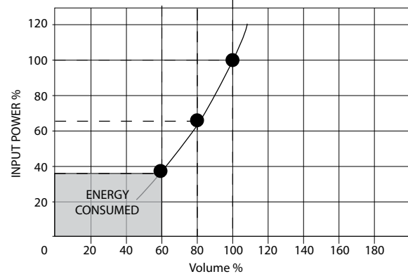
Kuva 4.6 Energiansäästö rajoitetulla puhaltimen kapasiteetilla
