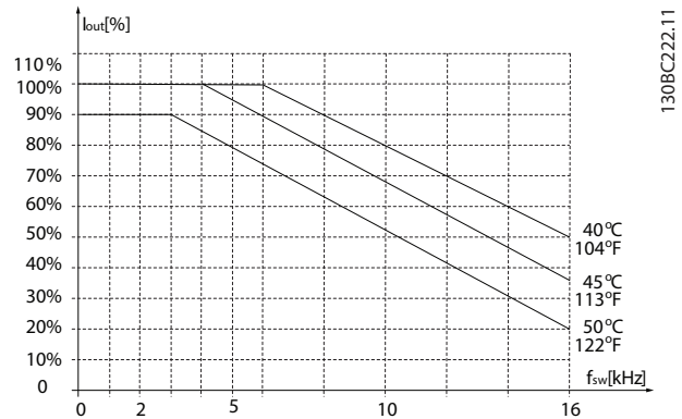
Kuva 6.5 400 V MH3 5.5–7.5 kW (7.5–10 hp)
