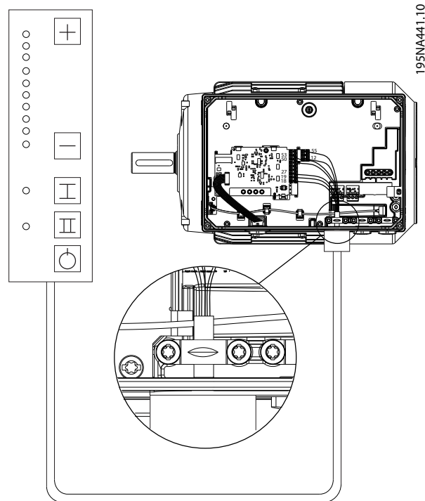
Kuva 3.11 LOP:n kytkennät
