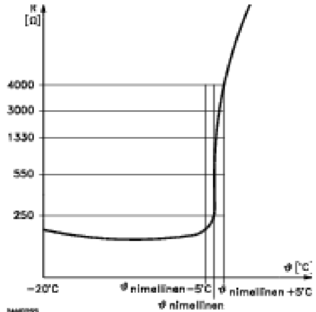
Kuva 3.6 Tyypillinen termistori toiminta
