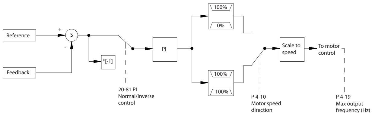
Kuva 2.14 Suljetun piirin ohjain
