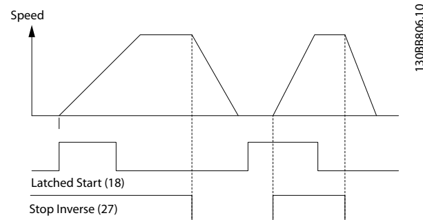
Ilustrația 8.2 Start/oprire inversată prin comandă tip puls
