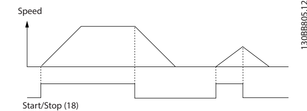
Ilustrația 8.1 Pornirea/oprirea cu funcția Safe Torque Off
