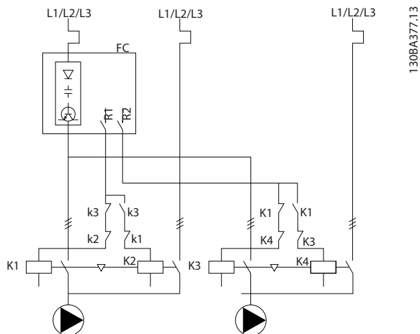
Ilustrația 8.6 Diagrama conductorilor de conectare pentru alternarea pompei principale
