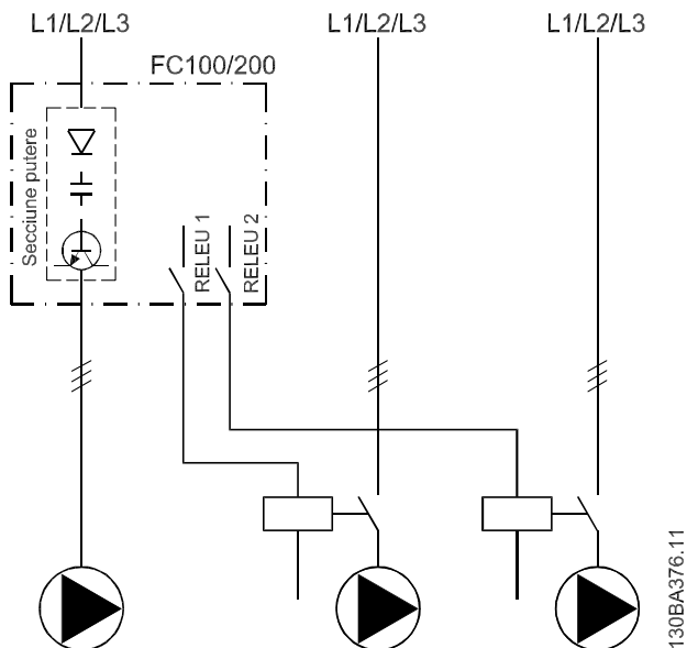
Ilustrația 8.5 Diagrama conductorilor de conectare pentru pompa cu viteză fixă/variabilă
