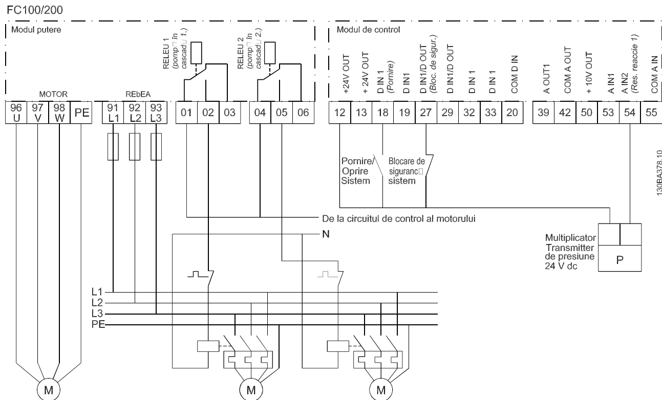
Ilustrația 8.4 Diagrama conductorilor de conectare pentru modulul de control în cascadă
