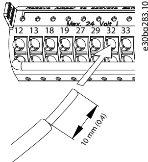
Ilustrația 5.37 Conectarea conductorilor de control solizi
