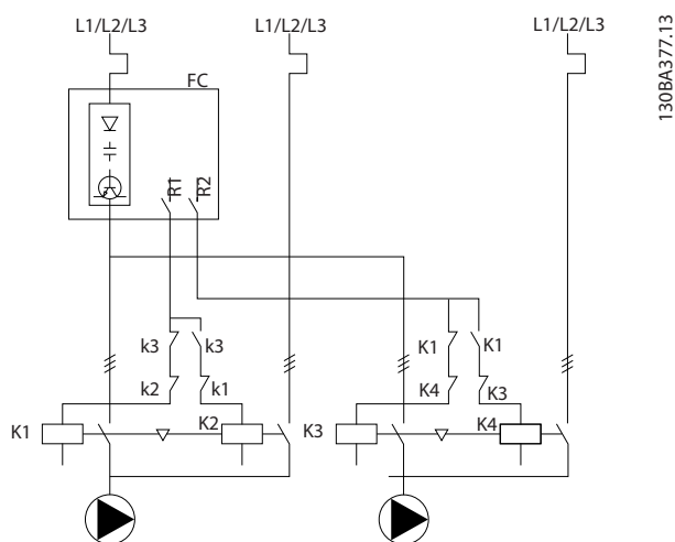
Obrázok 8.6 Schéma zapojenia pre striedanie hlavného čerpadla
