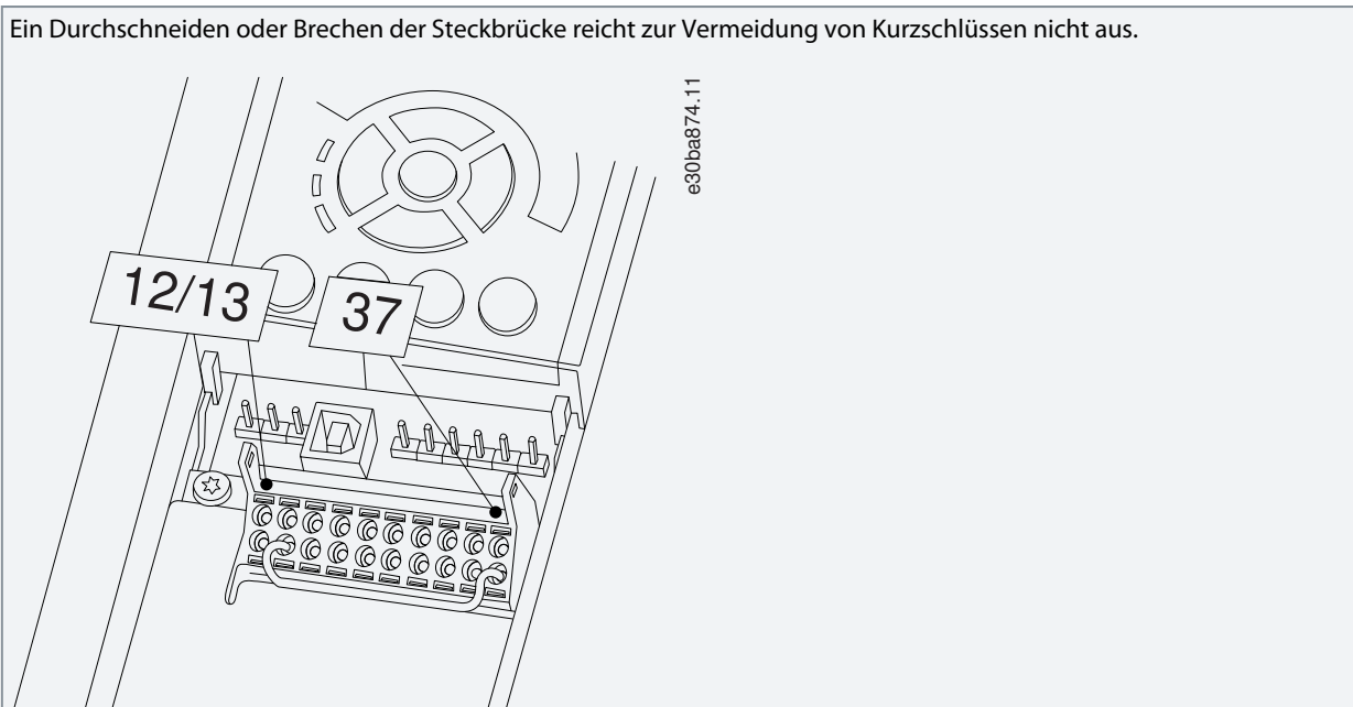
Abbildung 9: Steckbrücke zwischen den Klemmen 12/13 und 37 (VLT® AutomationDrive FC 302)
