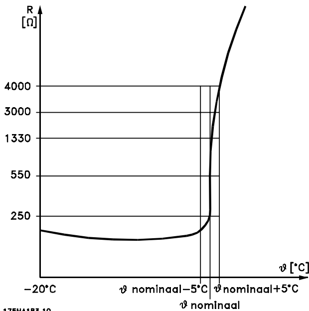
175HA183.10 Afbeelding 3.6 Typisch thermistorgedrag
