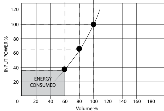
Afbeelding 4.6 Energiebesparing bij gereduceerd ventilatorvermogen
