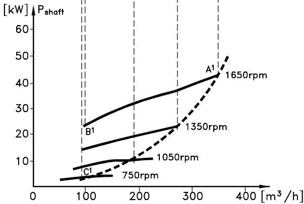
Afbeelding 4.10 Pompprestaties
