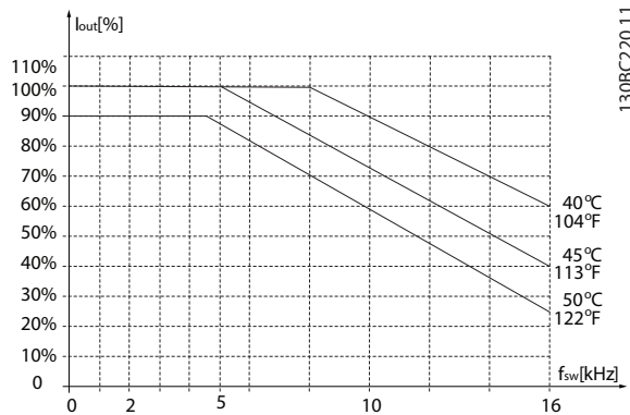
Afbeelding 6.4 400 V MH2 2.2–4.0 kW (3.0–5.0 hp)
