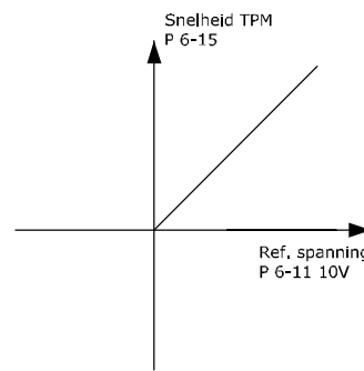
Afbeelding 4.4 Potentiometerreferentie
