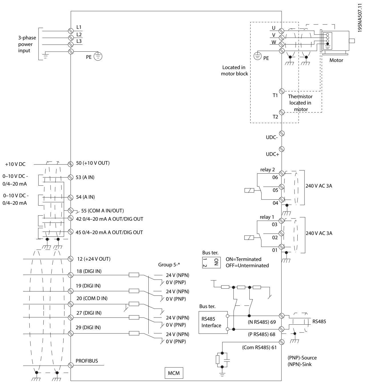
Afbeelding 2.4 Elektrisch overzicht
