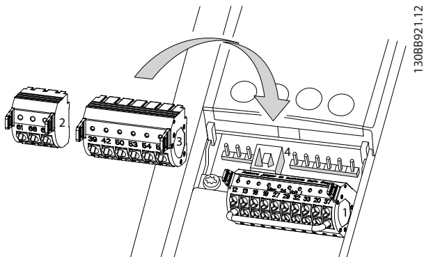
Ілюстрація 4.8 Розташування клем керування
