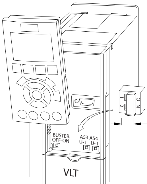
Ілюстрація 4.11 Розташування перемикачів клем 53 та 54
