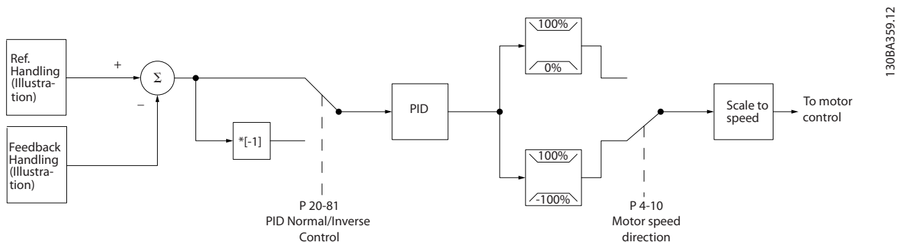
Рисунок 11.7 Блок-схема регулятора с замкнутым контуром
