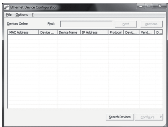
Ilustracja 5.2 Uruchamianie narzędzia
