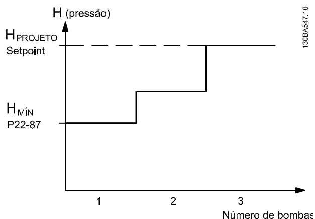
Ilustração 3.56 Número de Bombas
