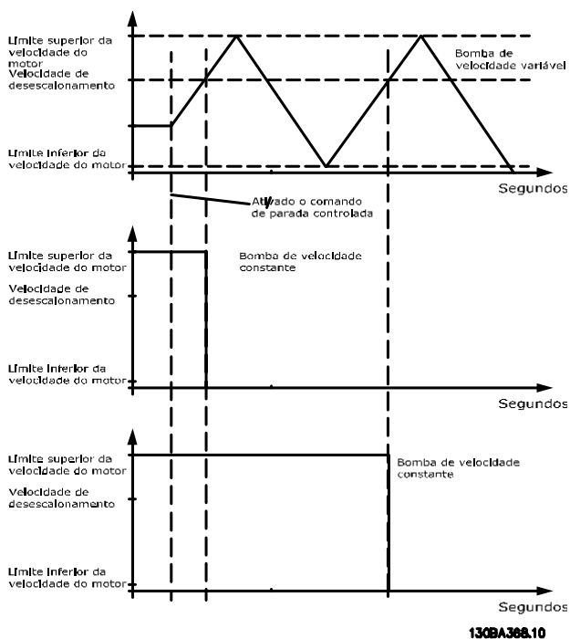
Ilustração 3.80 Velocidade de Desescalonamento
