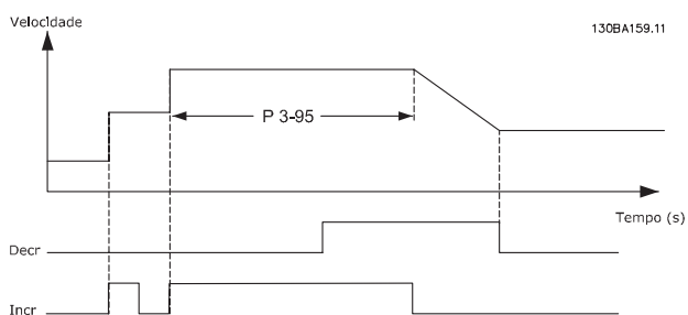
Ilustração 3.23 Atraso de Rampa Caso 2
