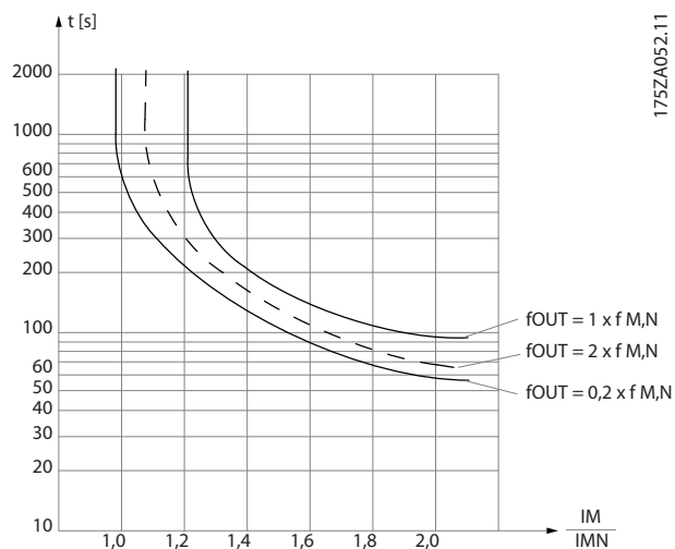
Ilustração 3.14 Perfil do ETR
