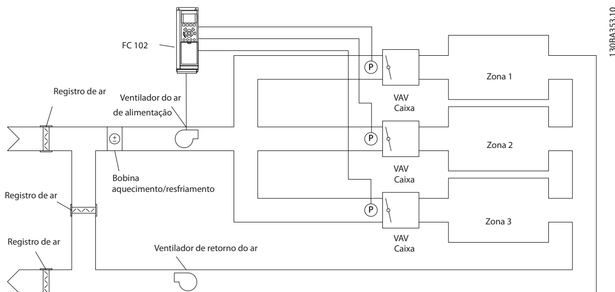
Ilustração 3.48 Exemplo, multizonas, setpoint único
