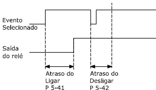
Ilustração 3.26 Atraso de desligamento, relé
