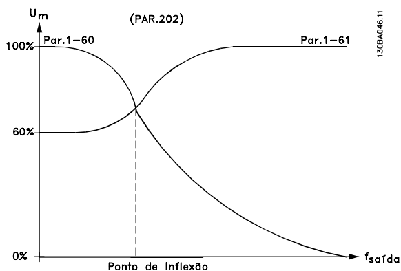
Ilustração 3.9 Compensação de Carga de Baixa Velocidade
