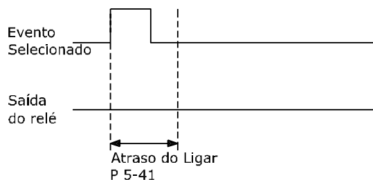
Ilustração 3.25 Atraso de Ativação do Relé
