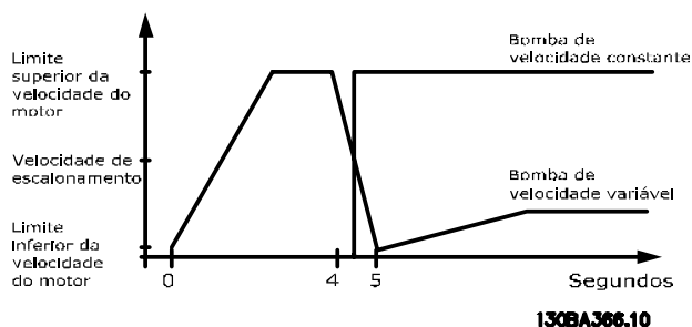
Ilustração 3.78 Limite de Escalonamento
