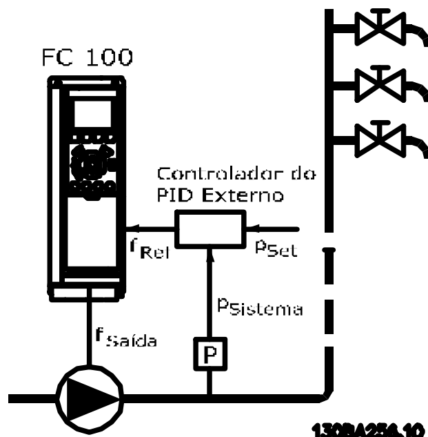
Ilustração 3.53 Sistema de impulso
