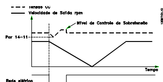
Ilustração 3.37 Desaceleração Controlada - Falha de Rede Elétrica de Curta Duração
