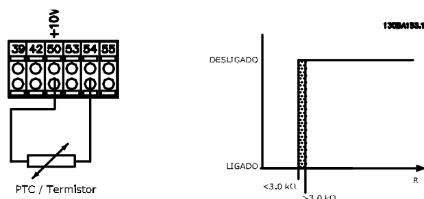
Ilustração 3.13 Conexão do termistor PTC - Entrada analógica
