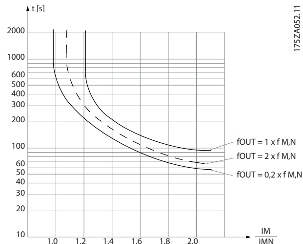
Ilustração 3.10 Proteção Térmica do Motor
