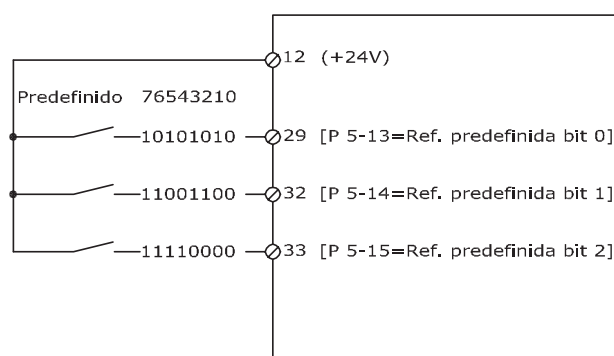
Ilustração 3.16 Esquema de Referência Predefinida
