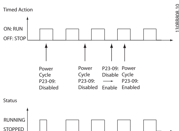
Ilustração 3.60 Diagrama de Teste de Reativação
