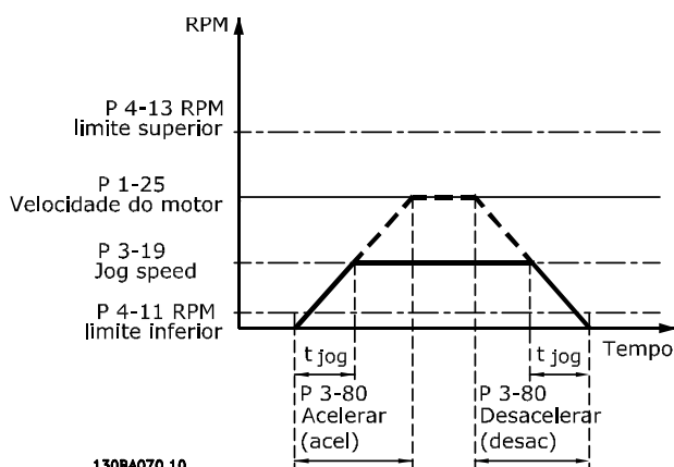
130BA070.10 Ilustração 3.21 Tempo de Rampa do Jog
