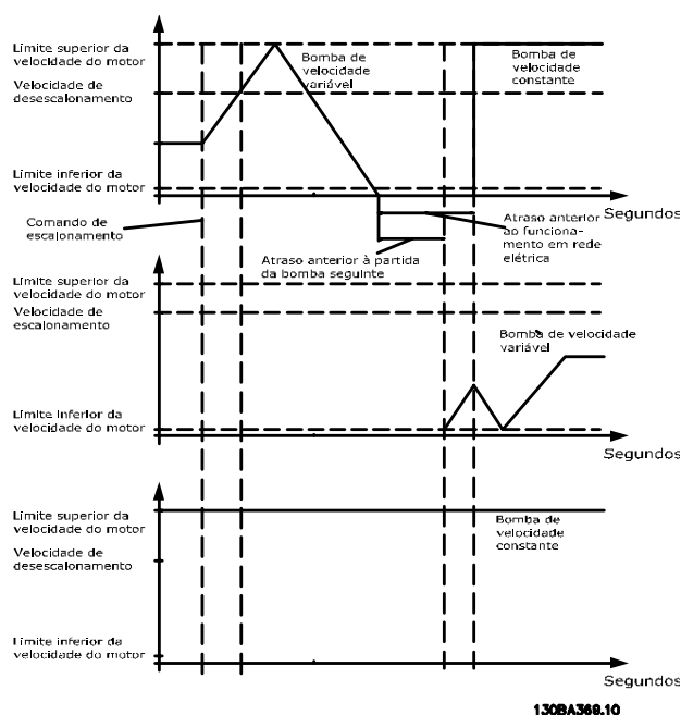
Ilustração 3.81 Modo Escalonamento em Alternação
