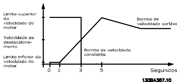
Ilustração 3.79 Limite de Desescalamento
