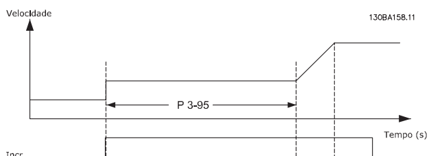
Ilustração 3.22 Atraso de Rampa Caso 1
