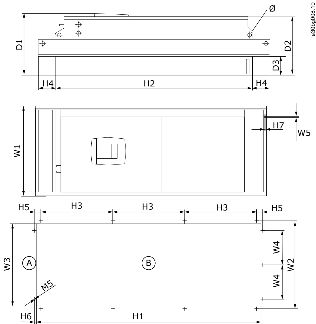
图解 68: VACON® NXS/NXP 交流变频器的尺寸, FR9
