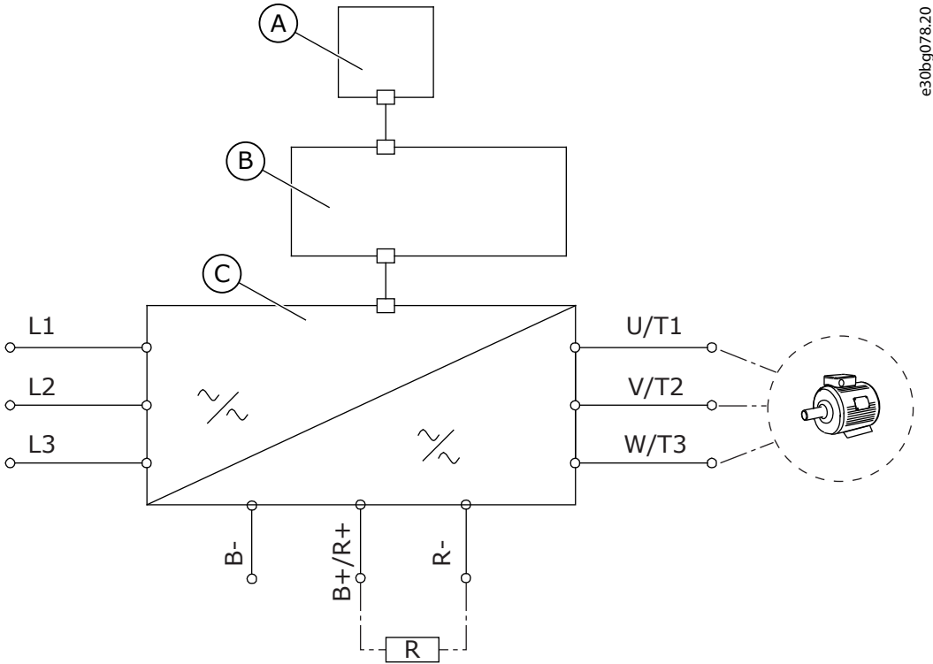
图解 13: 主要连接图
