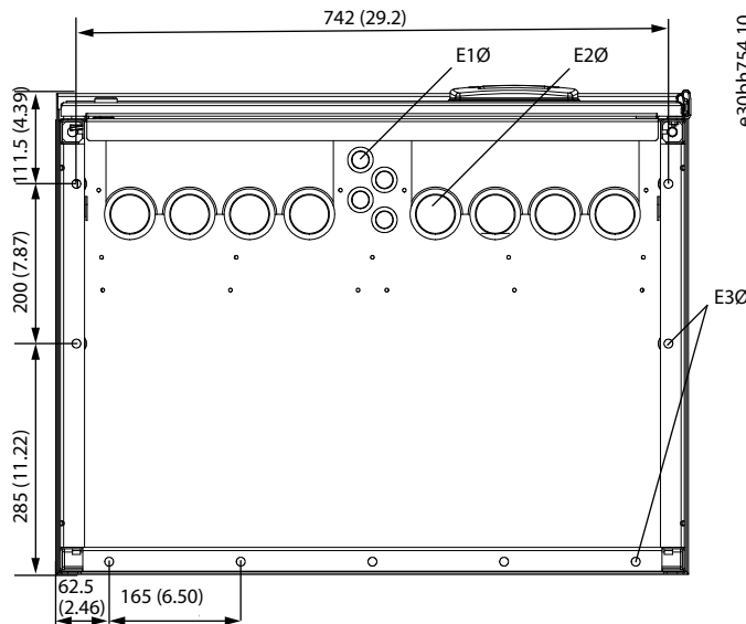
图解 72: VACON® NXS/NXP AC Drive 的安装孔尺寸, FR11 Standalone
