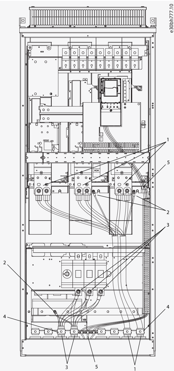
图解 34: FR11 Standalone, 0460 - 0502, 690 V
