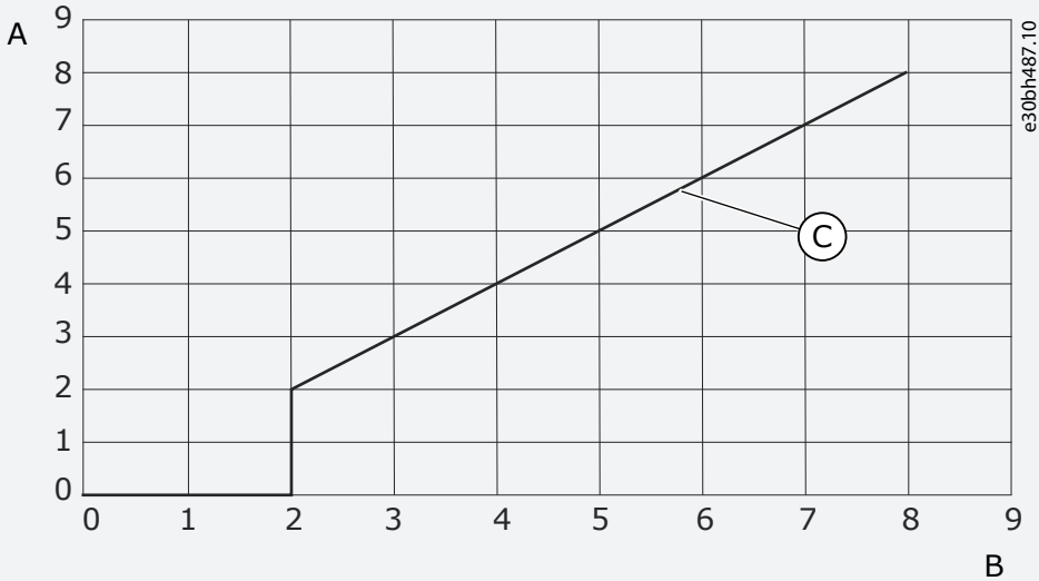
图解 52: 存储时间和重整时间
