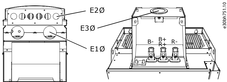
图解 59: VACON® NXS/NXP AC Drive 的安装孔尺寸, FR8
