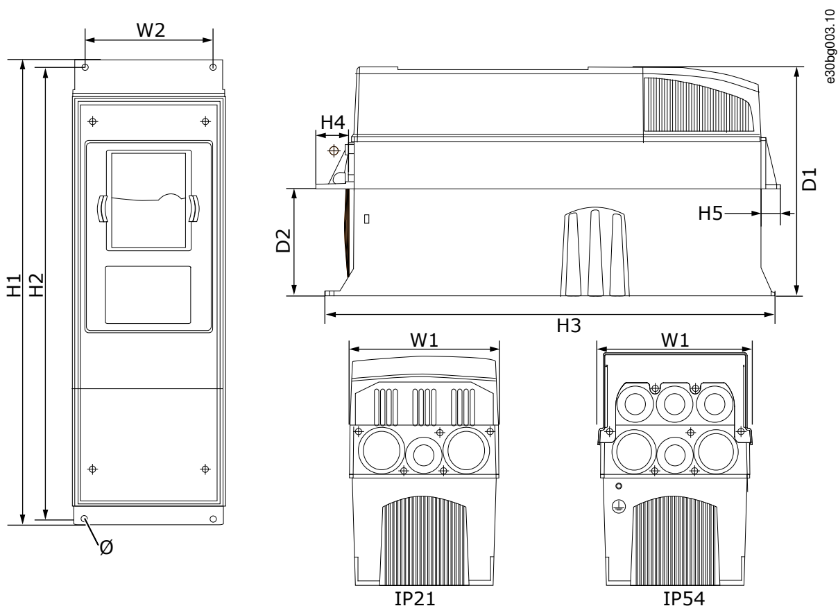
图解 63: 带法兰的 VACON ® NXS/NXP AC Drive 的尺寸, FR4 - FR6
