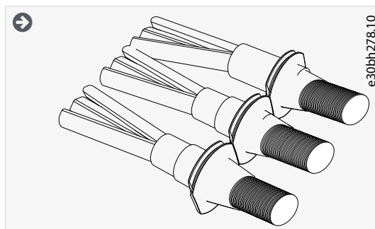
图解 29：在 IP54 防护等级下剪切索环
