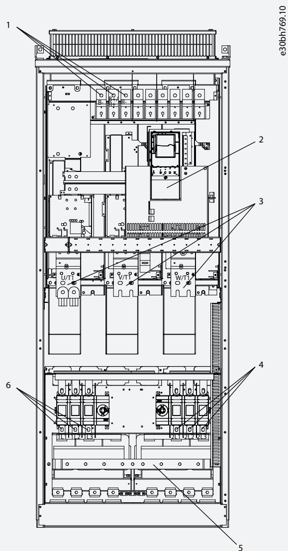
图解 23: FR11 Standalone 端子
