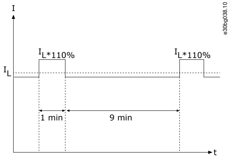
图解 74: 低过载
