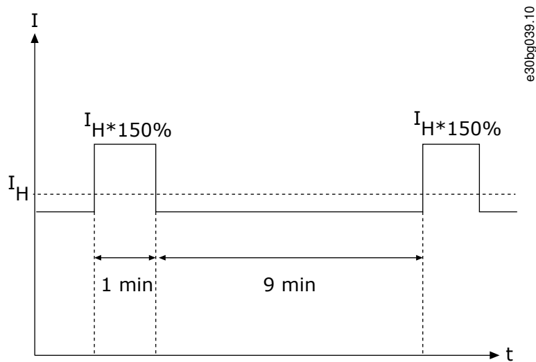
图解 75: 高过载
