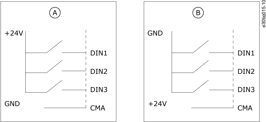
图解 42: 正/负逻辑
