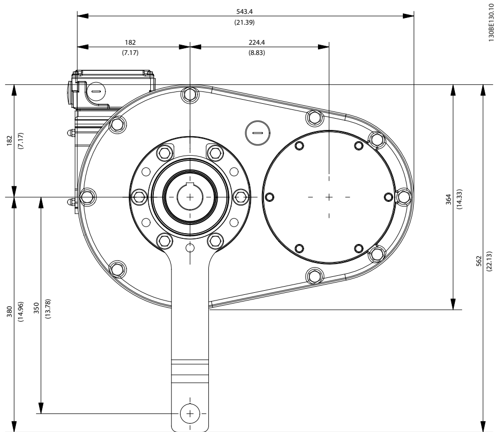
图 3.1 ExtensionBox 尺寸
