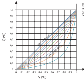
AV:4 / 32772 알파 값 곡선
