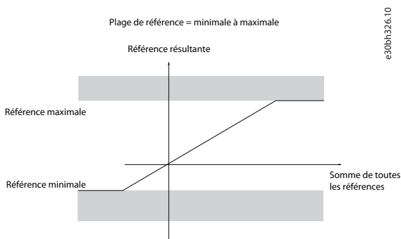
Illustration 44: Somme de toutes les références lorsque le mode de configuration est réglé sur Process
