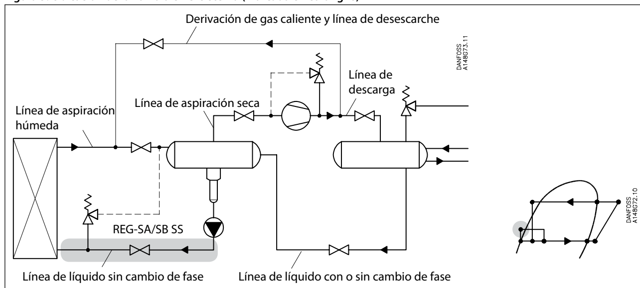
Figura 5: Ubicación de la válvula en el sistema (marcada en color gris)
