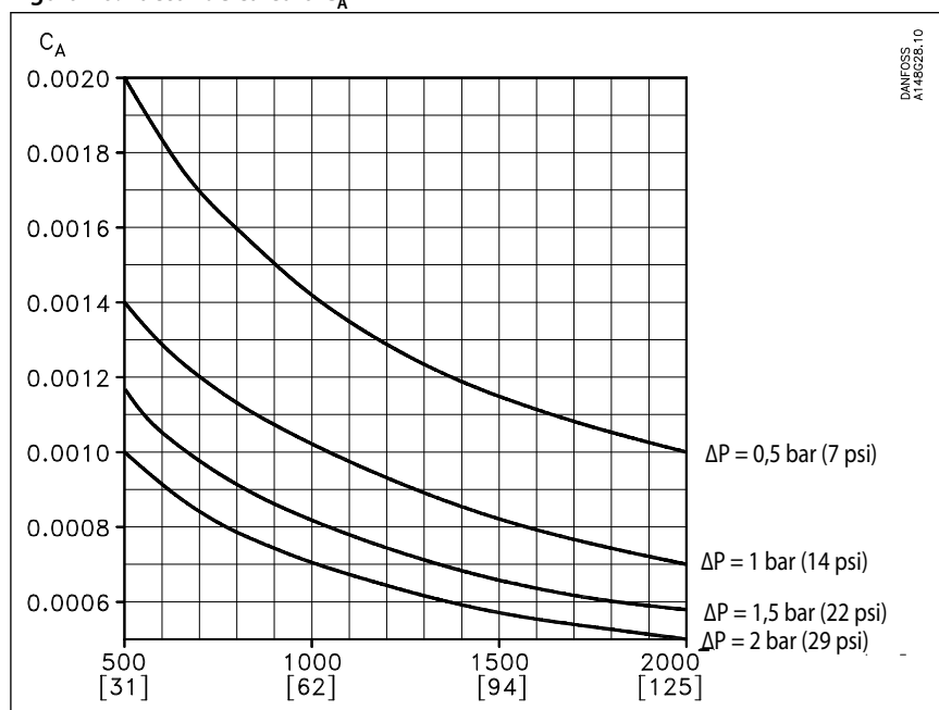
Figura 10: Factor de cálculo C_A
