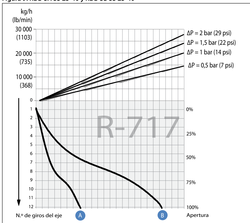
Figura 9: REG-SA SS 25-40 y REG-SB SS 25-40
