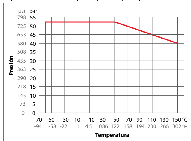
Figura 1: Gráfico de rangos de presión y temperatura
