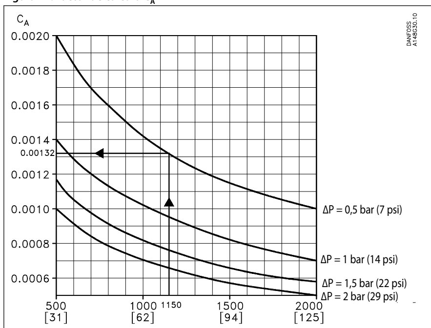
Figura 13: Diagrama de caudal
