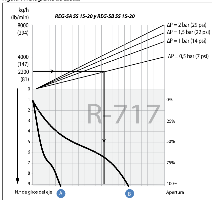
Figura 11: Diagrama de caudal
