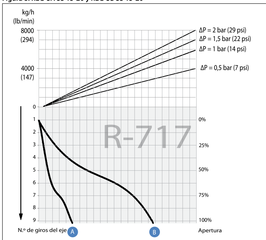
Figura 8: REG-SA SS 15-20 y REG-SB SS 15-20
