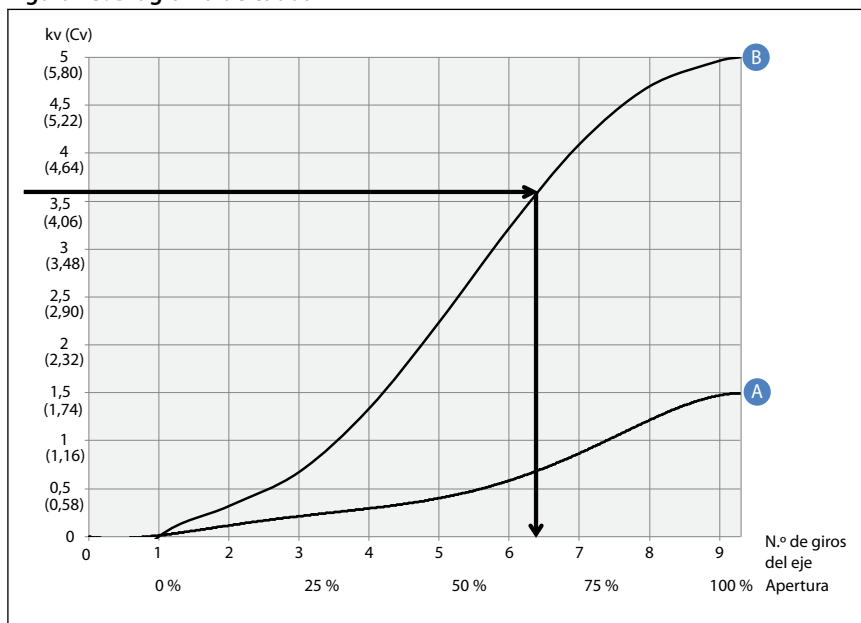
Figura 13: Diagrama de caudal
