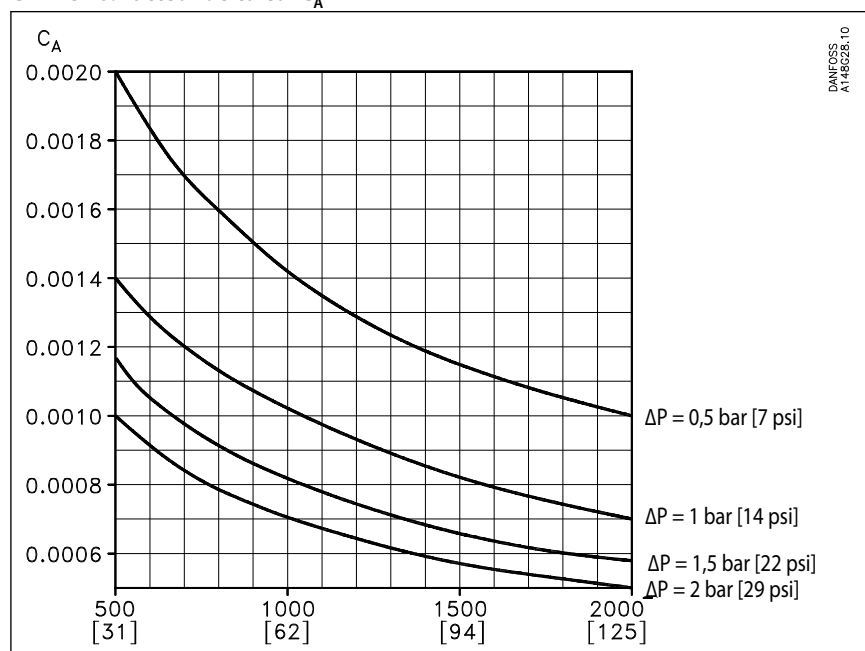
Chiffre 10: Facteur de calcul C_A
