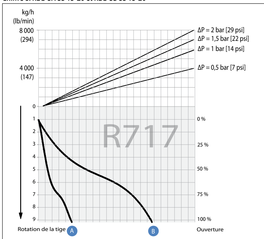
Chiffre 8: REG-SA SS 15-20 et REG-SB SS 15-20
