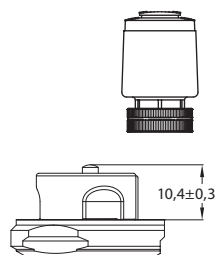
Uždarymo taškas (matavimas), skirtas DN 15-32
