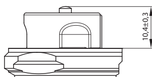
Point de fermeture (mesure) pour DN 15-32
