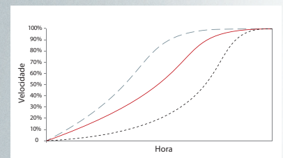
Três perfis de partida com Controle de Aceleração Adaptativo (AAC); aceleração antecipada, constante e tardia
