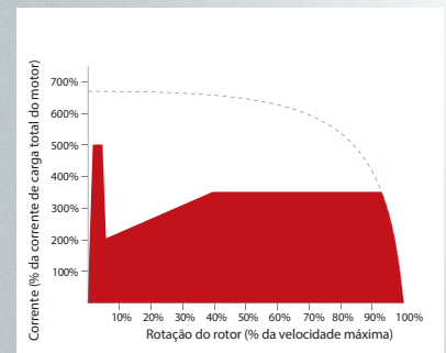
Corrente constante/rampa de corrente – mostrada aqui com arranque
