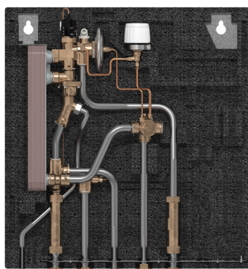
EvoFlat WSS , avec circulation
