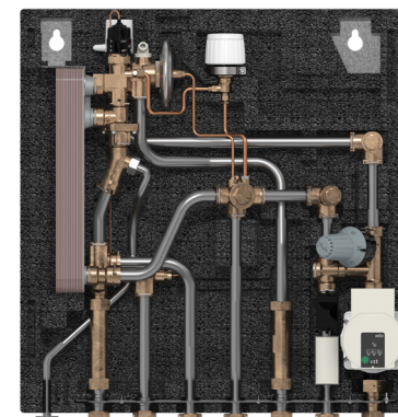
EvoFlat MSS, avec circulation
