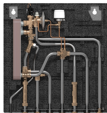
EvoFlat FSS, avec circulation
