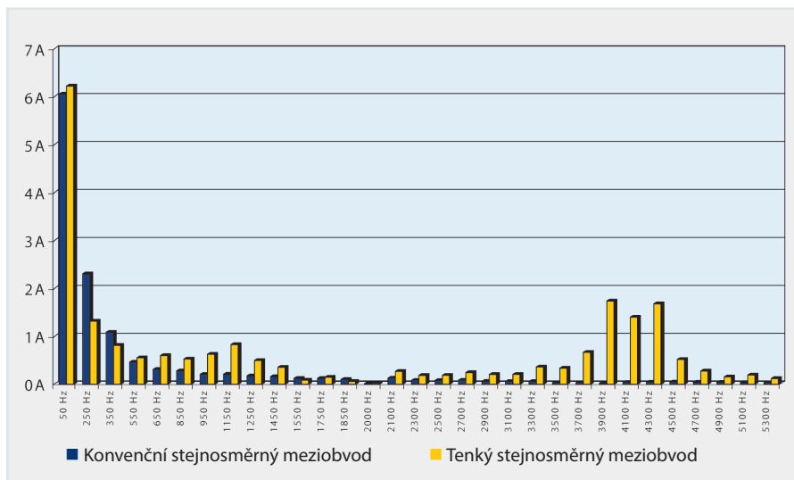
Měníče s tenkými stejnosměrnými meziobvody generují vyšší úroveň harmonických, zvláště ve vyšších rozsazích kmitočtů.
