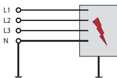
TT síť Samostatný vodič pro uzemnění a individuální uzemnění komponent
