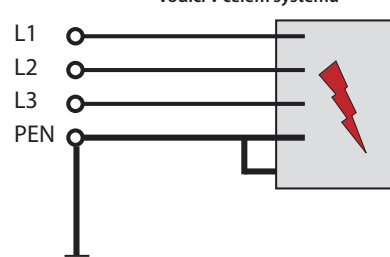
TN-C síť Kombinace nulového N vodiče a ochranného PE vodiče ve společném vodiči v celém systému
