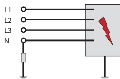
IT síť Izolovaný systém, kde nejsou komponenty uzemněny ani uzemněny s impedancí.
