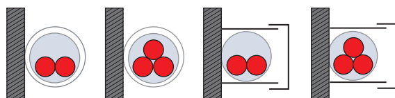
Metoda Instalacji B2: Przewód wielożyłowy, bądź przewód wielożyłowy osłonięty kanałem kablowym, albo zamknięty w korytkach
