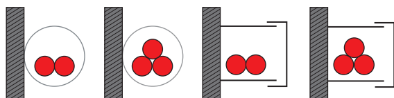
Metoda instalacji B1: Żyły przewoźne w kanałach kablowych, bądź zamknięte w korytkach.
