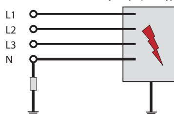
Układ zas. typu IT
