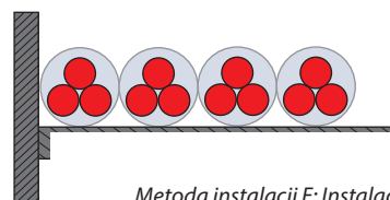
Metoda instalacji E: Instalacja na świeżym powietrzu, bądź w drabinkach kablowych.
