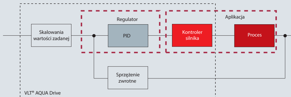
Schemat blokowy sterowania procesu PID
