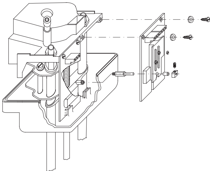
Концевой выключатель (2 контакта)
