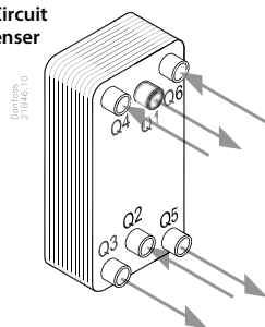
Evaporator
