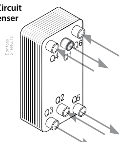
Evaporator
