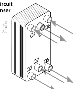
Evaporator
