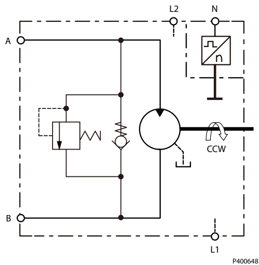
开式回路
