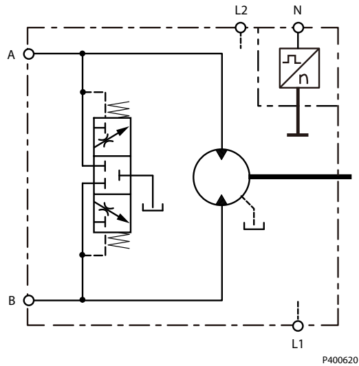
闭式回路
